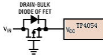
图 6：低损耗输入反向极性保护
