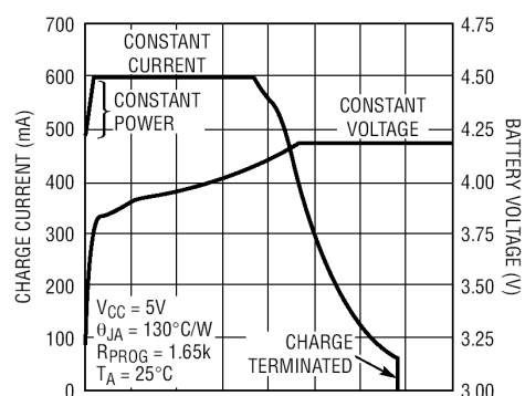
完整的充电循环 (750mAh 电池)
