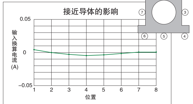
线径10mm，DC 100A输入
