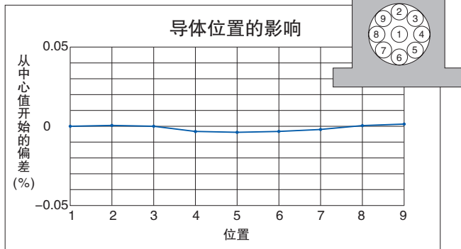
内径40mm，线径10mm，DC 100A输入
