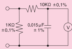
滤波器 ON
