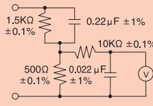
滤波器1 ON
