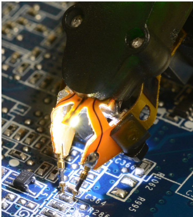
P77BRWSR 浏览器上的照明灯增强了查看探测点的能力
