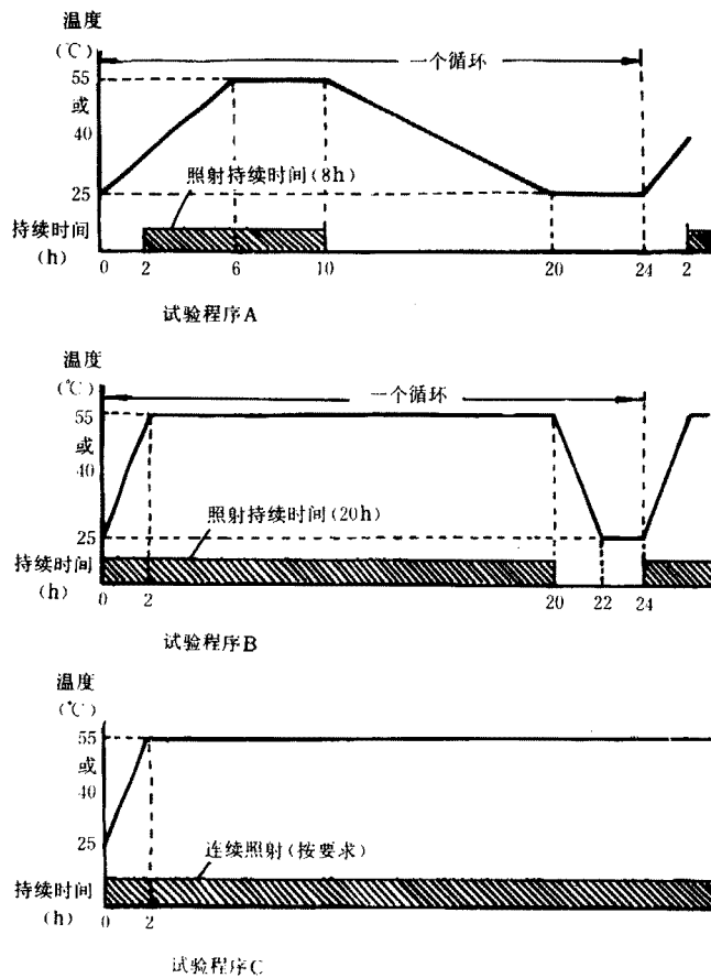
图1 温度-辐照-时间关系图
