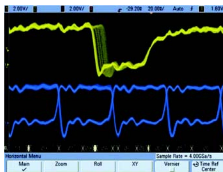
改进示波器显示质量
