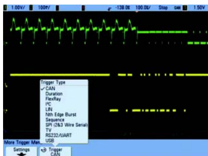
触发和解码 CAN 包
