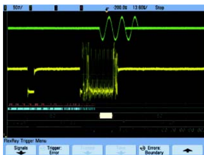
用 MSO 在 FlexRay 系统中进行混合信号测量
