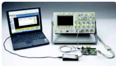
用 FPGA 动态探头和 Agilent MSO 更快和更有效地调试和验证您的 FPGA 设计
