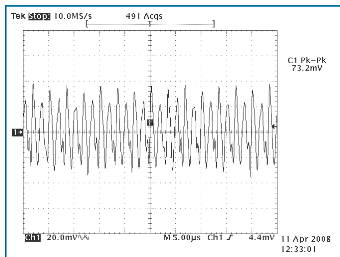
PST26 output noise V1 24V
