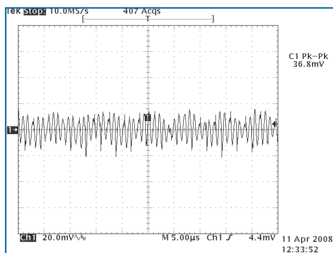
Output noise V2, V3 +/- 15V
