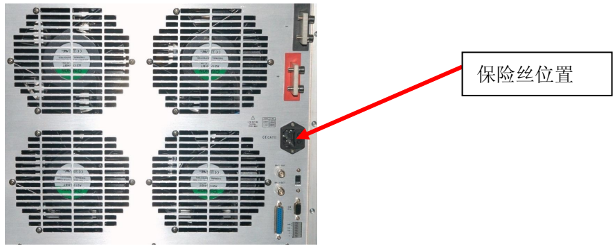
图3.1 保险丝位置
