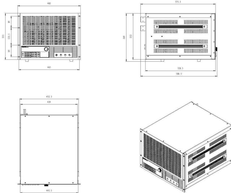
8U 仪器外形结构示意图
