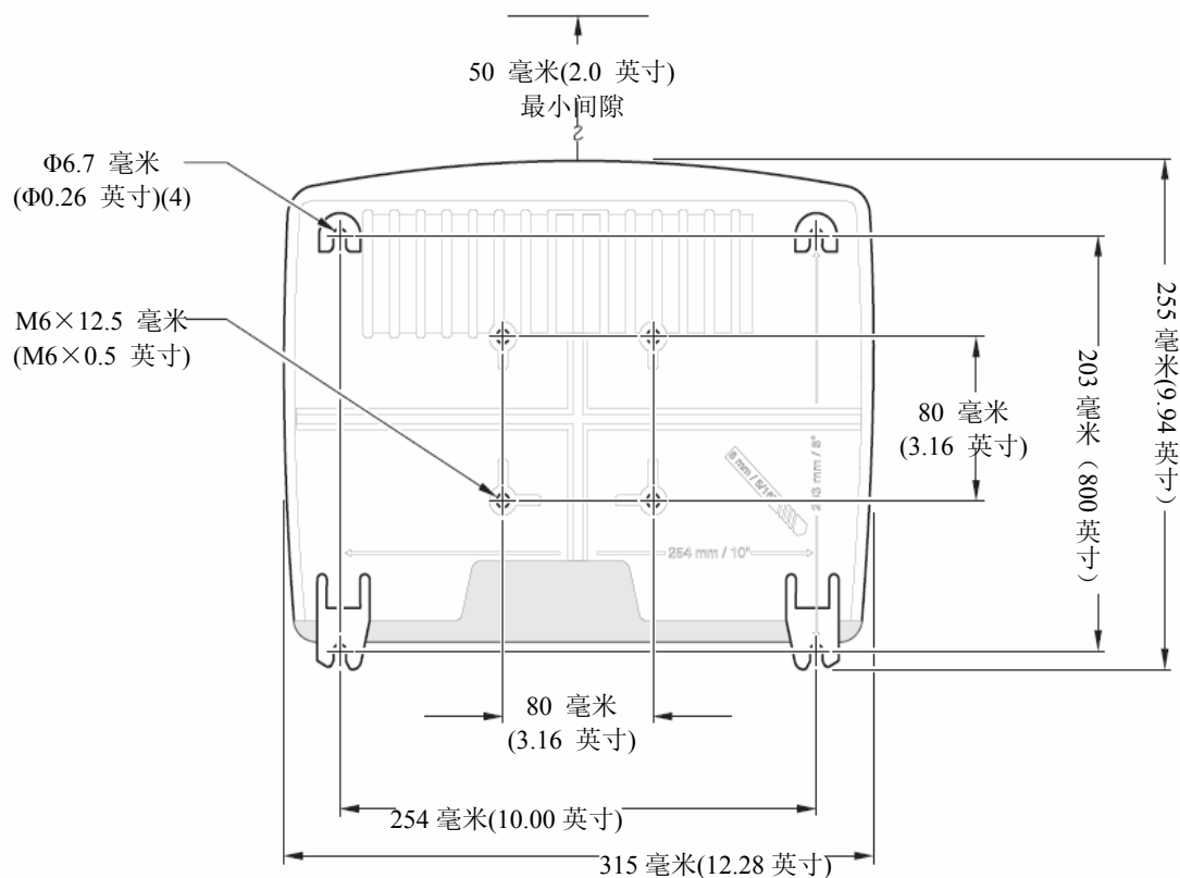
图 3 sc1000 控制器安装参数
