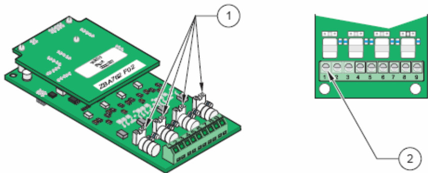
图 23 输入卡电缆线路和跳接设置
