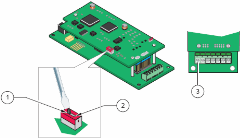
图 26 Profibus DP 卡线路
