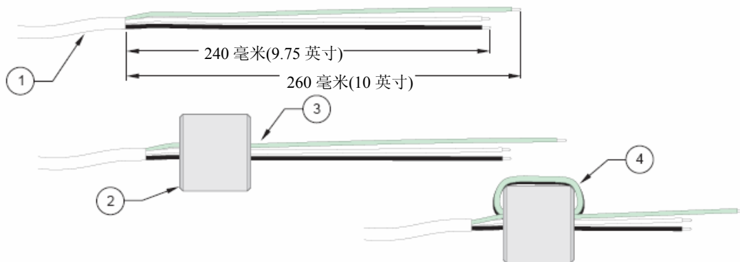
图 12 正确的接线准备和铁氧体磁心配线
