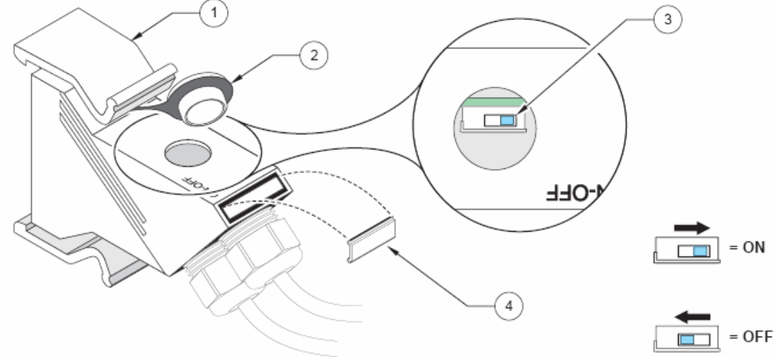
图 30 设置终端电阻器（连接器的 DIP 开关）
