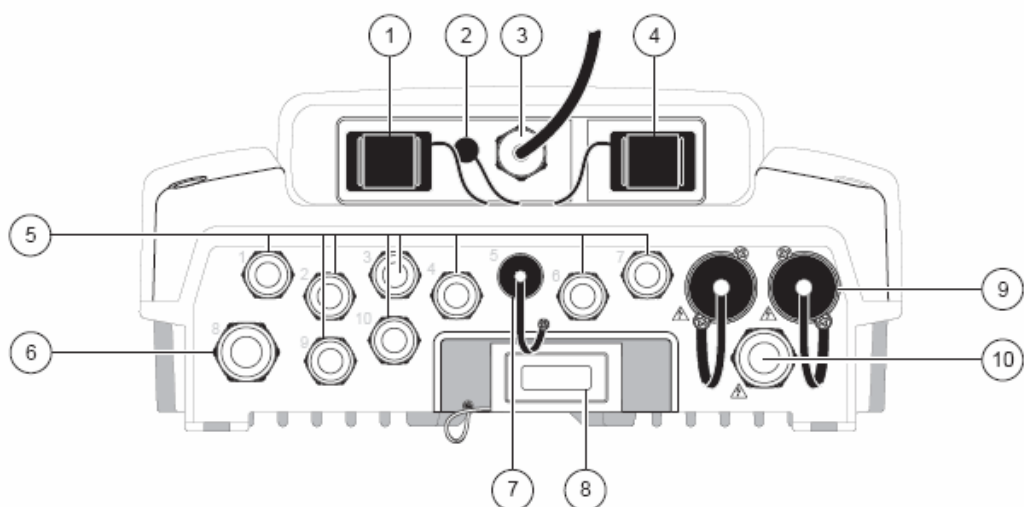
图 8 机架分线
