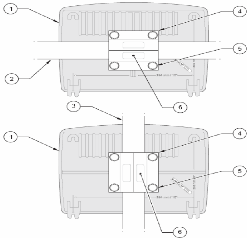
图 5 管道安装 sc1000 控制器
