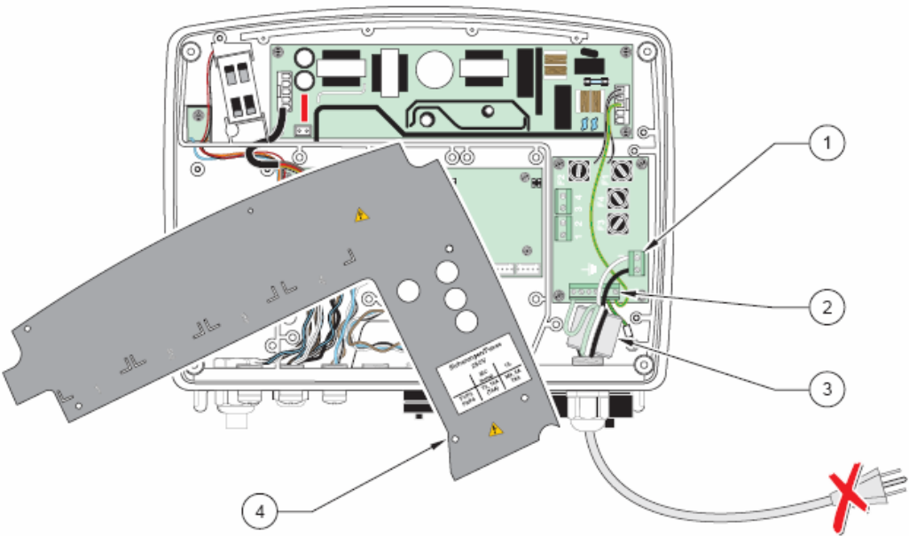
图 14 电源配线
