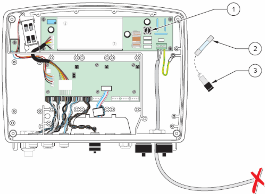
图 46 更换保险丝（24 伏直流电源）
