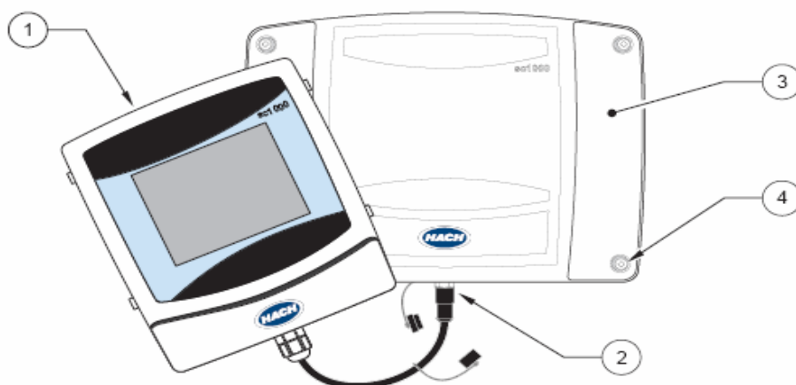
图 6 拆去显示器与探头外壳
