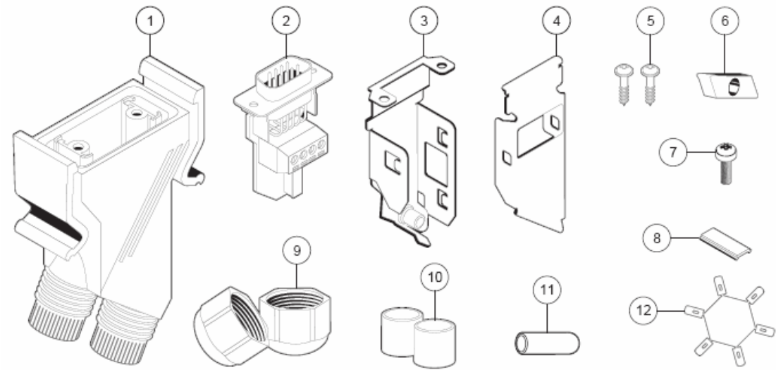
图 28 网络连接器组件
