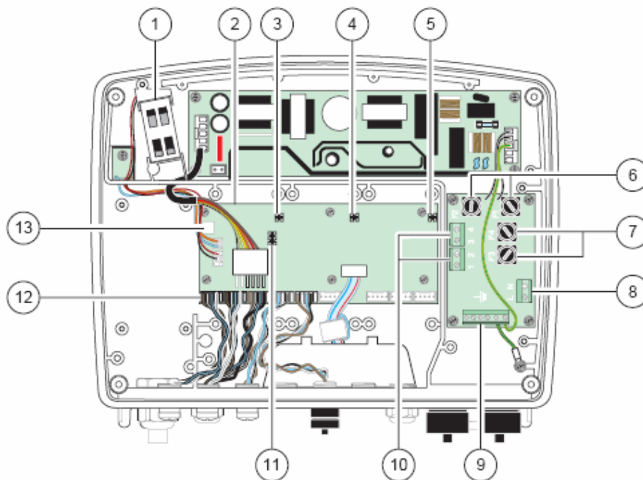
图 15 交流电源探头内部组成
