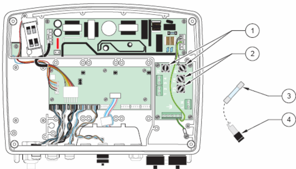
图 45 更换保险丝（交流电源）
