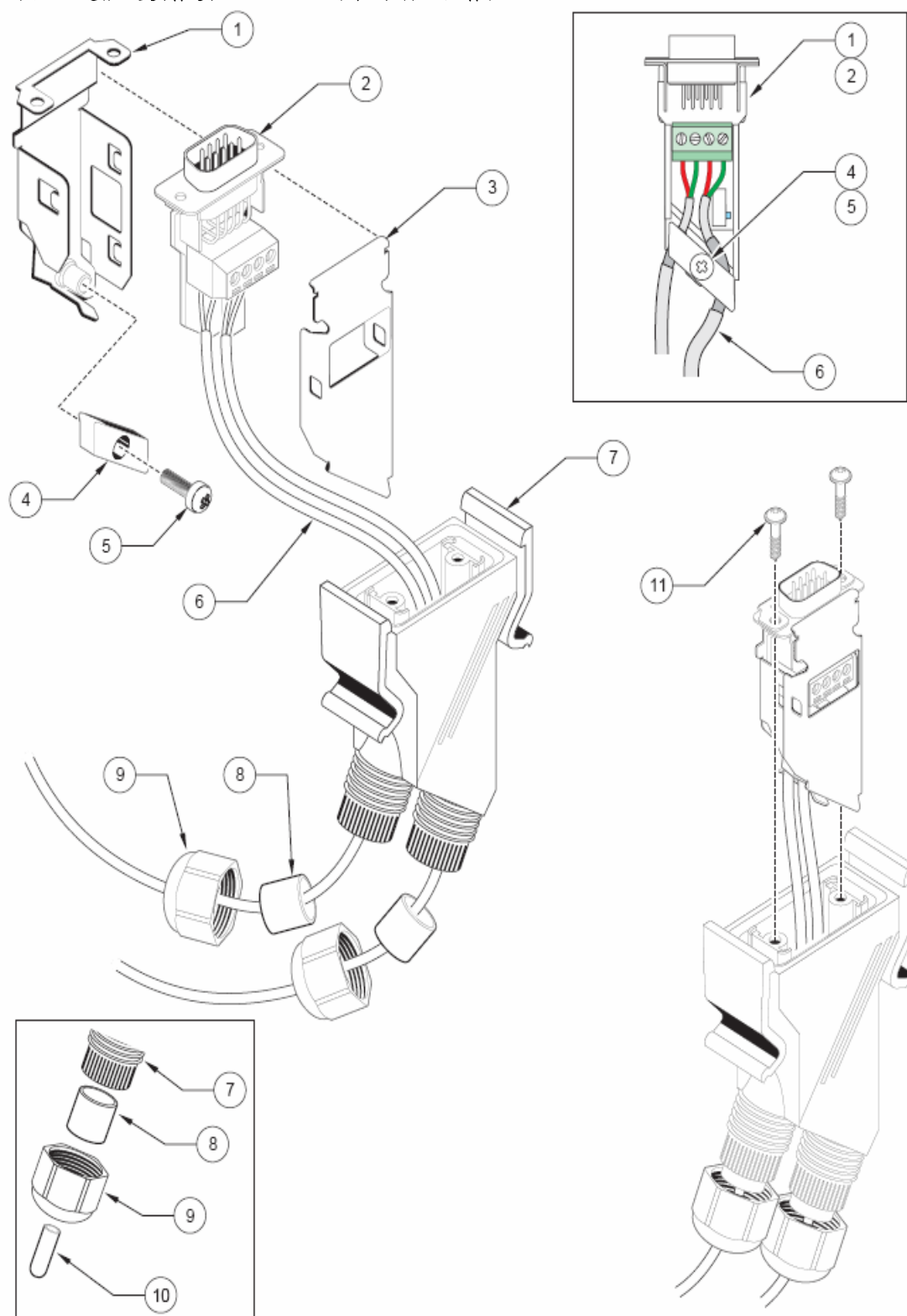
图 29 通信连接器接入 sc1000 网络终端电阻器方法
