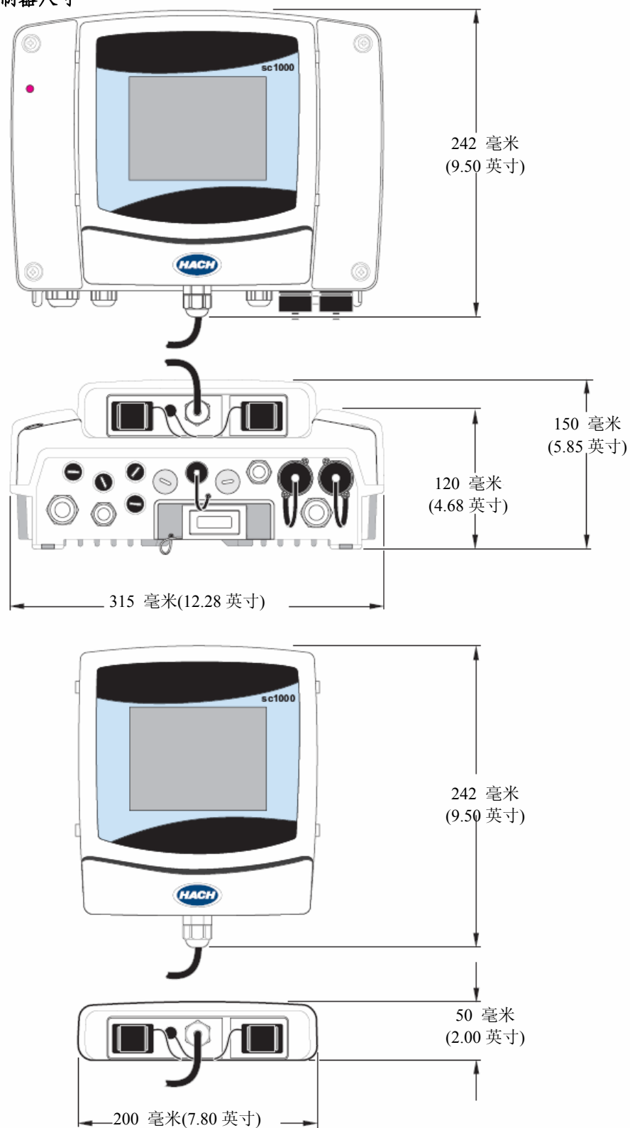
图 2 sc1000 控制器尺寸
