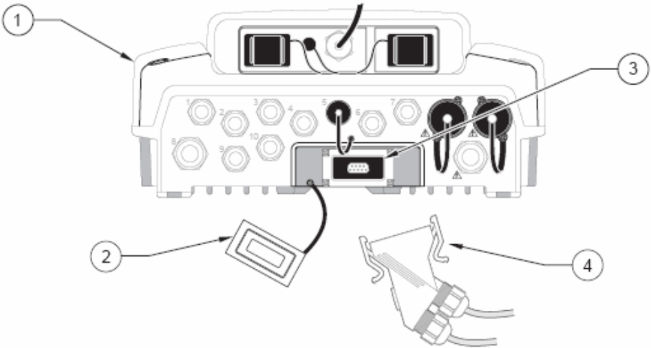
图 31 网络连接器插入网络接口
