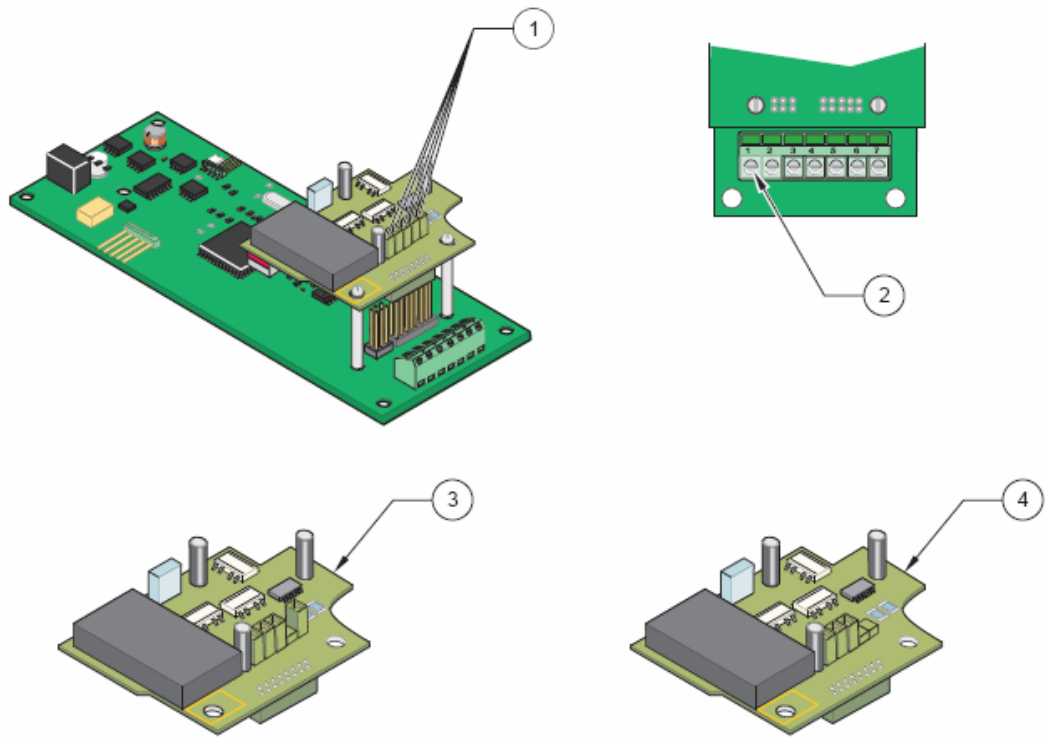
图 25 Modbus 卡线路
