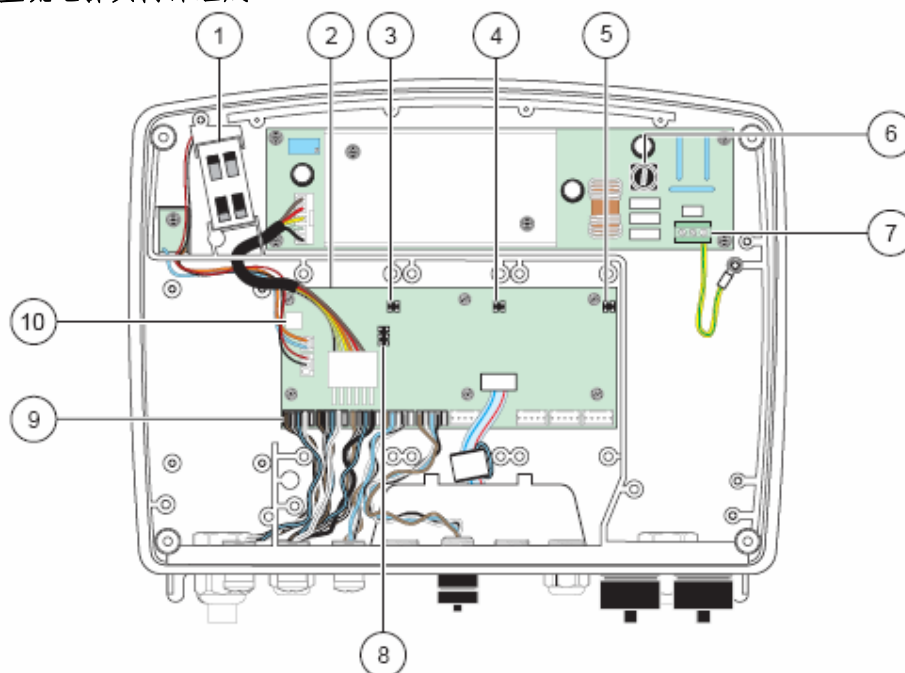
图 17 24 伏直流电探头内部组成
