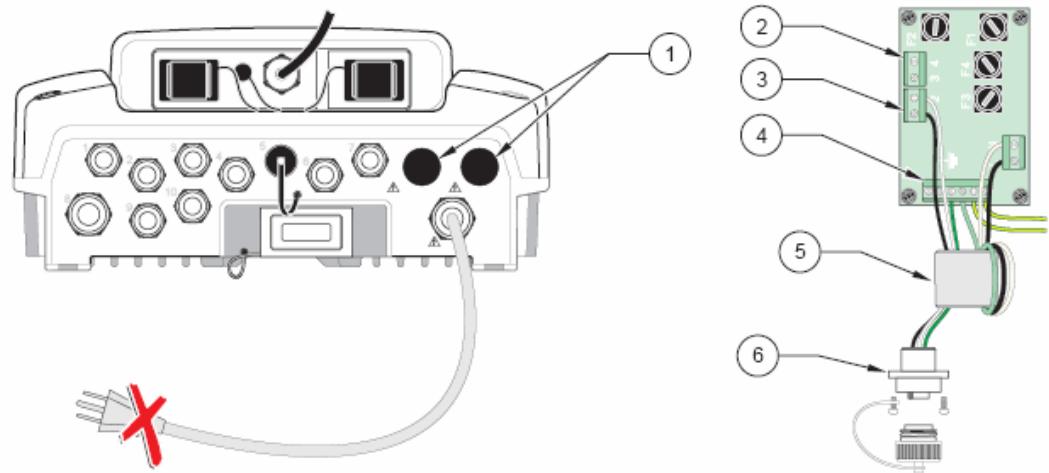
图 16 安装交流电输出端
