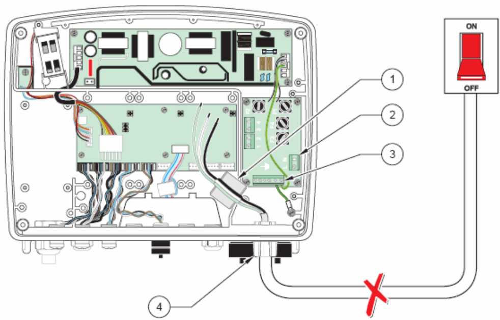
图 10 硬接线布局切断电源
