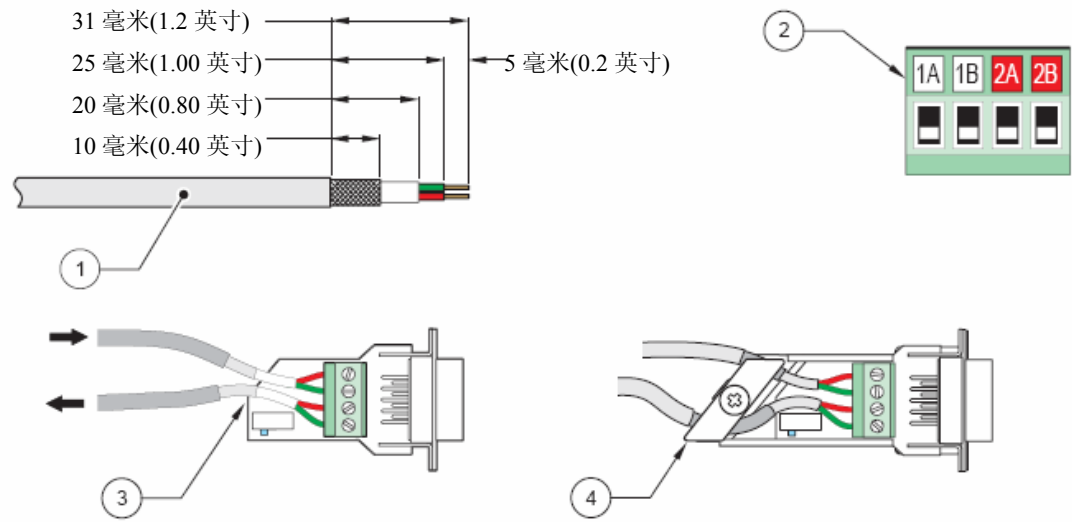
图 27 拆除通信电缆上的绝缘层
