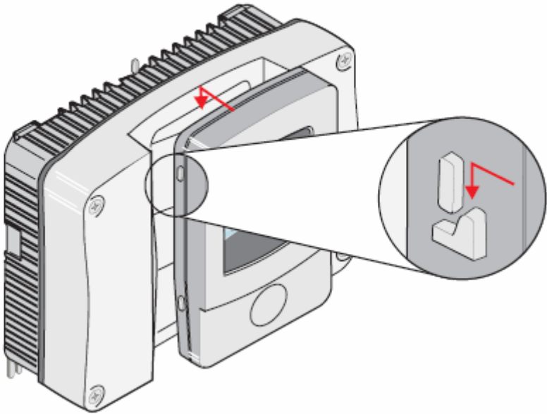
图 34 在探头单元上安装显示器
