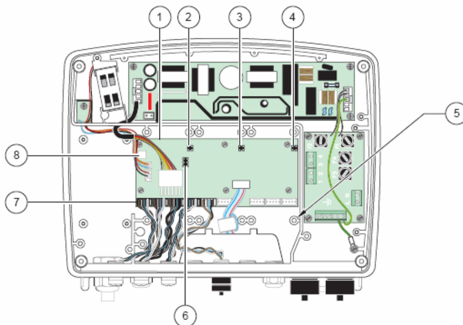
图 19 扩展卡主电路板接线
