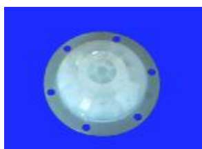
型号: 8605-2 焦距: 15 角度: 360° 距离: 5m 规格: \Phi 44.5
