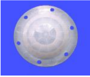
型号: 8603-4 焦距: 17.50 角度: 360° 距离: 5m 尺寸: \Phi 45.6
