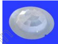
型号: 8604 焦距: 18 角度: 360^\circ 距离: 6m 外径: \Phi 51 内径: \Phi 35.5
