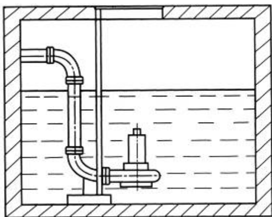
固定式安装
