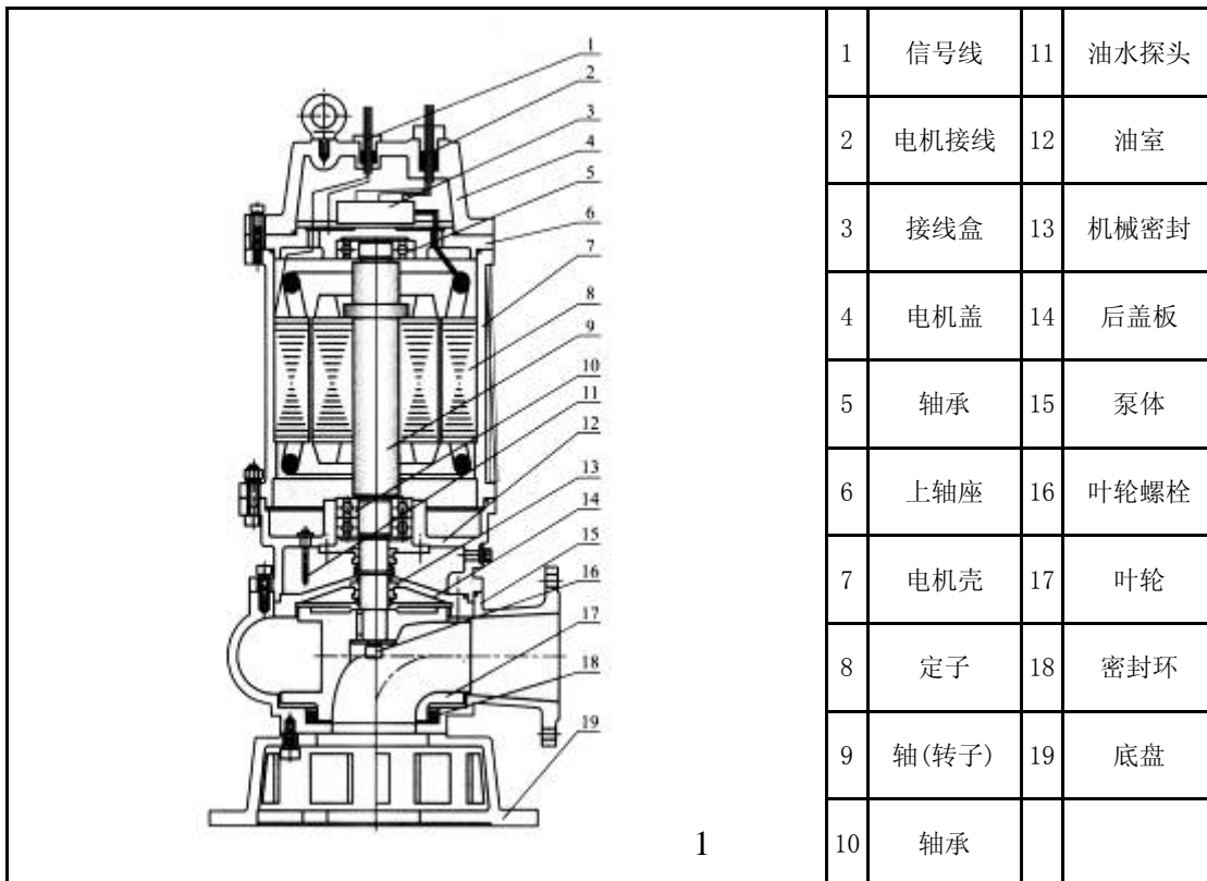
WQ 无堵塞潜水排污泵
