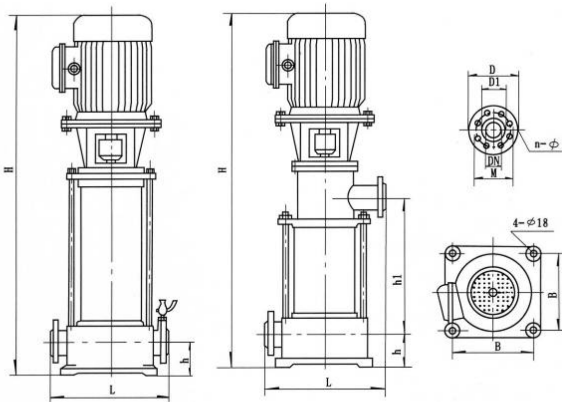
☆外型图及尺寸
