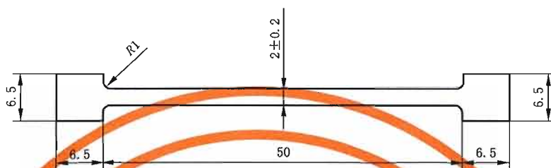
图 3 窄试样
