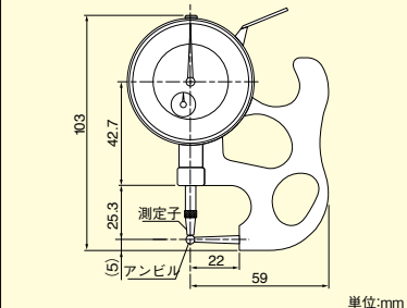
寸法図：TPM-116
