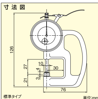
SM-528 厚さ20mmまでのワークが 測定できる小形シックネス 目量0.01mm 測定範囲20mm ・測定子、アンビル＝セラミック製
