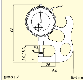
寸法図
