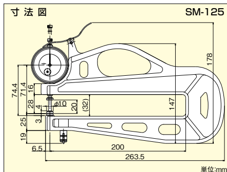
寸法図
