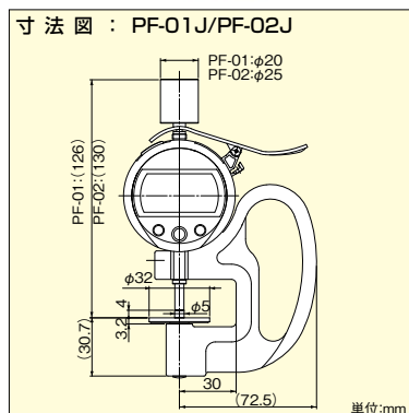
寸法図：PF-01J/PF-02J
