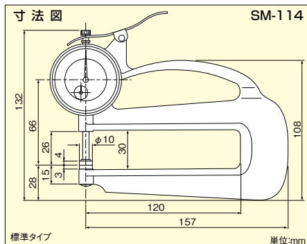
寸法図
