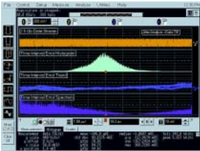
执行抖动分析
