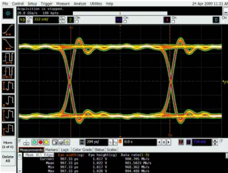
高达 4 GHz 的带宽和 20 GSa/s 的高采样率，可确保您能够看到被测信号的模拟特征的精确表征
