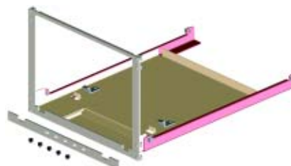
使用选件 1CM, 将 9000 系列示波器安装到 8U 高、19 英寸 (487 毫米) 宽的机架中。
