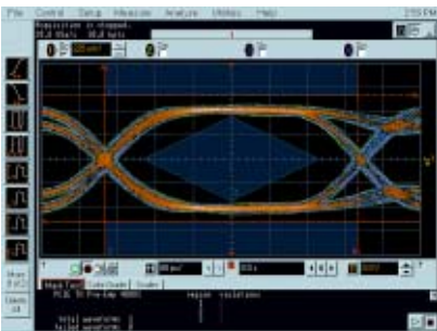
通过串行数据分析软件 ( SDA ) 恢复嵌入式时钟
