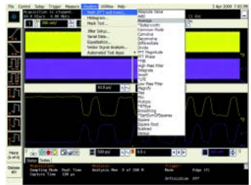
模板测试、直方图和大量的分析功能可对信号进行深入分析
