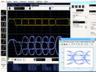
使用用户定义的函数进行信号均衡
