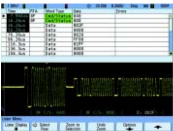
协议解码的 MIL-STD 1553 物理层信号的时间相关显示
