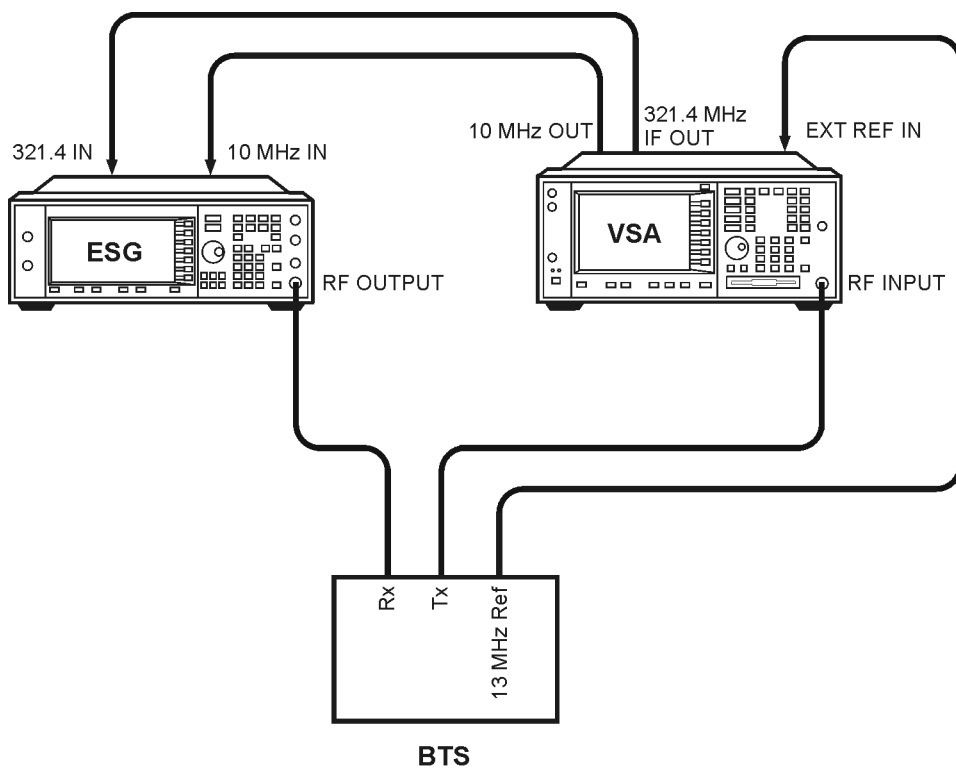
图 8-2 BTS 环回测试设备设置
