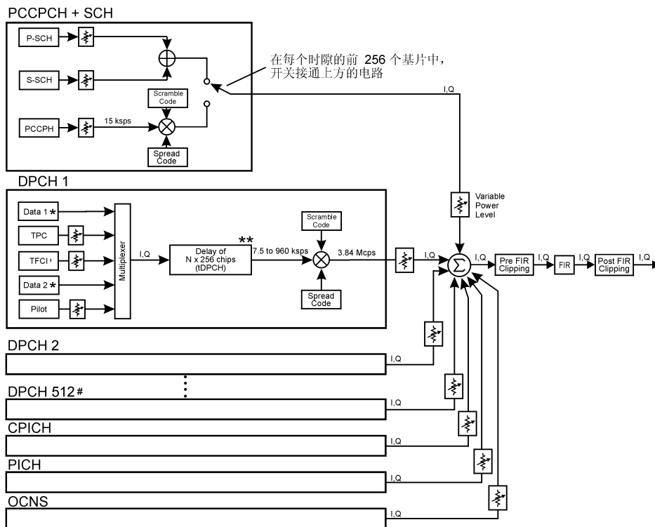
图 9-5 下行链路信道结构
