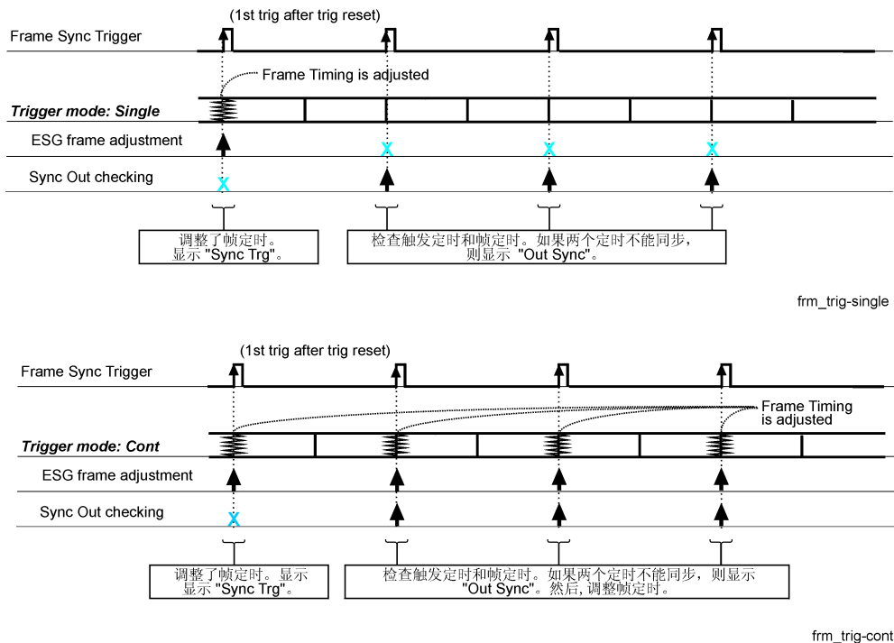
图 9-22 触发模式和同步
