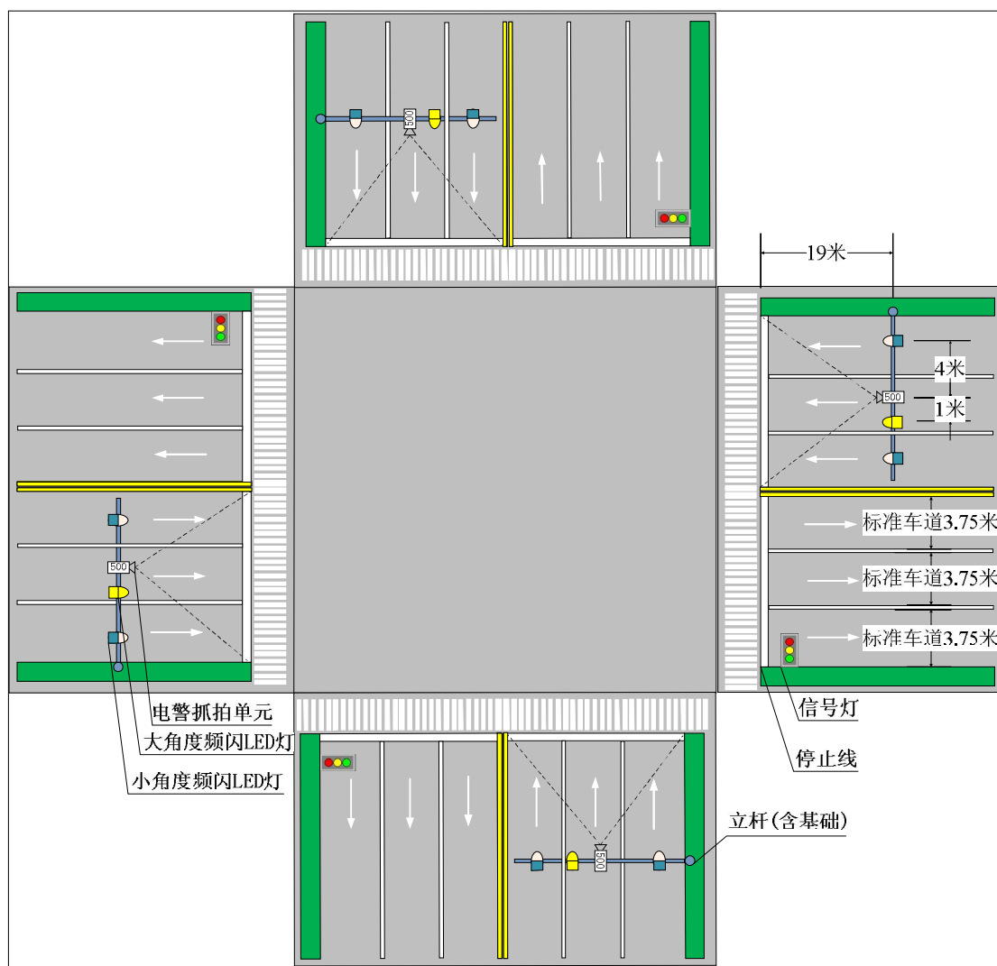
路口布局示意图
