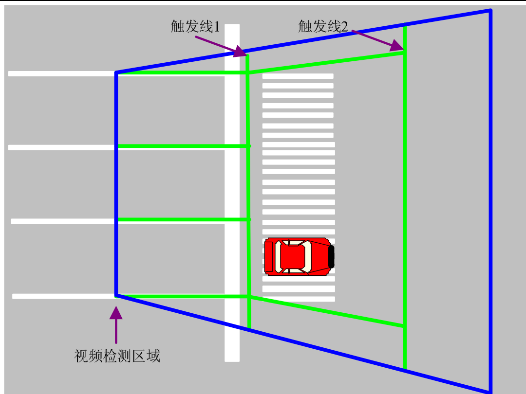
闯红灯车辆触发抓拍位置 2
