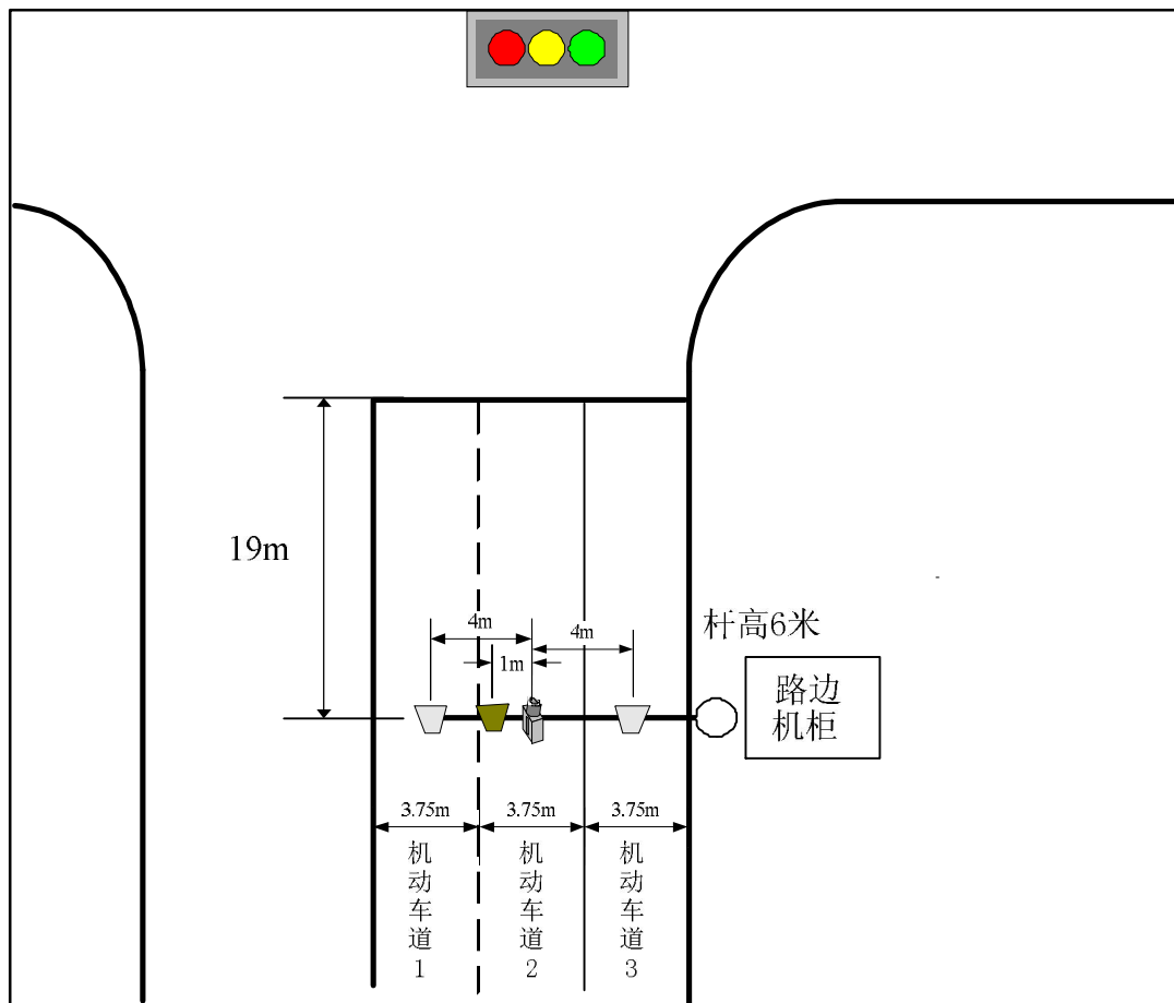
单向两车道 L杆安装示意图
