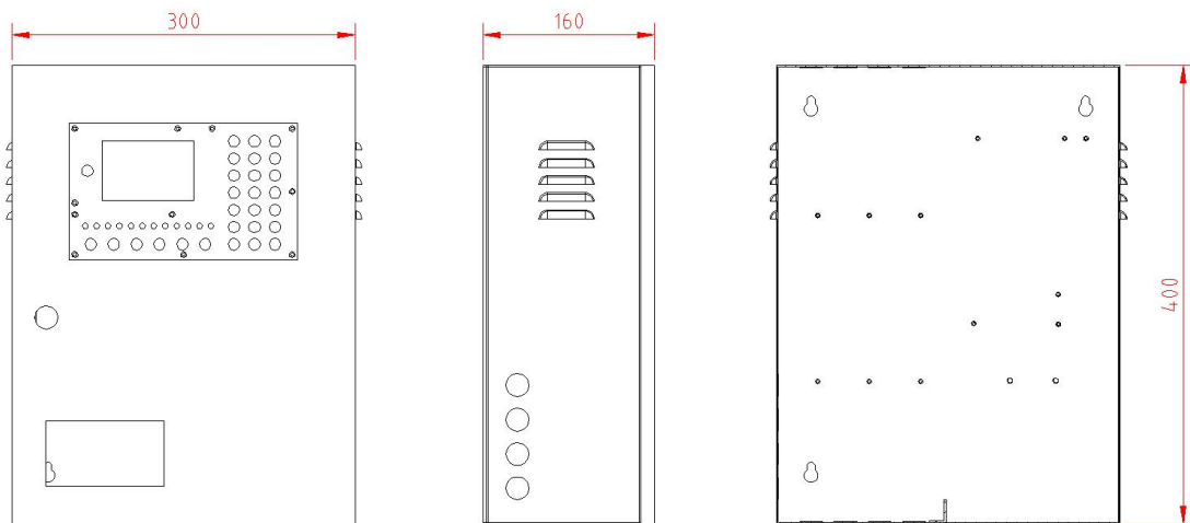
图 1 外形尺寸
