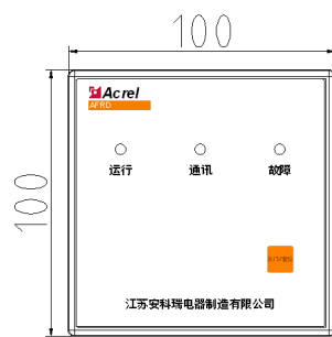
正面图
