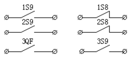
图 C.4 AM5-BL 二次接线原理图
