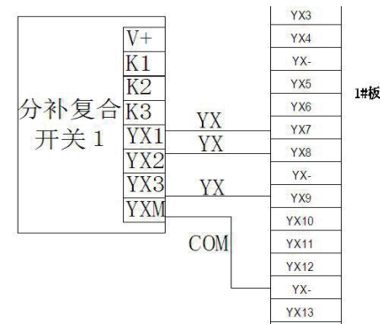
(6) YX10、YX11、YX12、YX13、YX14 分别接 1QF、2QF、3QF、4QF、5QF 断路器开关状态辅助接点。
