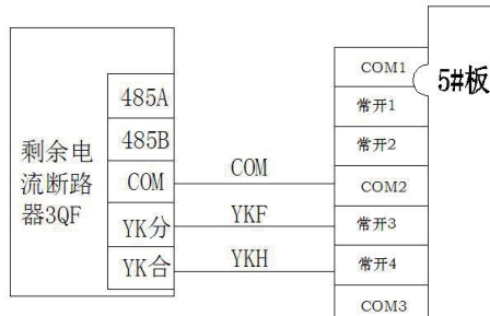
C、3QF 出线开关接线（剩余电流断路器）
