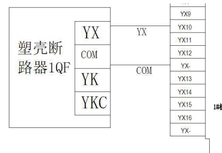
(6) YX10、YX11、YX12、YX13、YX14 分别接 1QF、2QF、3QF、4QF、5QF 断路器开关状态辅助接点。
