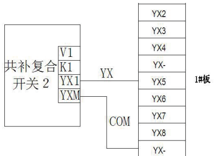
(3) YX5 接（共补复合开关 2）辅助接点。
