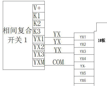
(2) YX4 接（共补复合开关 1）辅助接点。
