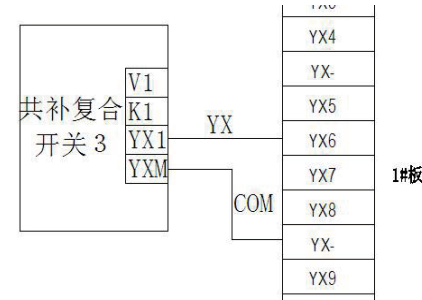
(5) YX7—YX9 接（分补复合开关 1）辅助接点。
