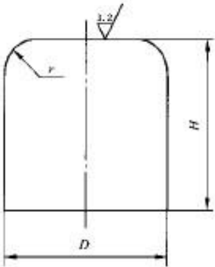
图 2 板状试样电极
