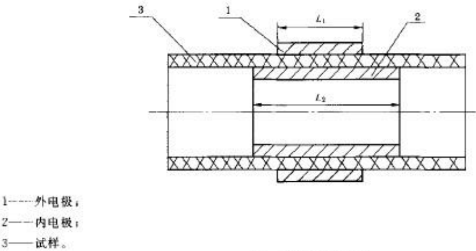
图 3 管状试样电极
