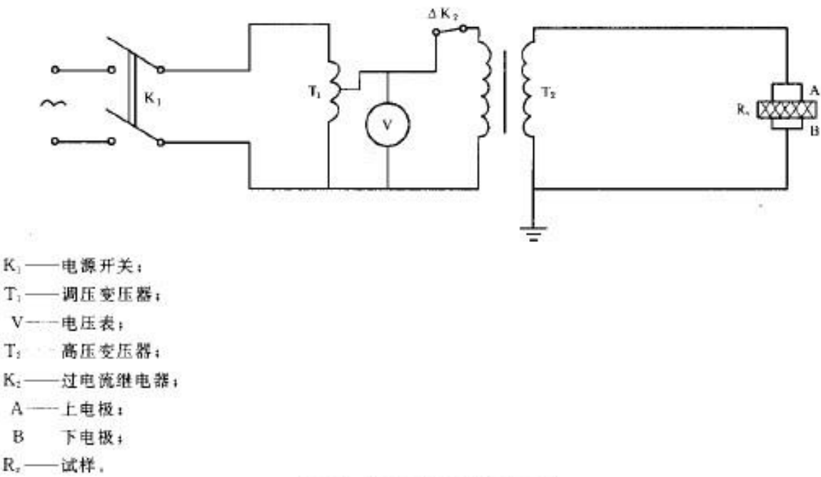
图 1 击穿电压测试原理图
