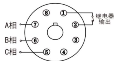
DX330 接线图
