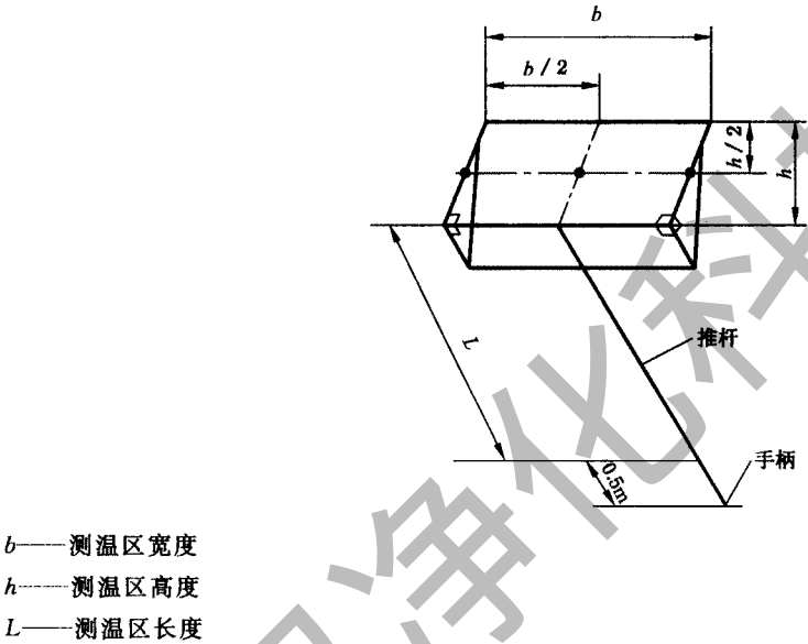
图 3 连续式电阻炉测温架(笆)和测温点位置图
