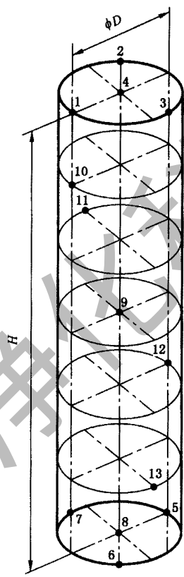
图 6 井式电阻炉工作区测温位置示意图
