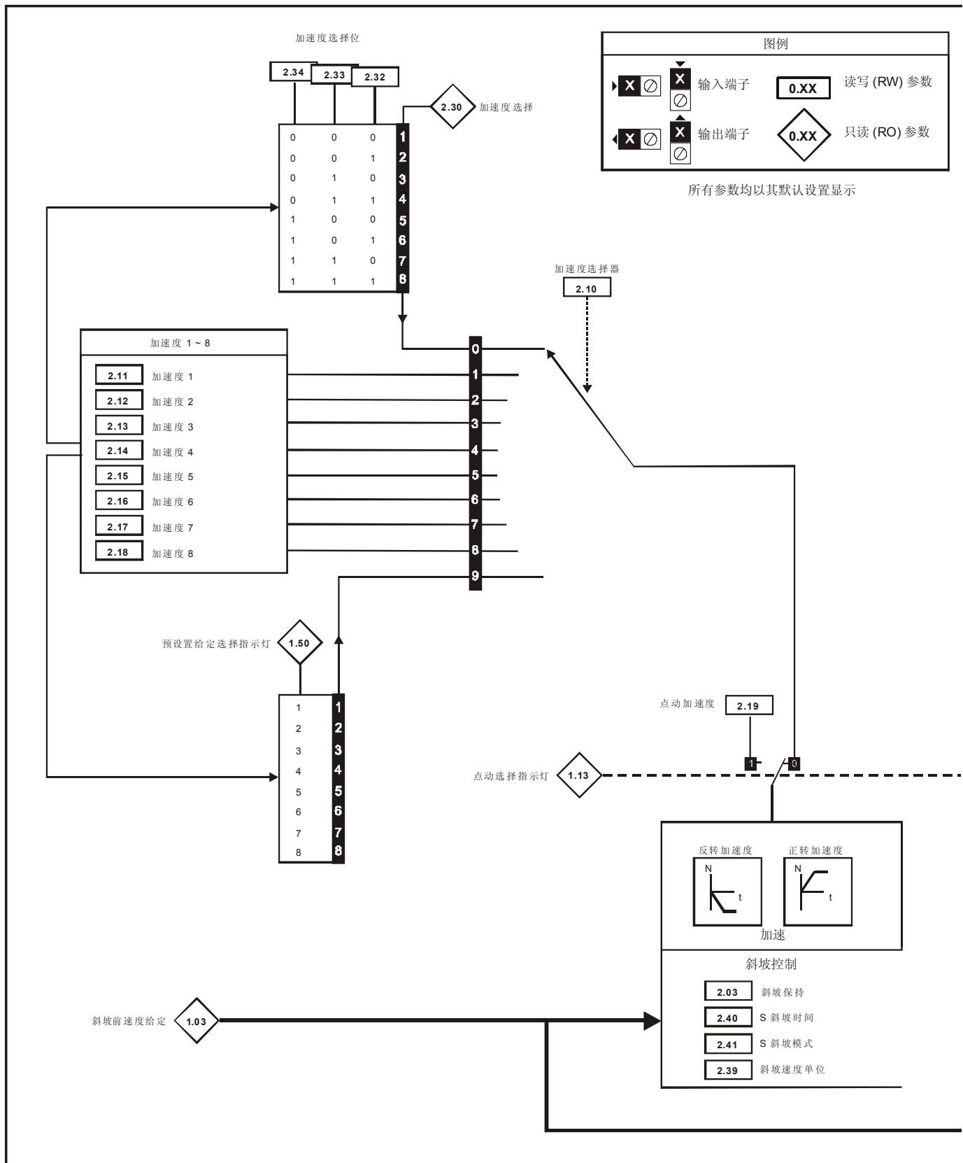
图 11-2 菜单 2 逻辑图
