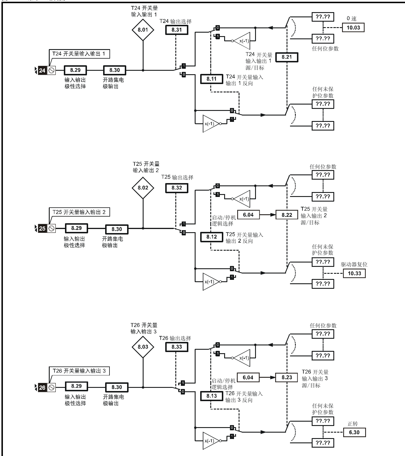
图 11-9 菜单 8 逻辑图
