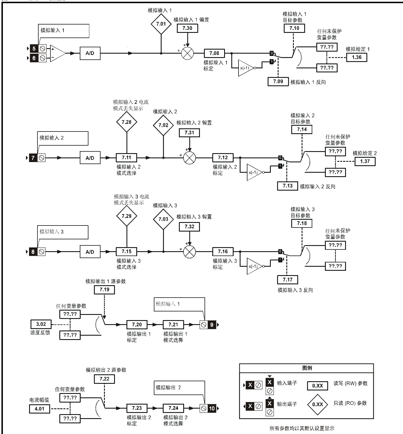
图 11-8 菜单 7 逻辑图
