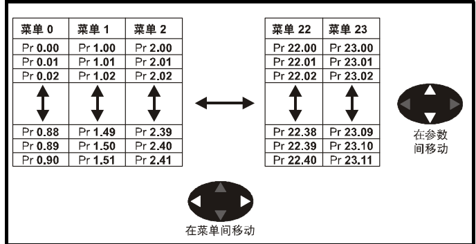
图 5-7 菜单结构
