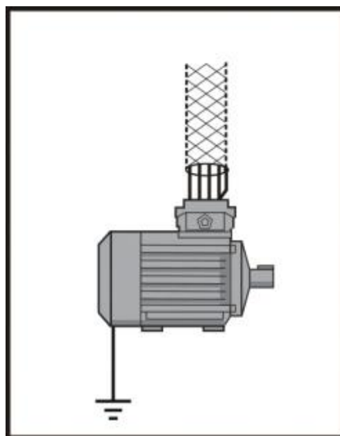
图 3-45 电机线缆屏蔽接地
