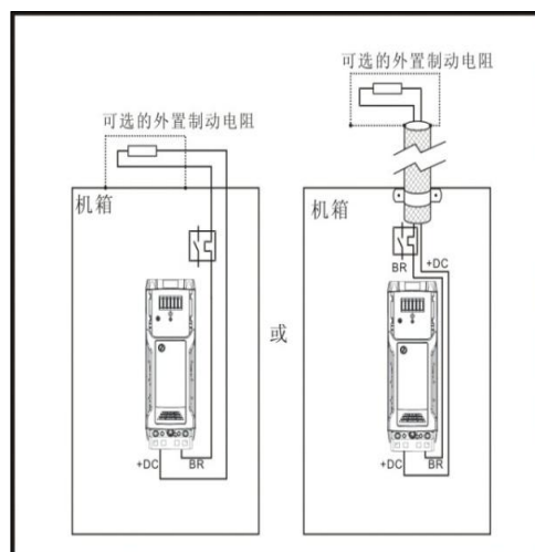
图 3-46 可选外置制动电阻器的屏蔽要求
