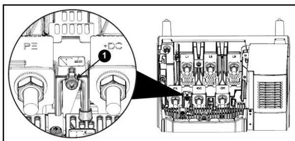
图 3-38 Size7-8 内置 EMC 滤波器移除示意图
