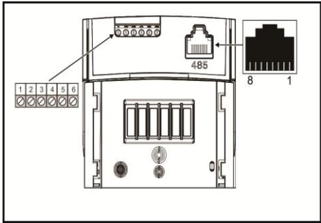
图 3-30 外置 RS485 通讯卡配线
