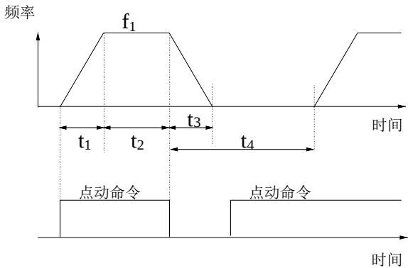
图 5-15 点动运行参数说明
