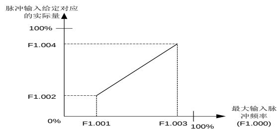
图 5-4 端子脉冲给定正作用特性
