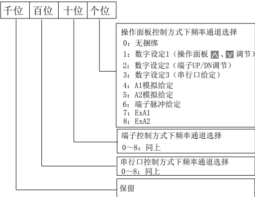
图 5-46 运行命令通道捆绑频率给定通道
