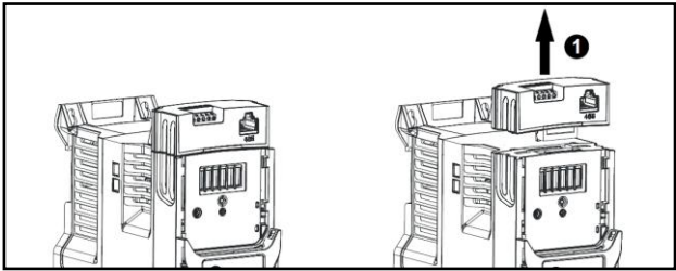
图 3-8 外置 RS485 通讯卡拆卸示意图
