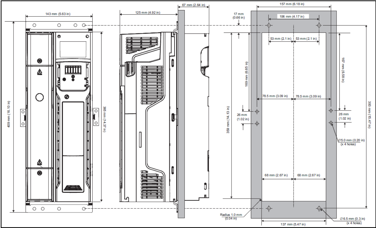
图 3-11 Size5 透壁式安装尺寸图
