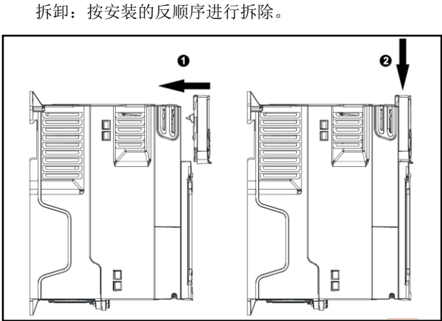
图 3-9 LCD 键盘安装示意图
