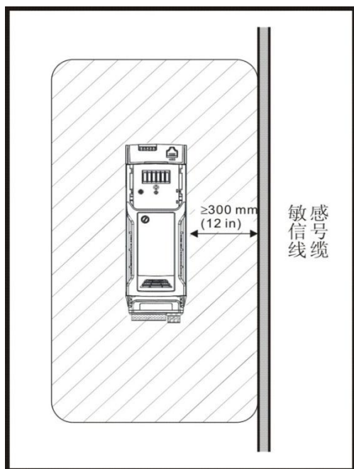
图 3-43 敏感信号电路间距
