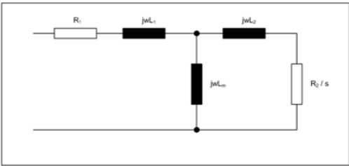
图 5-61 异步电机稳态等效电路图
