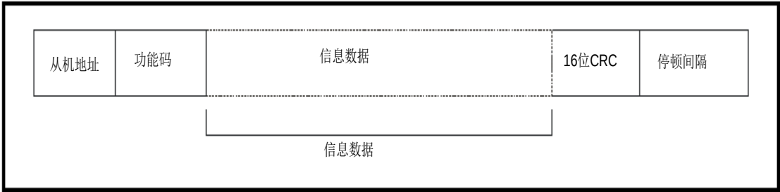
附图 4 帧格式
