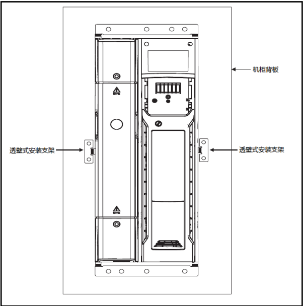
图 3-18 透壁式安装示意图
