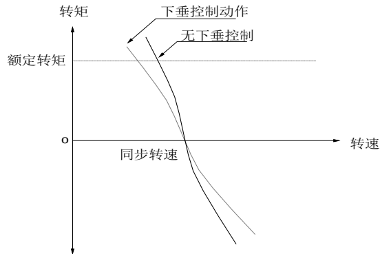
图 5-50 下垂控制电机特性
