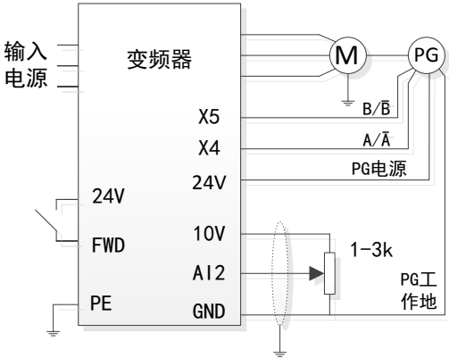
图 5-23 PG 速度闭环控制系统接线图
