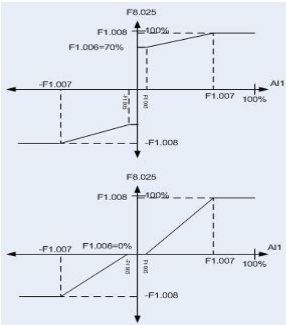
图 5-6 模拟输入 AI1 给定正作用特性
