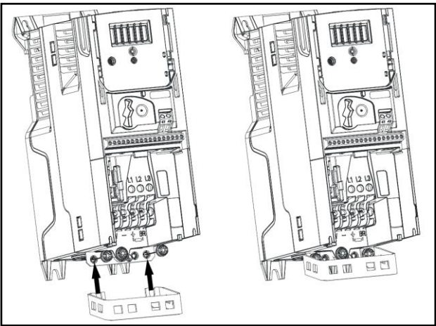
图 3-31 Size2-4 接地支架安装示意图
