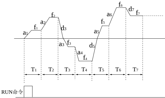
图 5-56 PLC 单循环后保持方式
