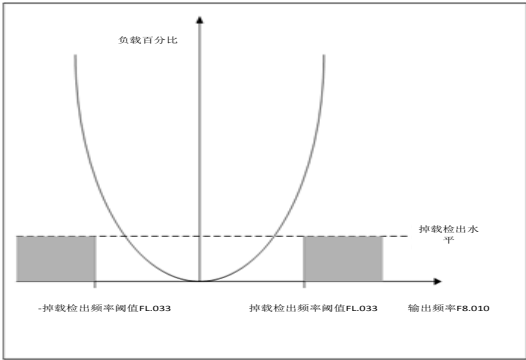
图 5-65 掉载检出示意图
