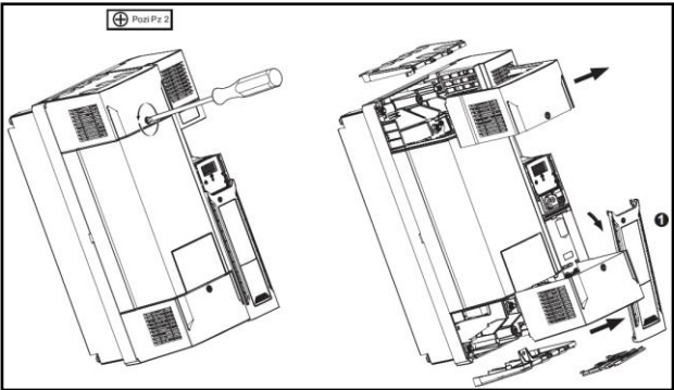
图 3-3 size5 ~ 8 盖板拆卸示意图
