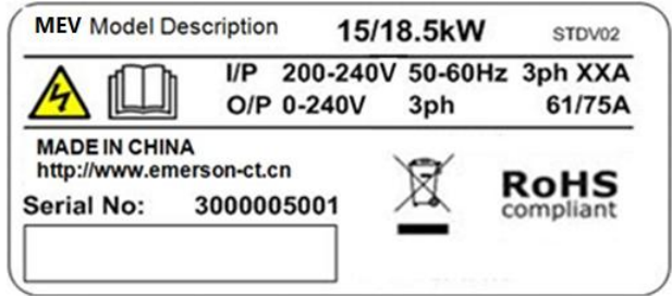
图 A-3 变频器铭牌
