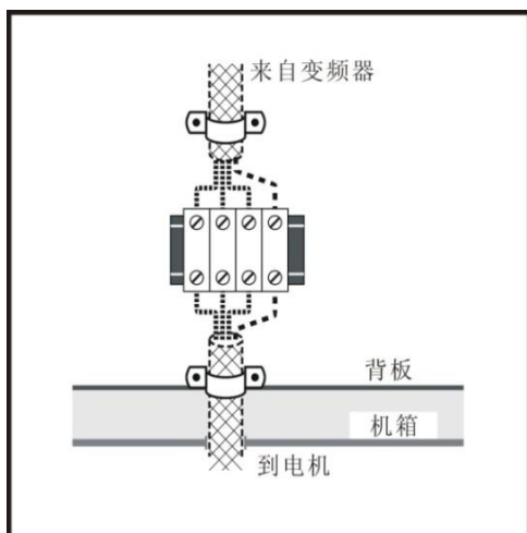
图 3-48 将电机线缆连至柜内接线端子
