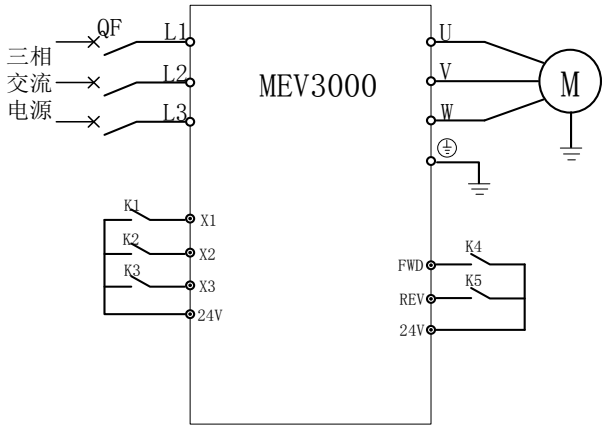
图5-35中以端子运行命令通道为例，由K4、K5可以对运行方向进行控制。通过K1、K2、K3的不同逻辑组合，可以按上表格选择普通运行频率和1~7段多段频率进行多段速度运行。
