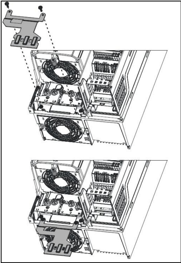
图 3-34 Size6 接地夹钳安装示意图
