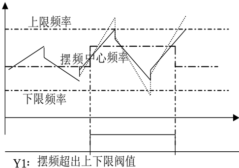
图 5-37 摆频幅度限制
