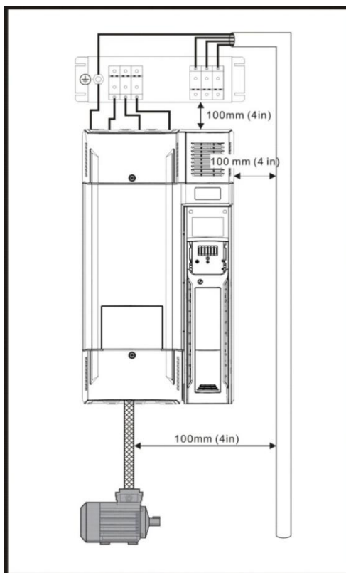
图 3-42 电源及接地线缆间距（Size7,8,9）
