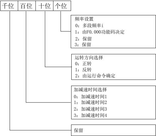
图 5-60 PLC 阶段 i 设置 (i=1~7)
