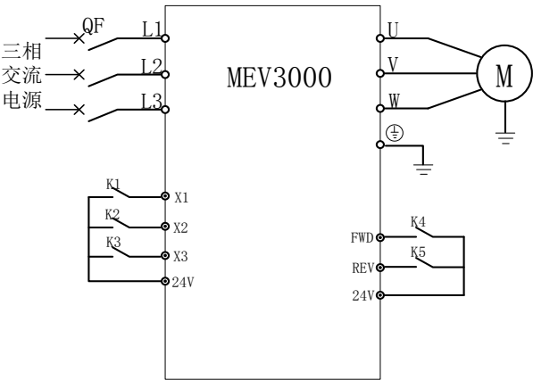
图 5-35 多段速度运行示意图
