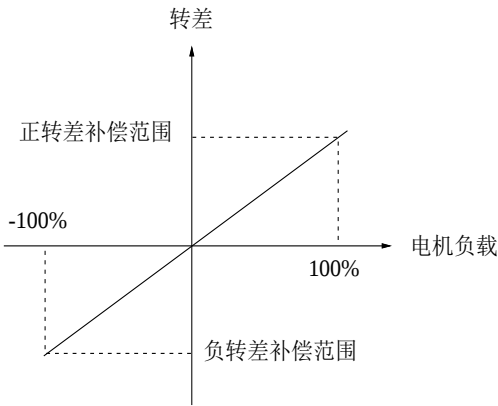
图 5-14 自动转差补偿
