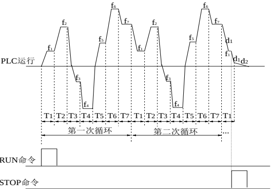
图 5-57 PLC 连续循环方式
