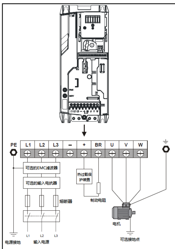
图 3-24 Size4 主回路输入输出连接图
