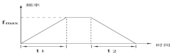
图 5-11 直线加减速
