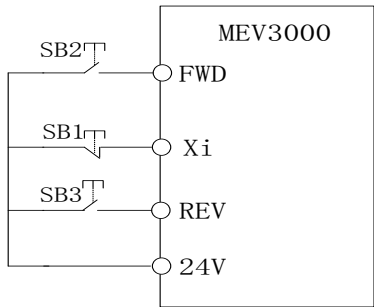
图 5-40 三线式运转模式 1
