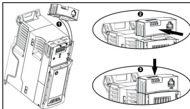
图 3-7 外置 RS485 通讯卡安装示意图
