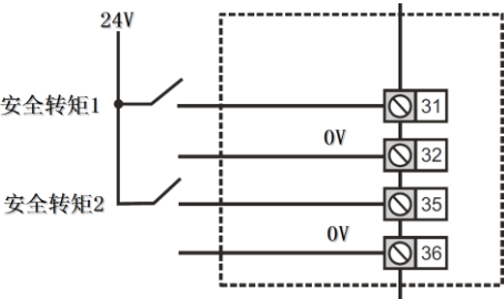
图 3-29 Frame 5-9 STO 端子连接图
