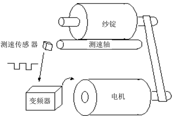
图 5-52 定长停机功能的应用
