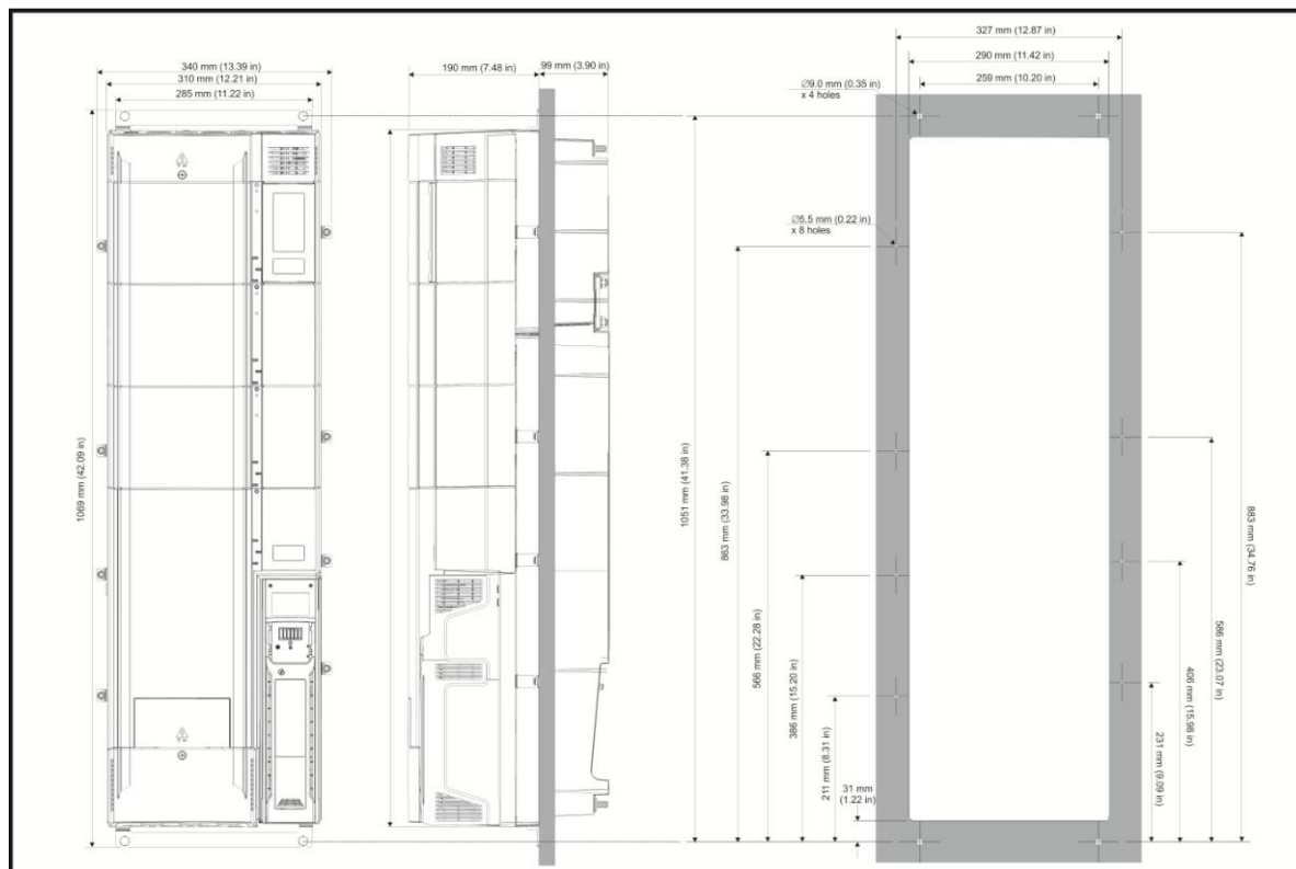
图 3-15 Size9 透壁式安装尺寸图
