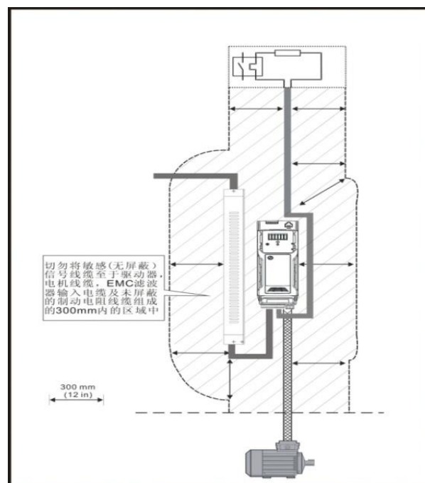
图 3-40 变频器线缆间隔
