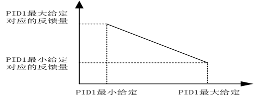
图 5-27 给定、反馈曲线示意图
