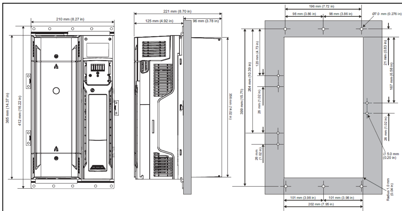
图 3-12 Size6 透壁式安装尺寸图
