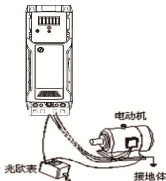
图 1-1 电机绝缘检查示意图
