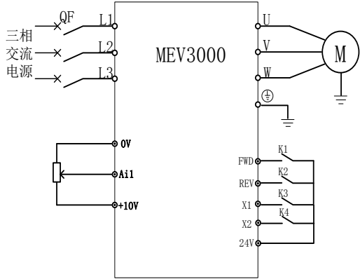
图 5-48 两地控制硬件接线图
