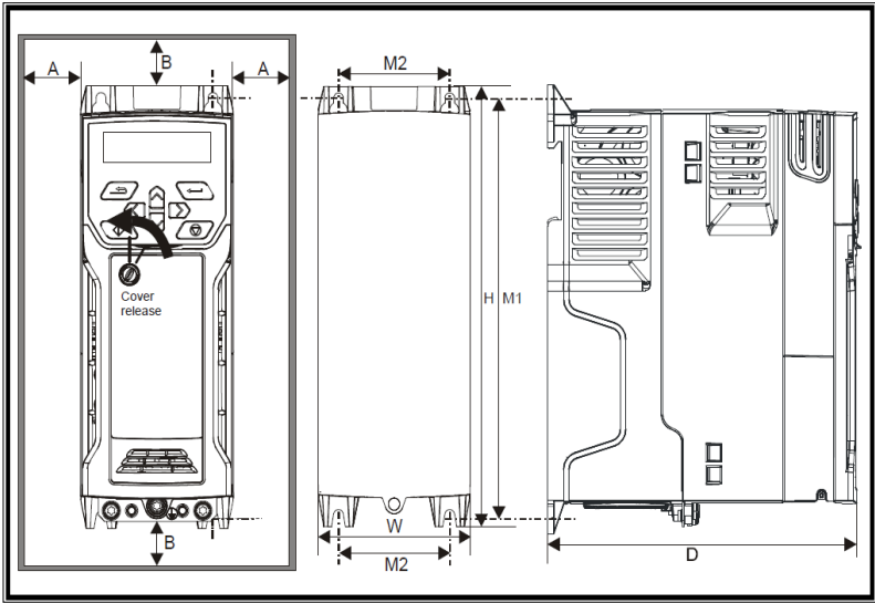
图 3-10 MEV3000 变频器外形图
