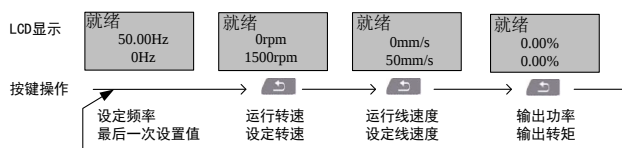
图4-5 停机状态参数显示操作示例
