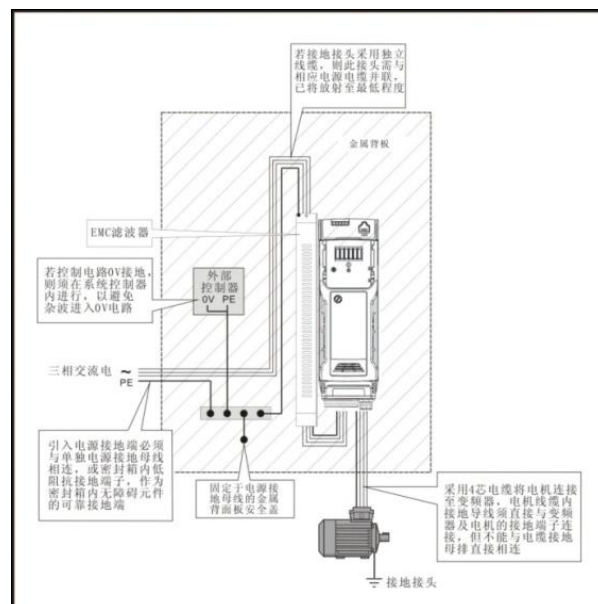
图 3-39 一般 EMC 机壳所示接地连接
