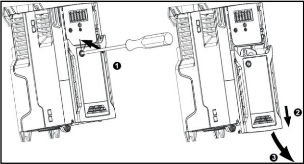
图 3-2 size4 盖板拆卸示意图
