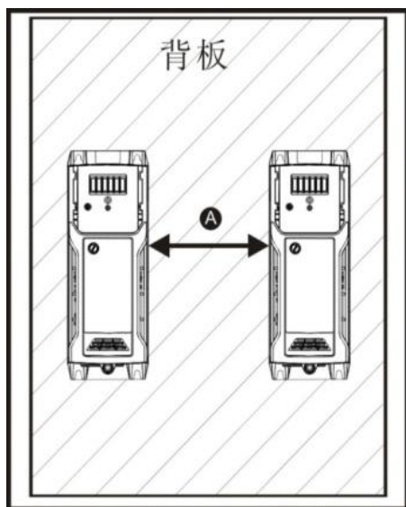
图 3-1 安装间距距离
