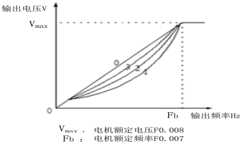
图 5-2 降转矩曲线
