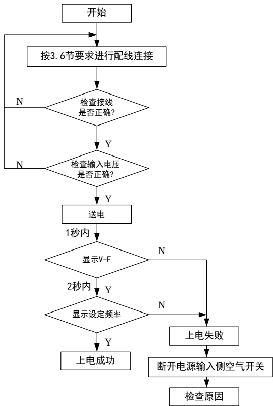
图 4-11 变频器初次上电操作流程
