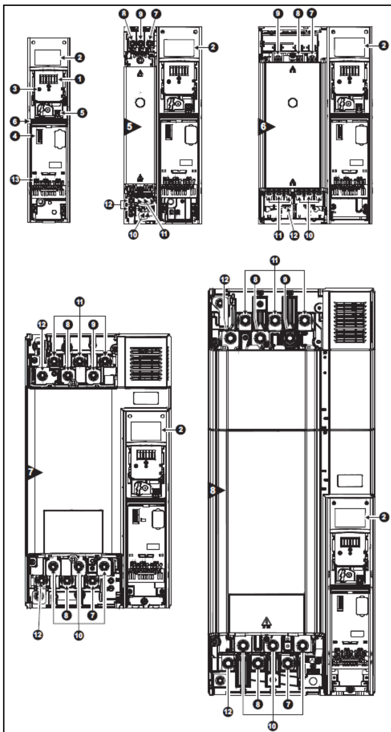
图 2-2 Size 5~8 变频器各部位名称示意图
