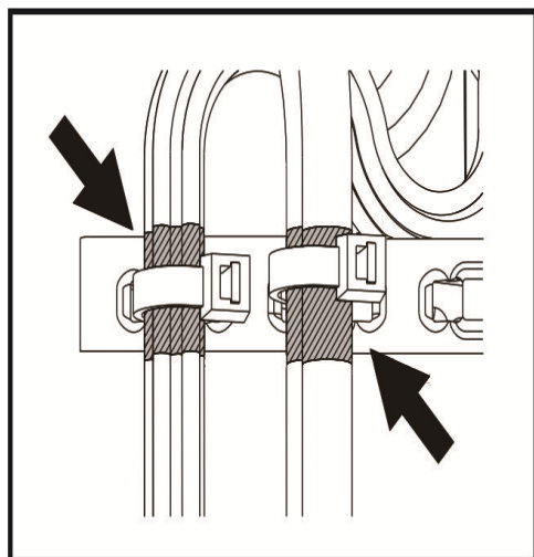
图 3-47 使用接地支架进行信号线缆屏蔽接地
