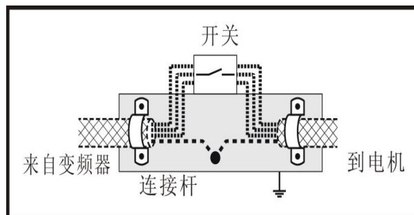
图 3-49 连接电机电缆至隔离开关
