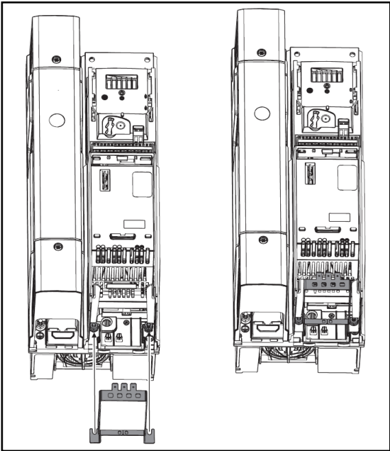
图 3-32 Size5-8 接地支架安装示意图（size5 为例）
