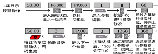
图 4-8 用户密码锁定操作示例
