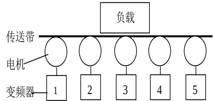
图 5-49 下垂控制示意图
