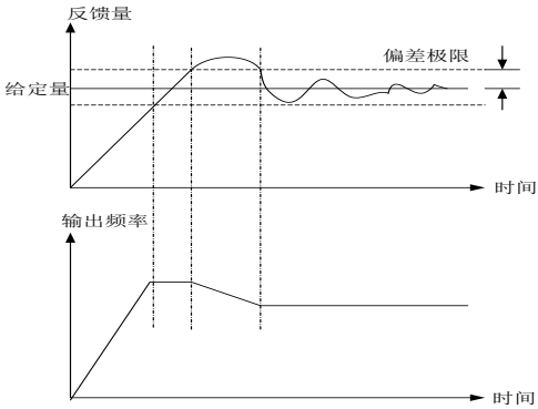
图 5-28 偏差极限示意图 1
