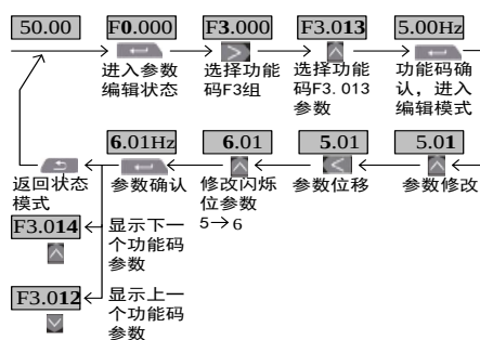
图4-6 参数编辑操作示例
