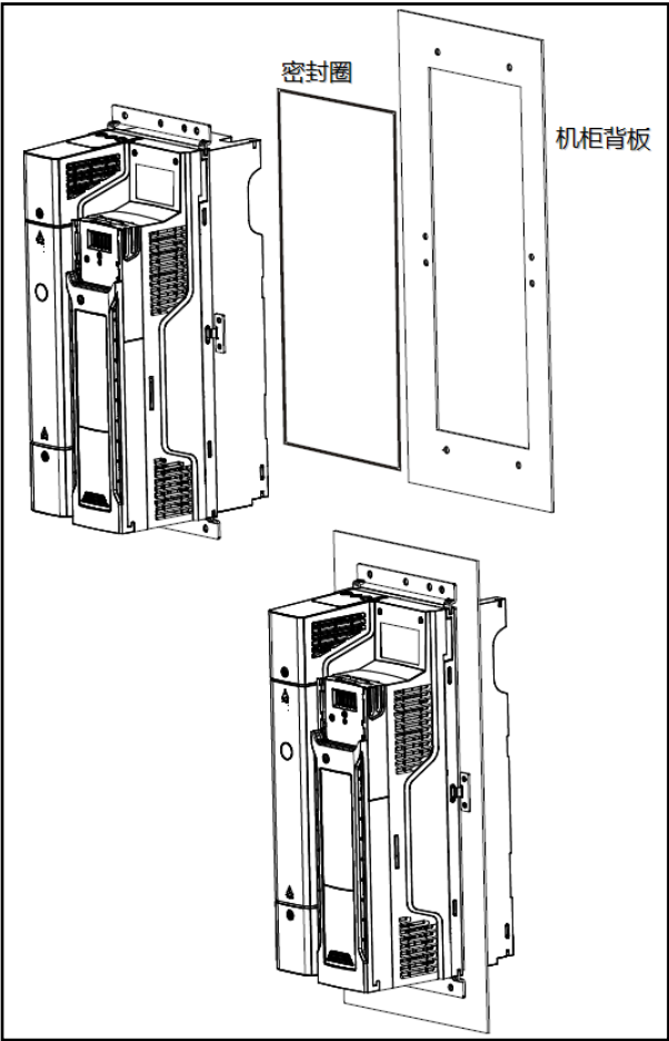
图 3-17 安装密封圈
