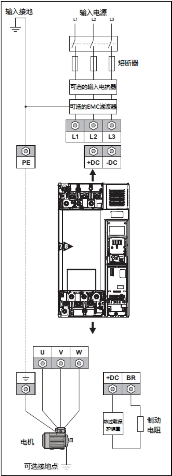
图 3-27 Size7~9 主回路输入输出连接图
