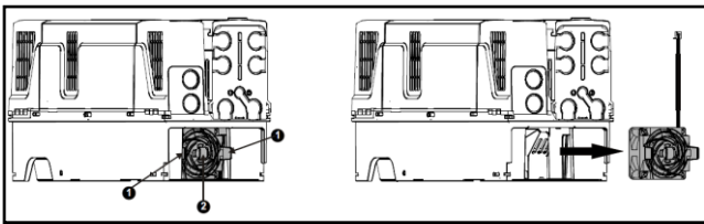
图 3-20 风扇拆除示意图
