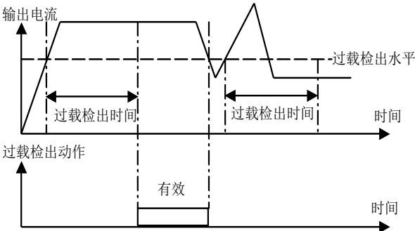
图 5-63 过载预警检出功能示意图
