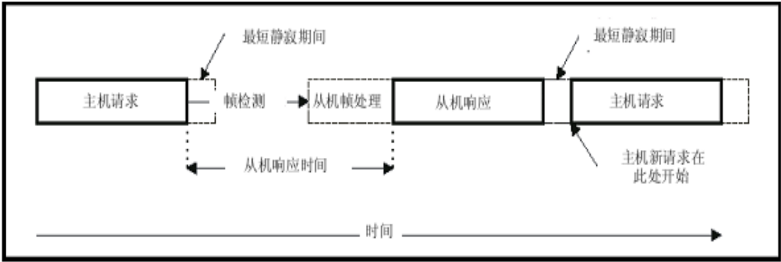
附图 5 主从通讯时间示意图
