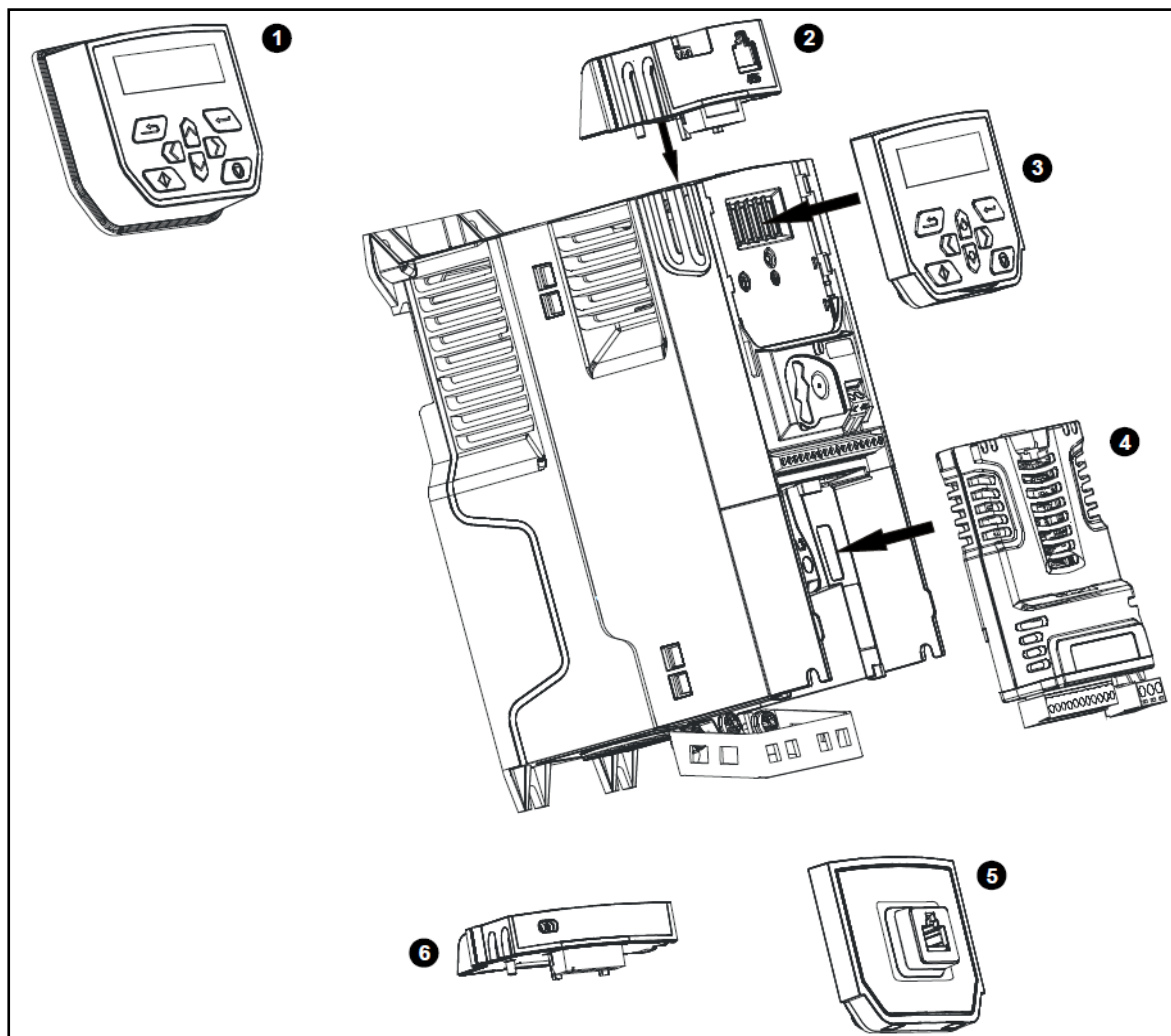
图 2-3 MEV3000 可支持的配件
