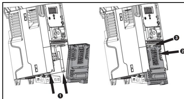
图 3-5 选件卡安装示意图
