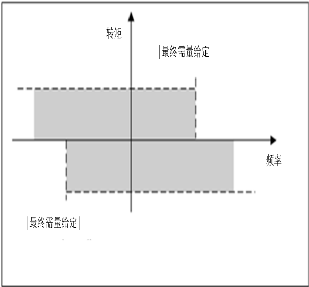
图 5-21 带频率限幅的双向转矩控制
