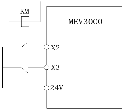
图 5-36 外部设备故障常开/常闭输入示意图
