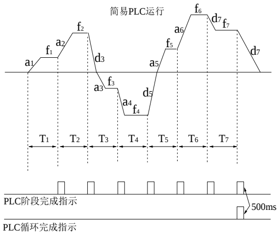
图 5-53 简易 PLC 运行图
