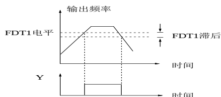
图 5-43 频率水平检测示意图
