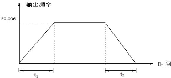
图 5-1 加减速时间定义
