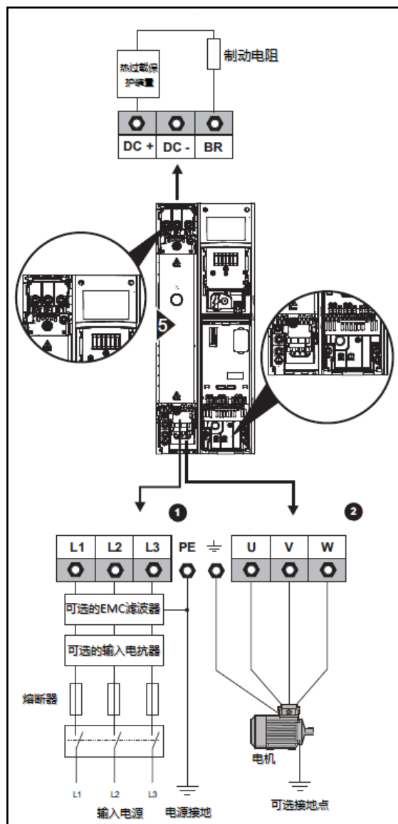
图 3-25 Size5 主回路输入输出连接图
