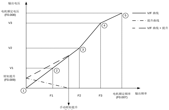
图5-3 自定义V/F曲线
