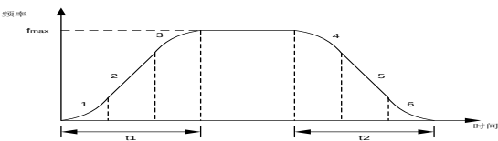
图 5-12 S 曲线加减速
