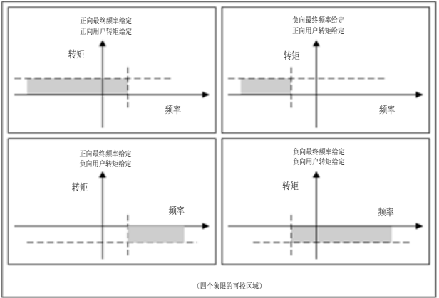
图5-18 带频率限幅的转矩控制
