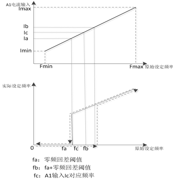
图 5-51 零频回差运行
