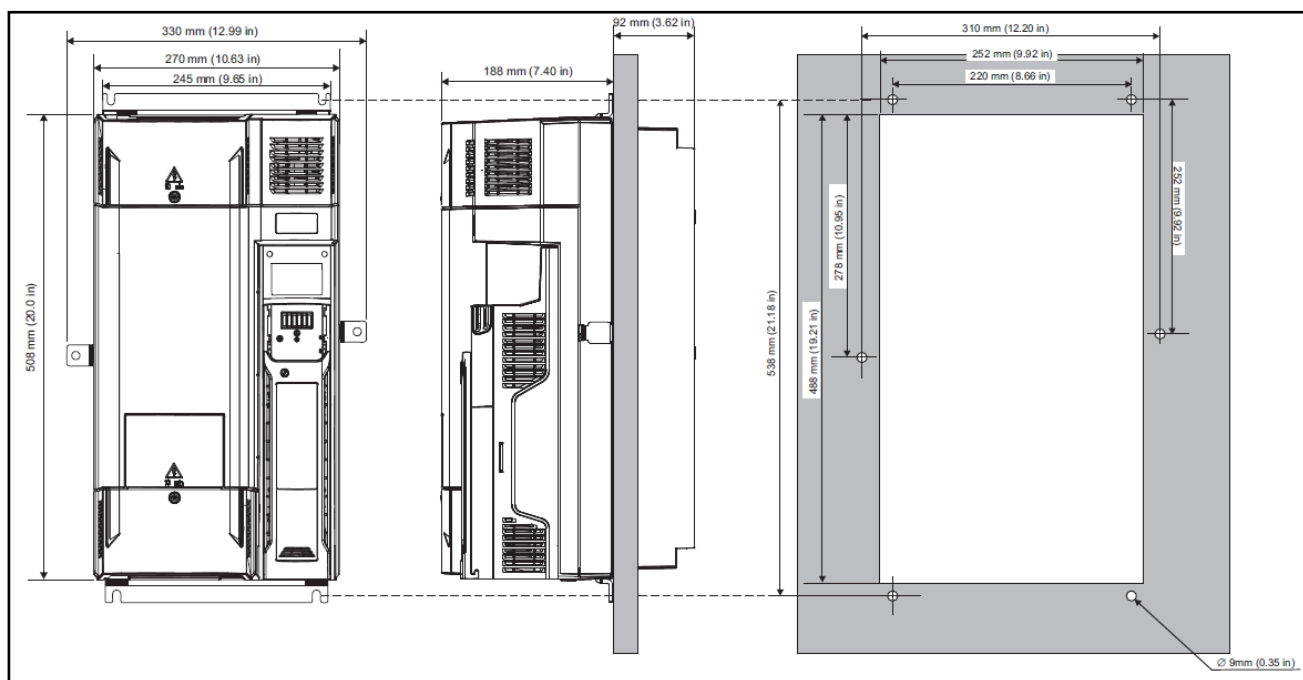
图 3-13 Size7 透壁式安装尺寸图
