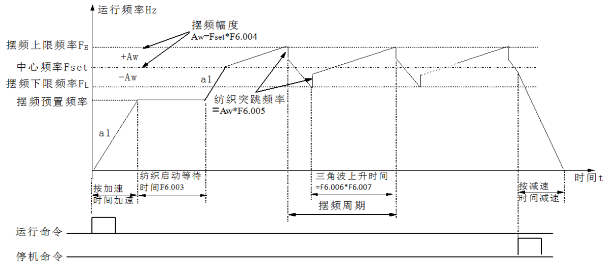
图 5-30 摆频示意图
