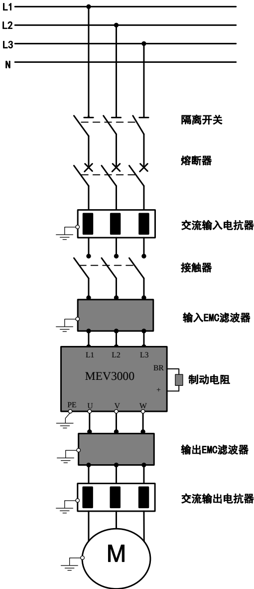
图 3-21 变频器与选配件的连接
