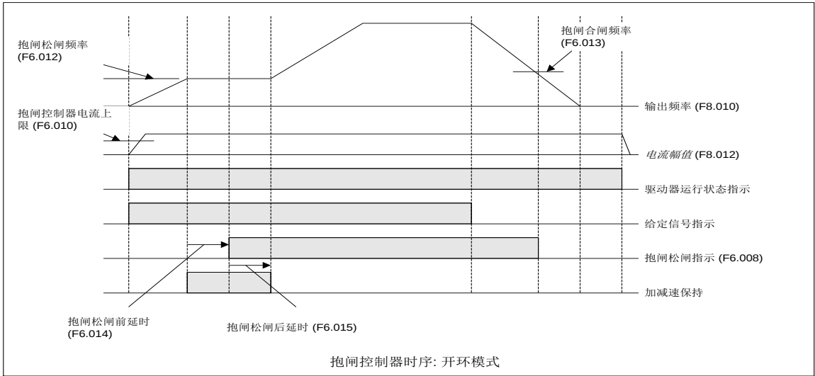
图 5-32 抱闸控制器时序：开环模式
