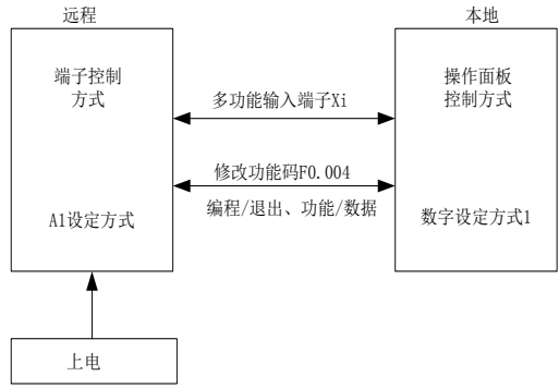
图 5-47 两地控制需求
