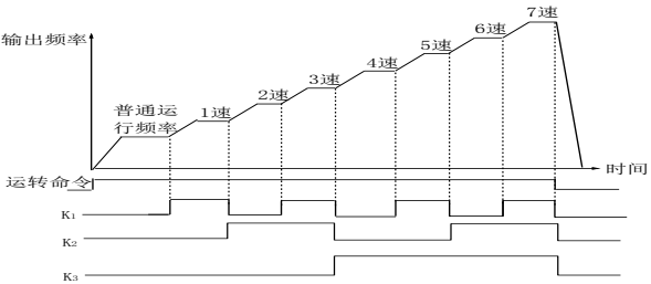
图 5-34 多段速度运行示意图
