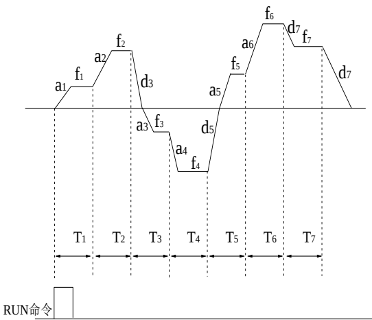
图 5-55 PLC 单循环后停机方式
