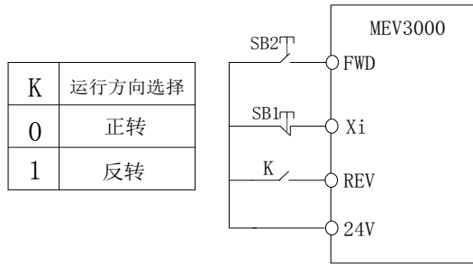
图 5-41 三线式运转模式 2
