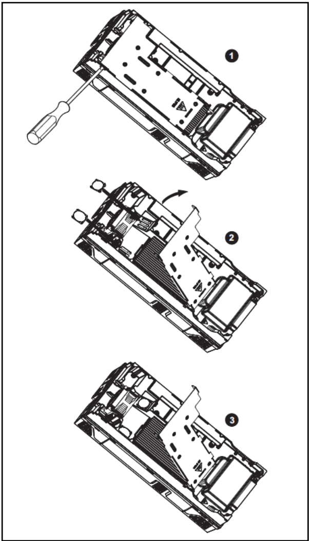
图 3-19 安装 IP 插片
