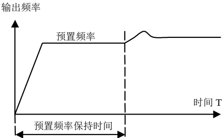
图 5-29 闭环预置频率运行示意图
