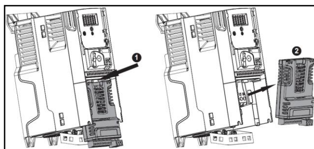
图 3-6 选件卡拆卸示意图
