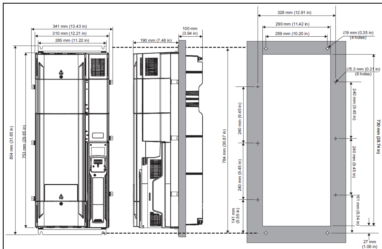
图 3-14 Size8 透壁式安装尺寸图
