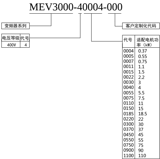
图 A-2 变频器型号说明
