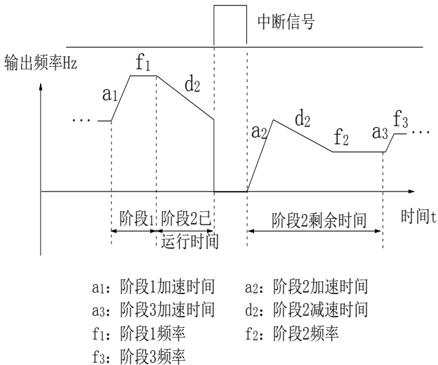
图 5-59 PLC 起动方式 2
