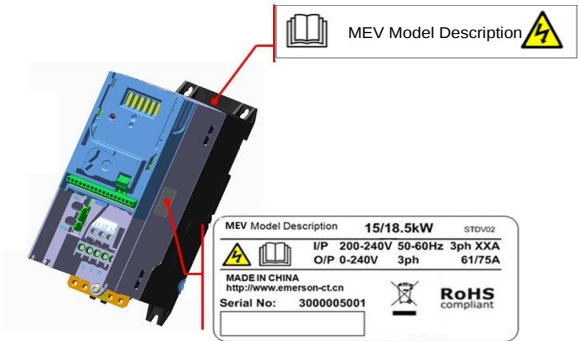
图 A-1 图铭牌和条码位置示意图
