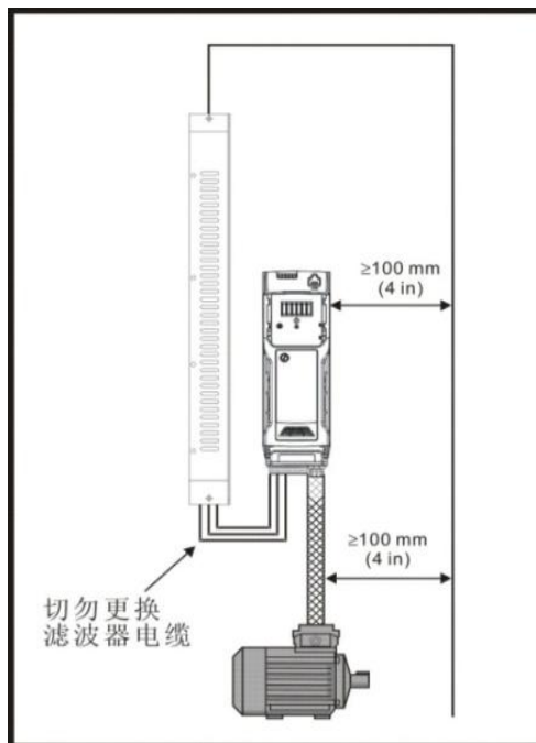
图 3-41 电源及接地线缆间距（Size2-6）
