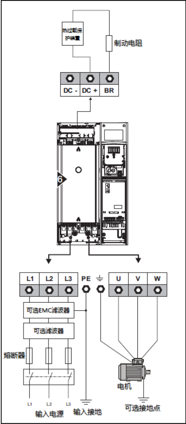
图 3-26 Size6 主回路输入输出连接图
