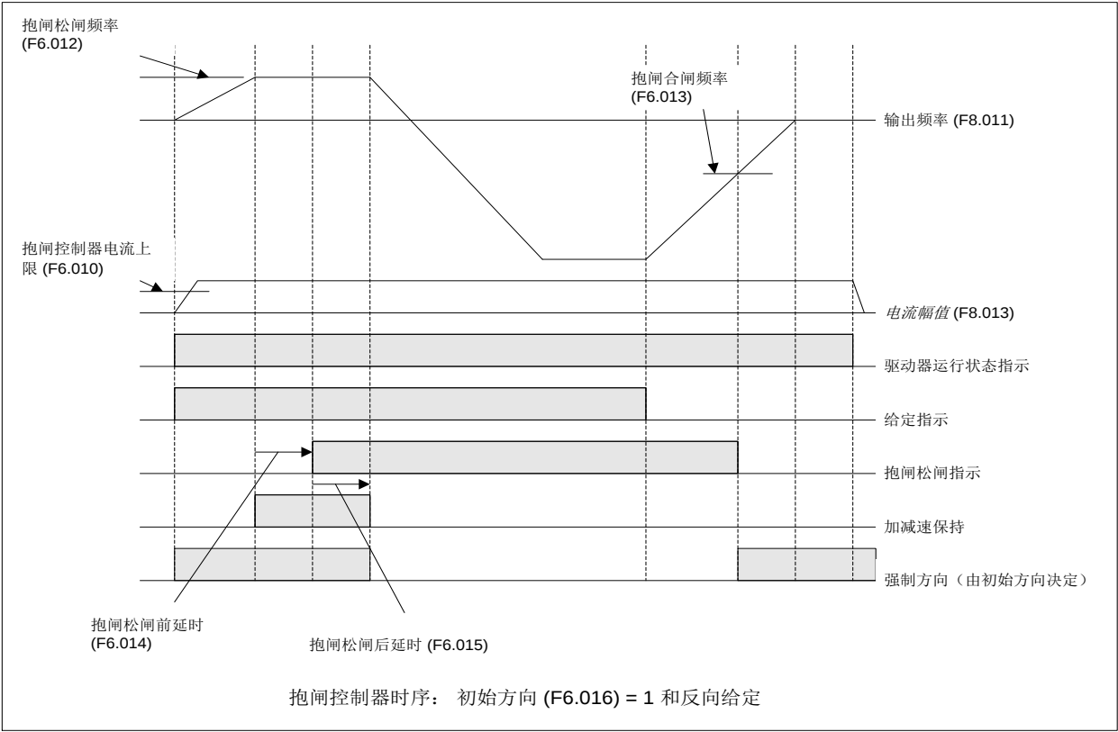
图5- 33 抱闸控制器时序：初始方向（F6.016）=1和反向给定
