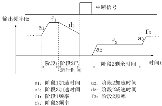
图 5-58 PLC 起动方式 1
