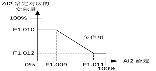
图 5-9 模拟输入 AI2 给定反作用特性
