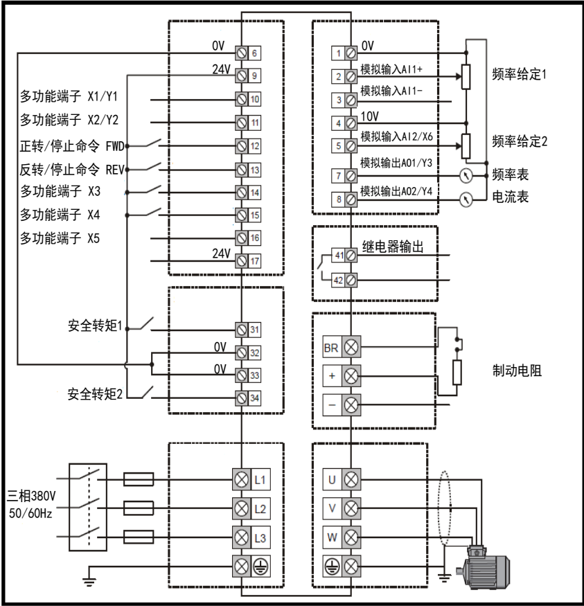
图 3-28 端子连接图
