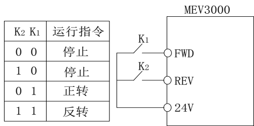
图 5-39 两线式运转模式 2
