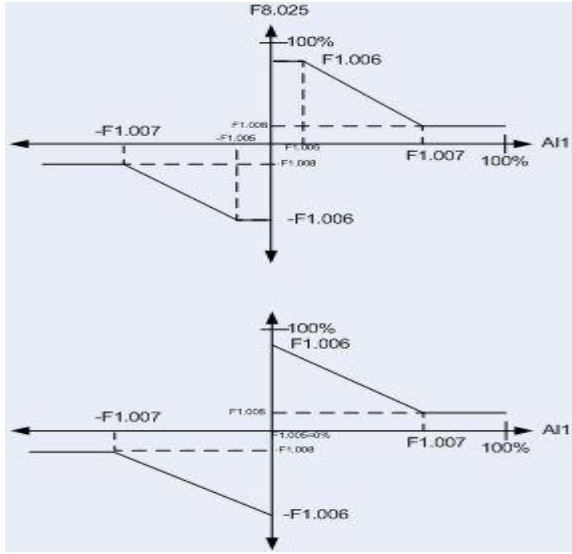
图 5-7 模拟输入 AI1 给定反作用特性
