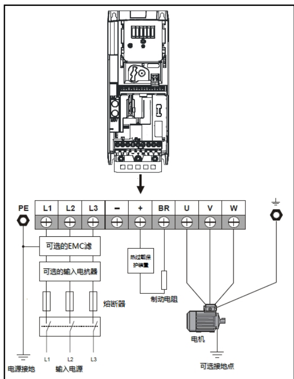
图 3-23 Size3 主回路输入输出连接图
