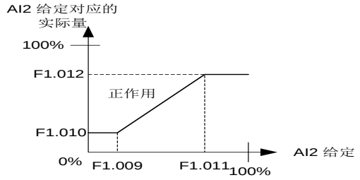
图 5-8 模拟输入 AI2 给定正作用特性
