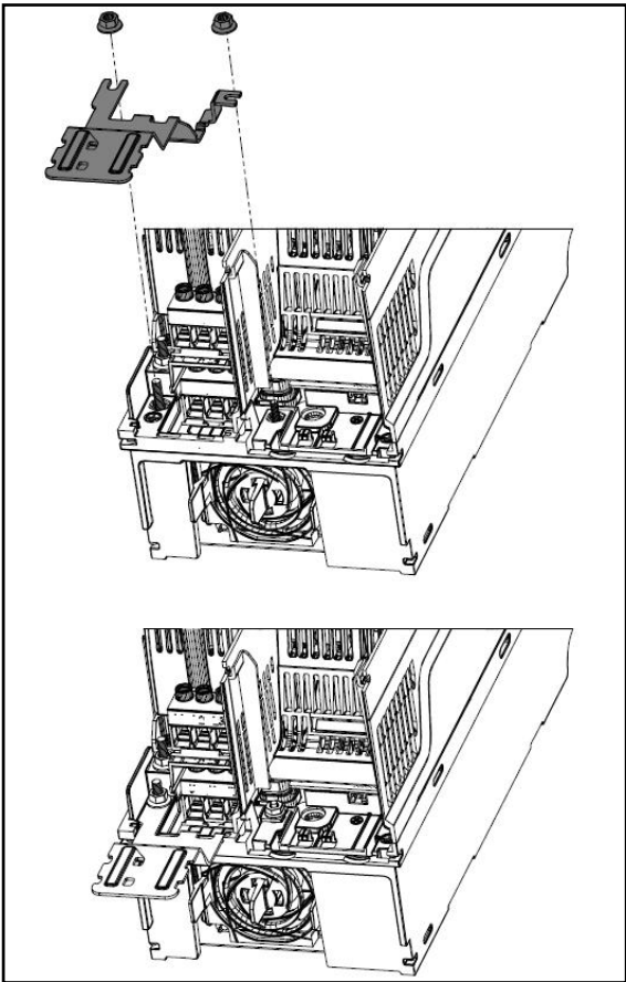
图 3-33 Size5 接地夹钳安装示意图
