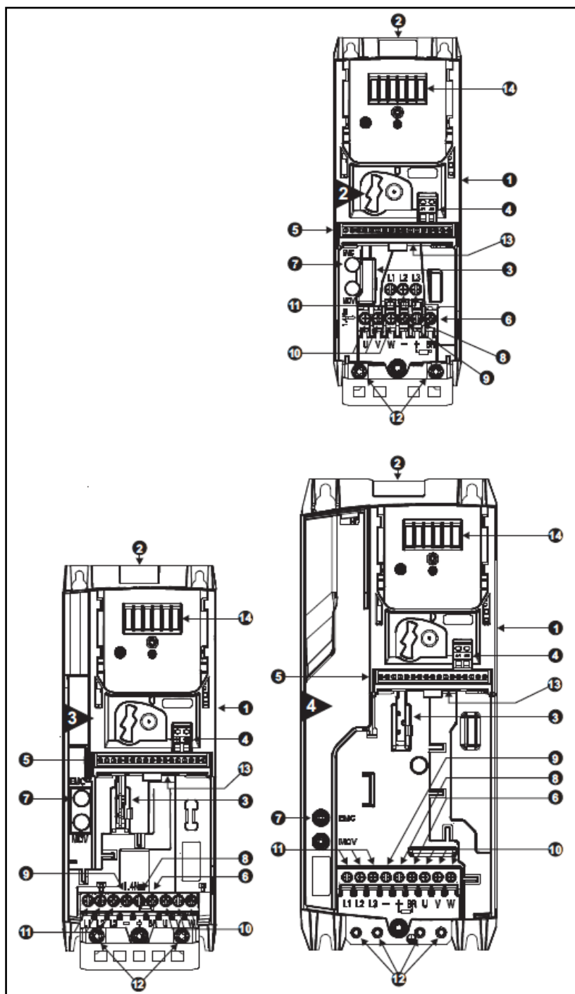
图 2-1 Size 2~4 变频器各部位名称示意图
