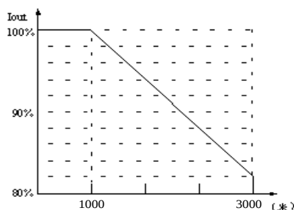
图 1-3 变频器额定输出电流与海拔高度降额使用
