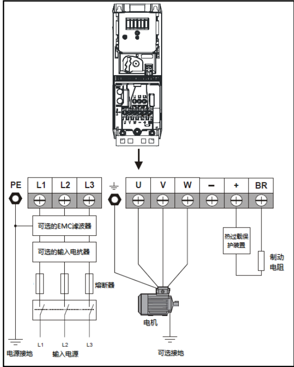
图 3-22 Size2 主回路输入输出连接图
