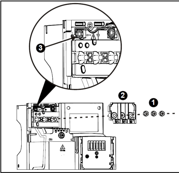
图 3-36 Size5 内置 EMC 滤波器移除示意图
