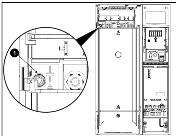
图 3-37 Size6 内置 EMC 滤波器移除示意图
