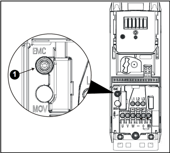
图 3-35 Size2-4 内置 EMC 滤波器移除示意图
