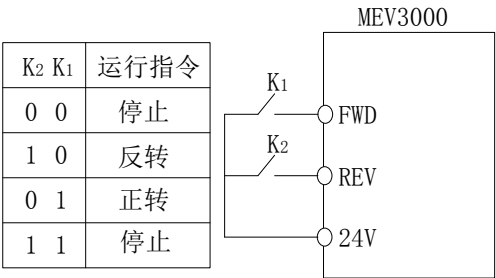
图 5-38 两线式运转模式 1
