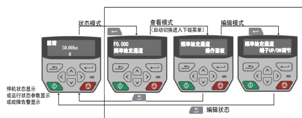
图 4-4 操作面板的编程显示状态
