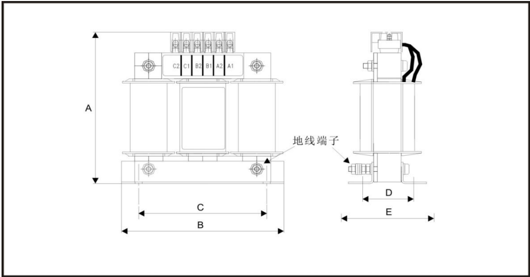
附图 1 交流输入电抗器外形图
