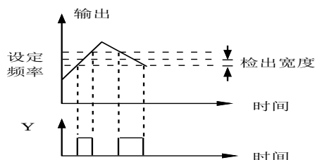
图 5-42 频率到达信号输出示意图
