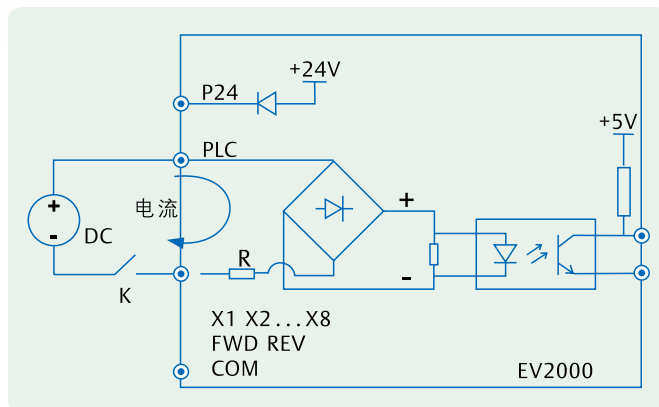
输入开关量接口示意图
