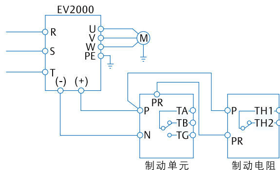
变频器与制动组件连线图
