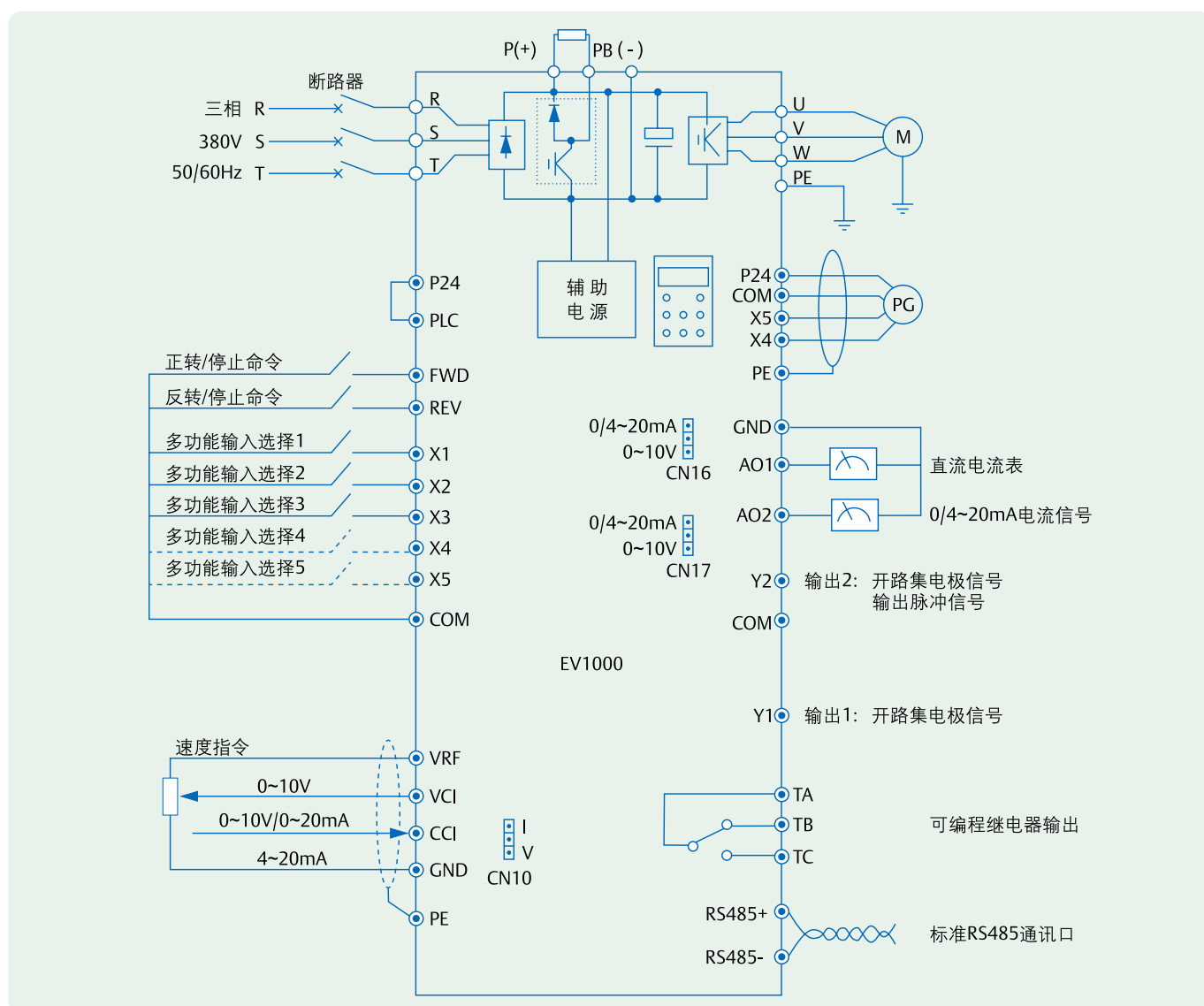
变频器外部接线图
