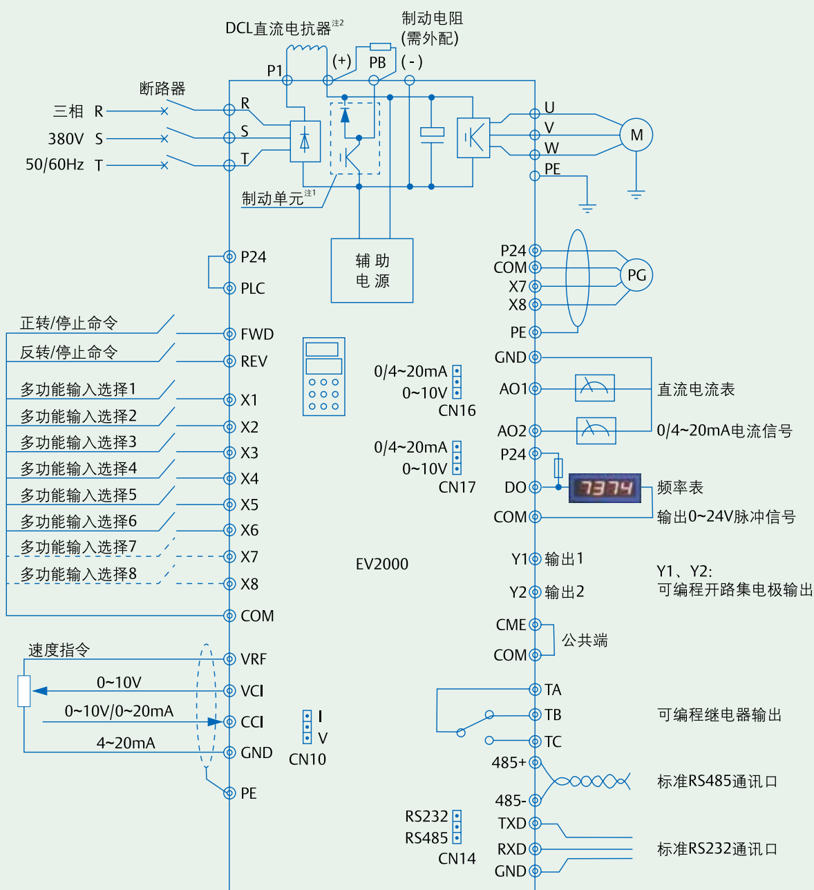
变频器外部接线图
