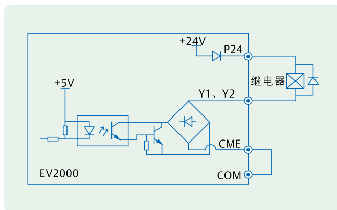
输出开关量接口示意图
