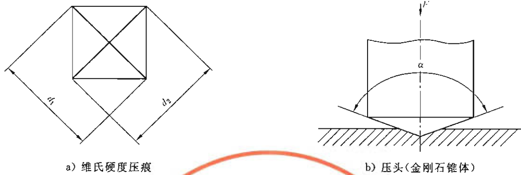
图 1 试验原理
