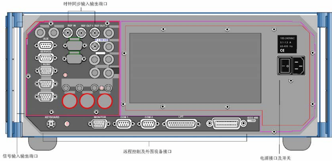
图 2-2 CMU200 后视图
