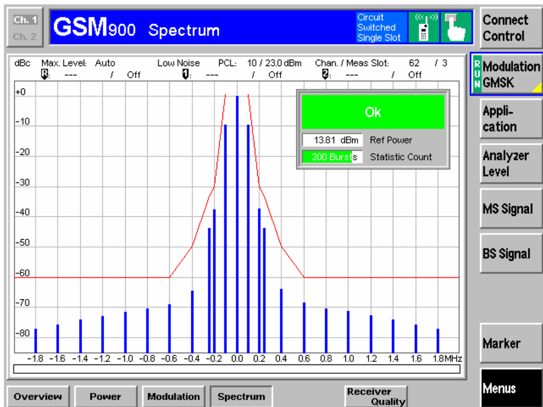
图 2—43 GSM900 Spectrum
