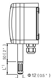
EE33-MFTAx 墙面安装 探头材料: PC
