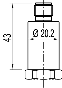
Deutsch connector
