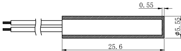
开关组件 Switch Assembly
