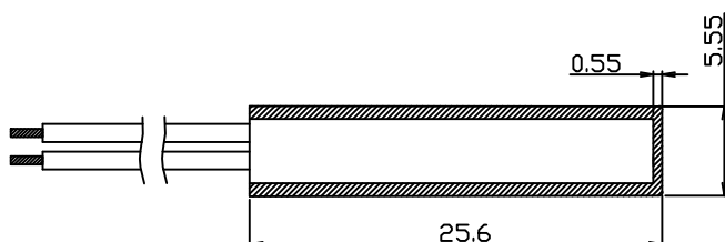
开关组件 Switch Assembly
