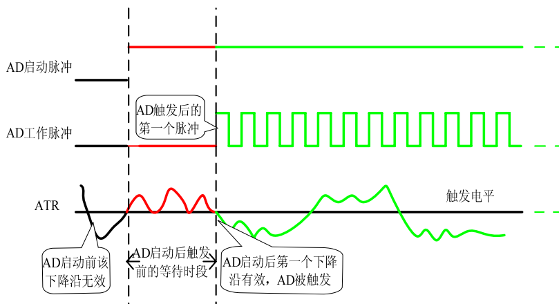
5.3 下降沿触发图例
