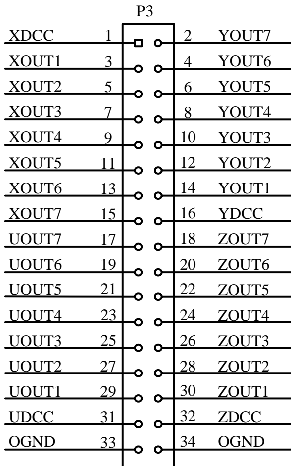
关于 34 芯插头 P3 的管脚定义（表格方式）
