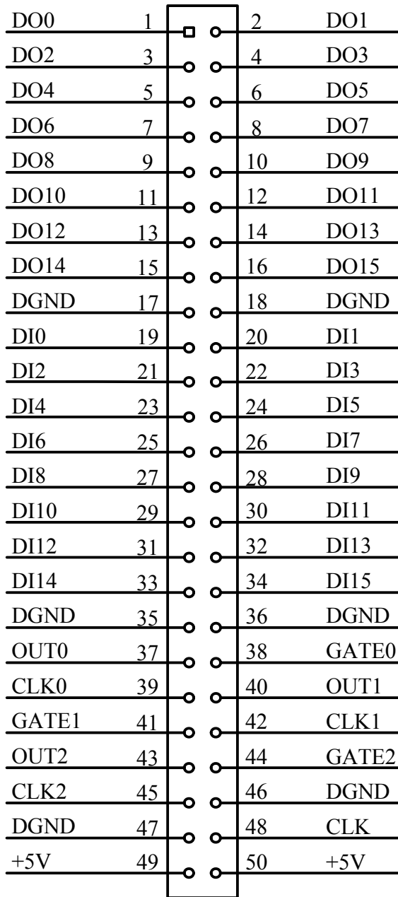
关于 50 芯插座 P1 的管脚定义（表格方式）
