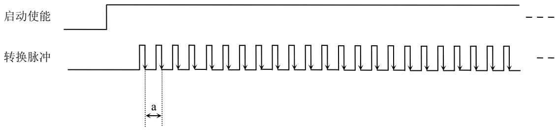
图 7.5 内时钟模式下的连续采集
