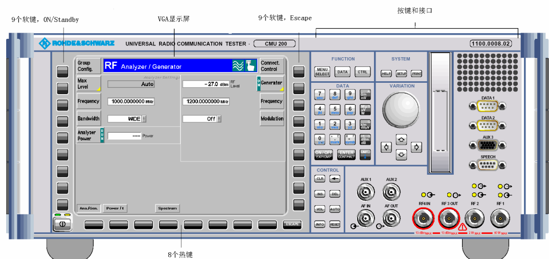
图 2-1 CMU200 前视图
