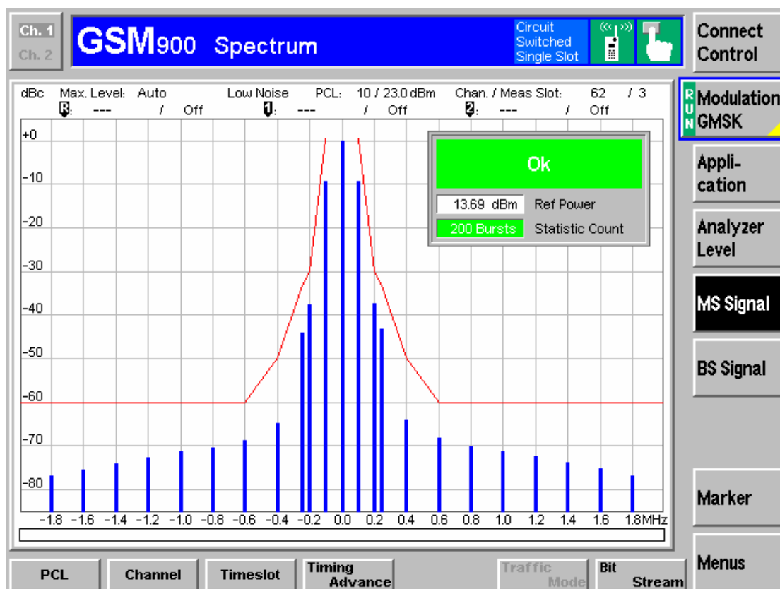
图 2—46 GSM900 Spectrum_MS Signal_Modulation GMSK
