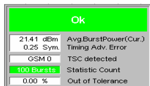
图 2—21 GSM900 Power_P/t Norm. GMSK
