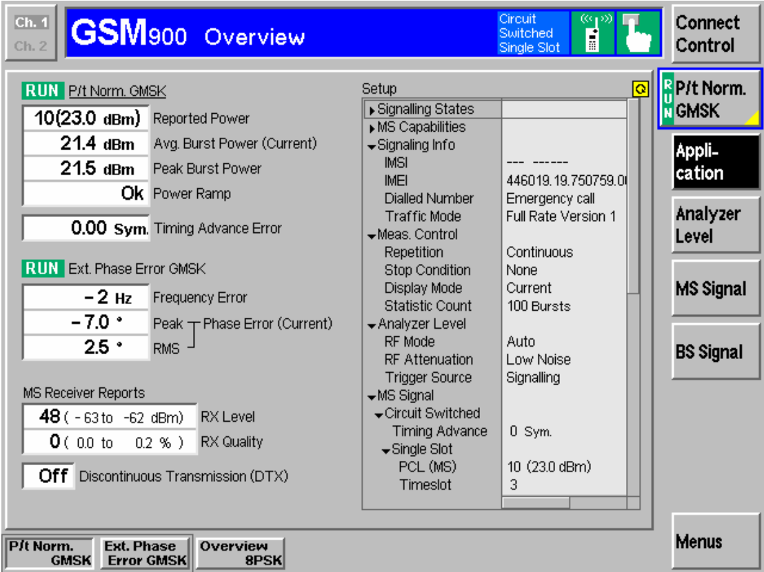
图 2—16 GSM 900 Overview_Application
