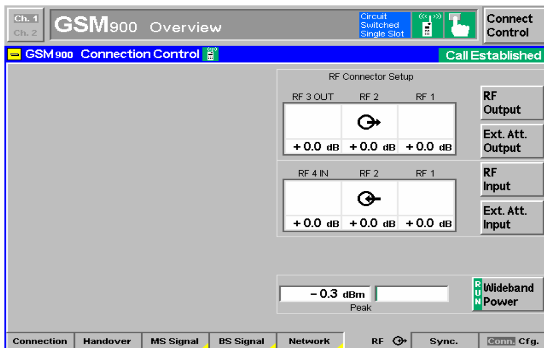
GSM900RF Overview
