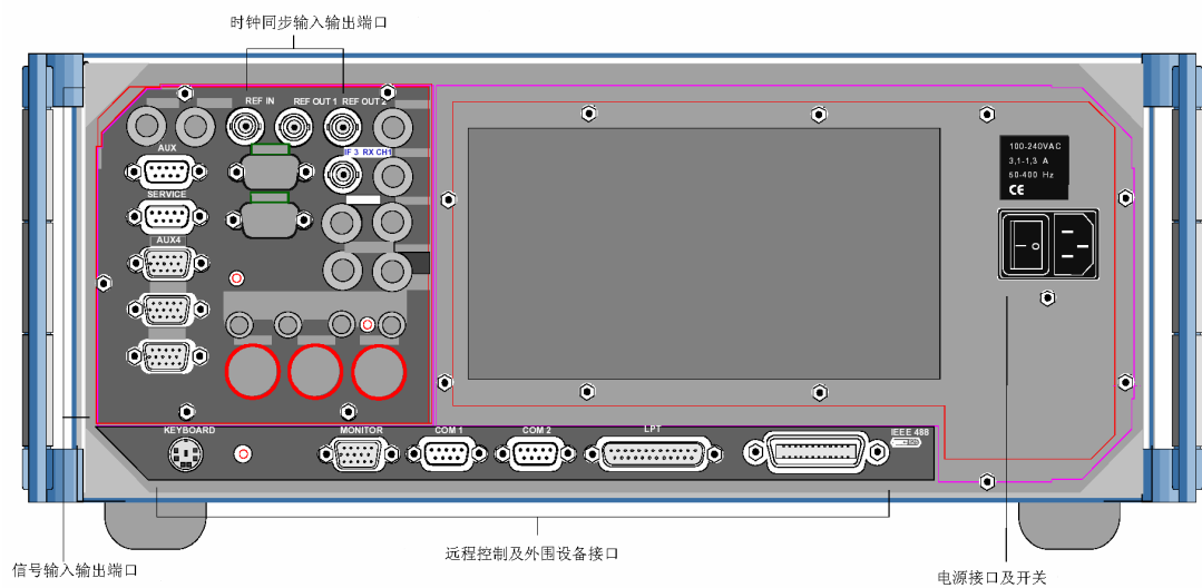
图 2-2 CMU200 后视图
