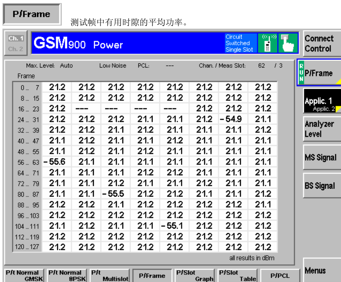
图 2—15 GSM900 Power_Applic.1_P/Frame
