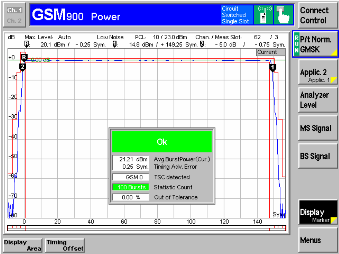
图 2—30 GSM900 Power_Display
