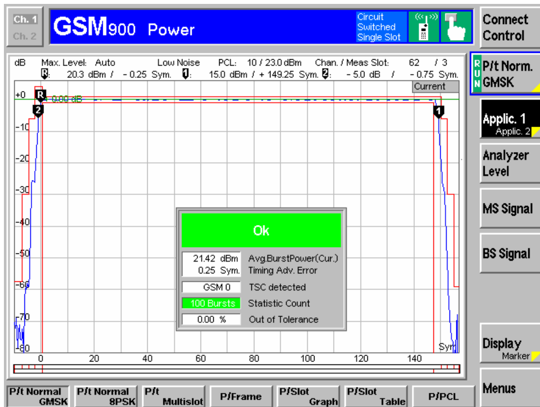
图 2—22 GSM900 Power_Applic.1
