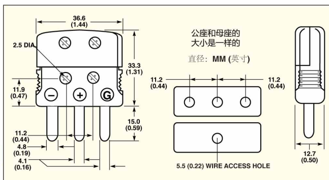
OTP-T-F 母座
