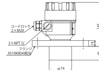
S□□-46G-□ / PP,PVDF
