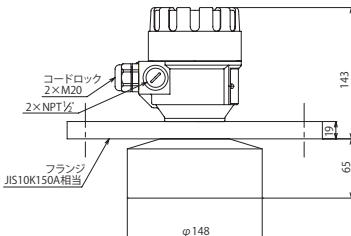
S□□-42R-□ / PP,PVDF
