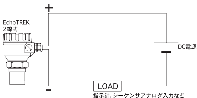
2線式システム図
