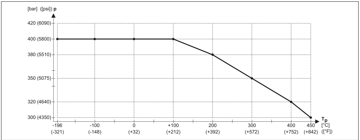
FMP54 -过程压力取决于过程温度
