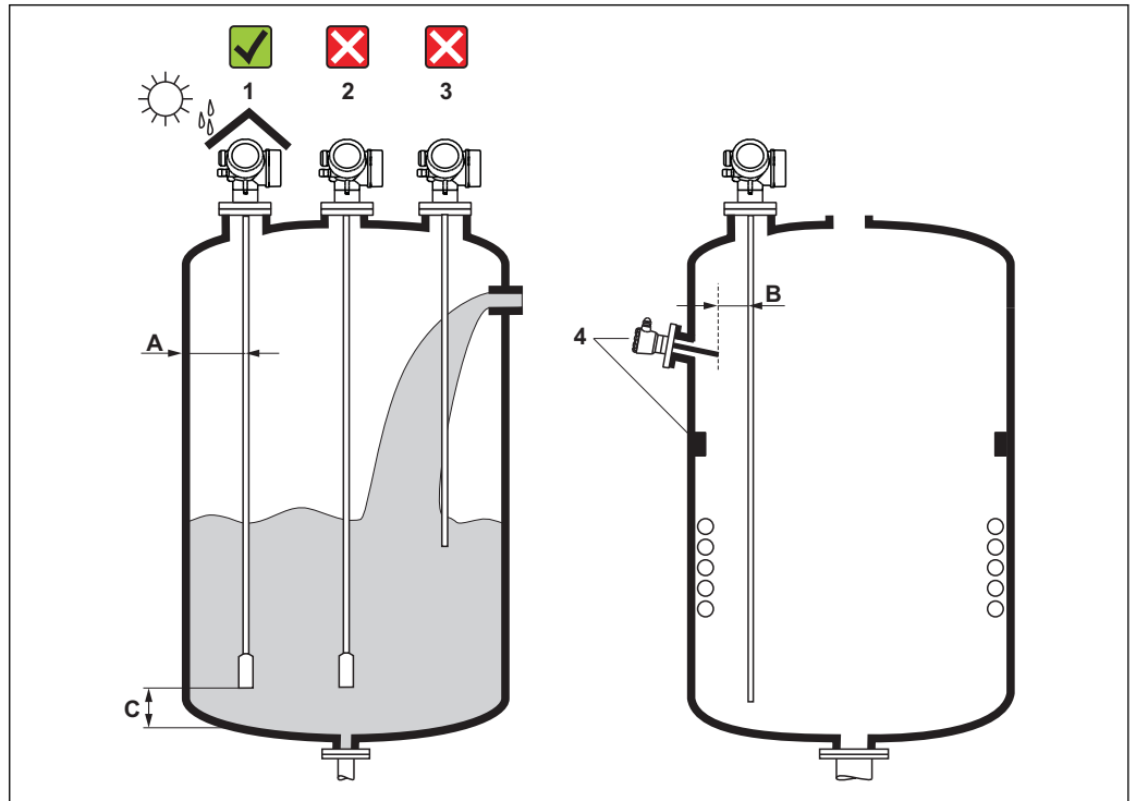
图 17 Levelflex 的安装要求
