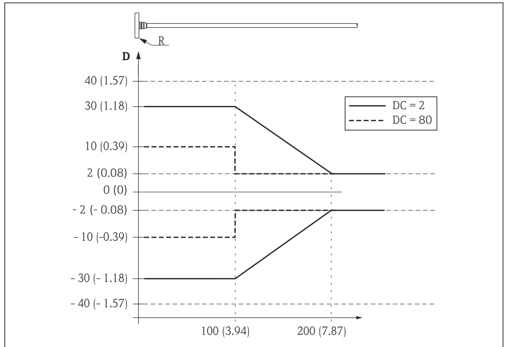
图 16 缆式探头末端出现的测量误差, 单位: mm (in)
