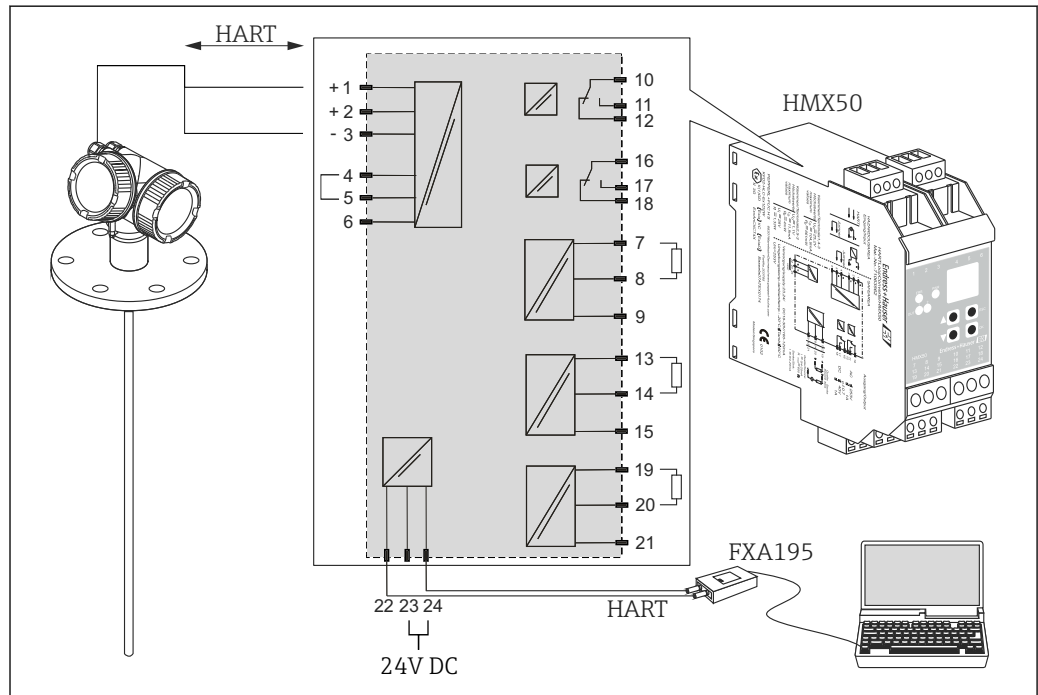
图 12 HART 回路转换器 HMX50 的接线图(实例: 两线制无源设备, 电流输出连接至电源)
