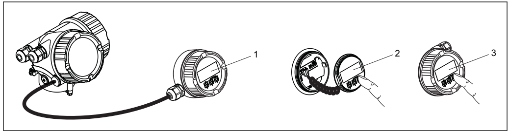
图 33 FHX50 的操作选项
