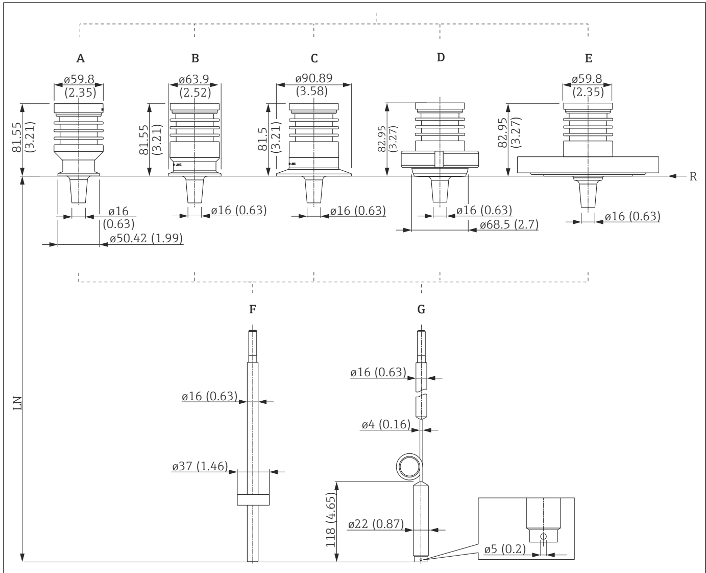
图 31 FMP52: 过程连接/探头; 单位: mm (in)mm (in)。测量单位 mm (in)
