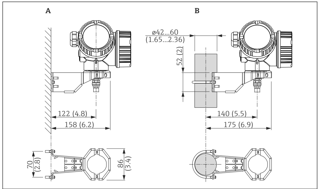
图 27 电子腔外壳的安装支架示意图，单位：mm (in)
