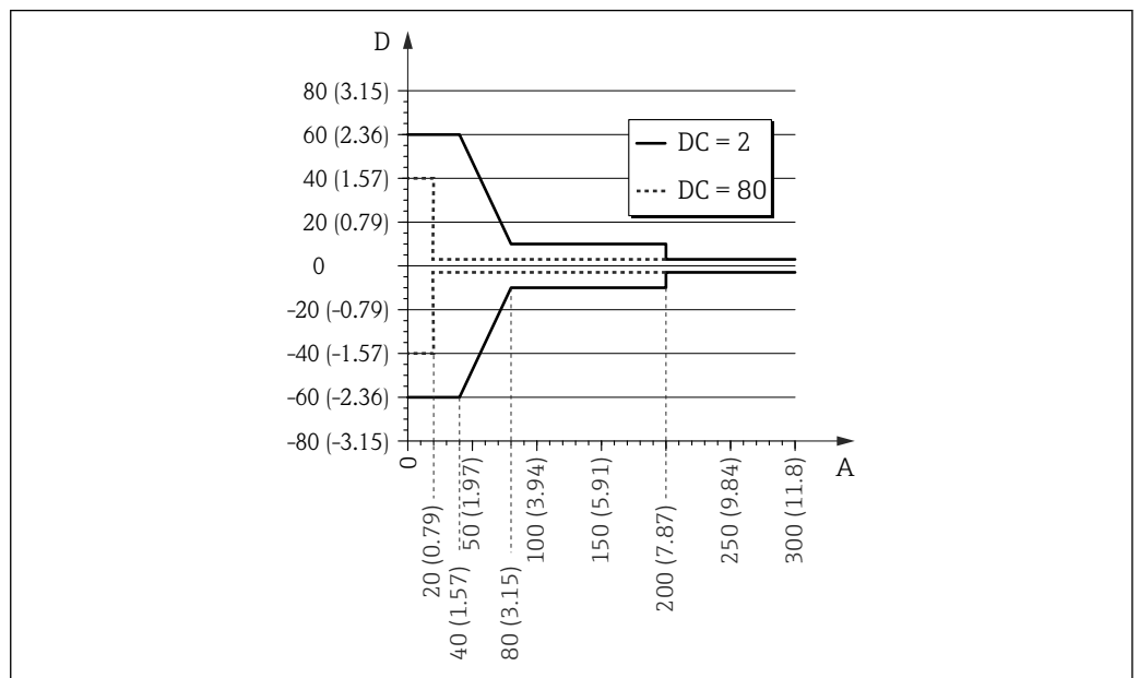
图 13 杆式探头和同轴探头末端出现的测量误差
