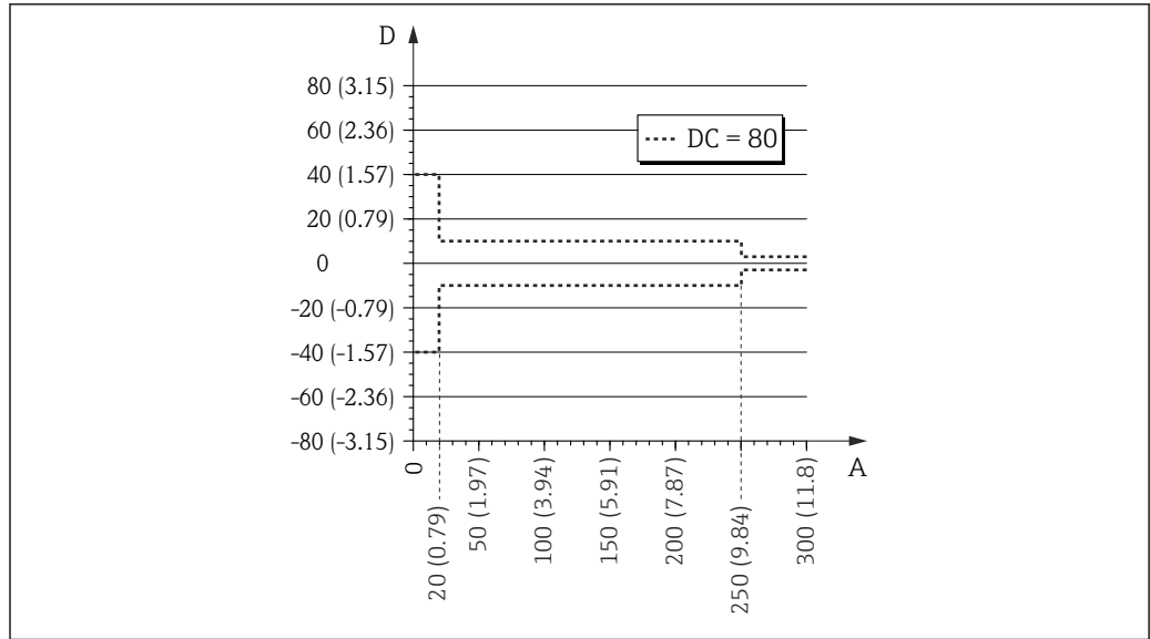
14 缆式探头末端出现的测量误差
