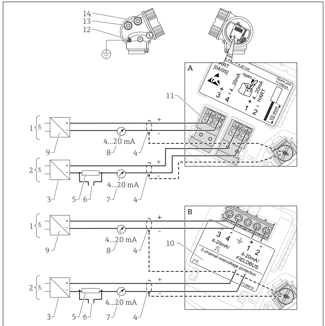
图 6 两线制连接的接线端子分配示意图; 4...20 mA HART, 4...20 mA
