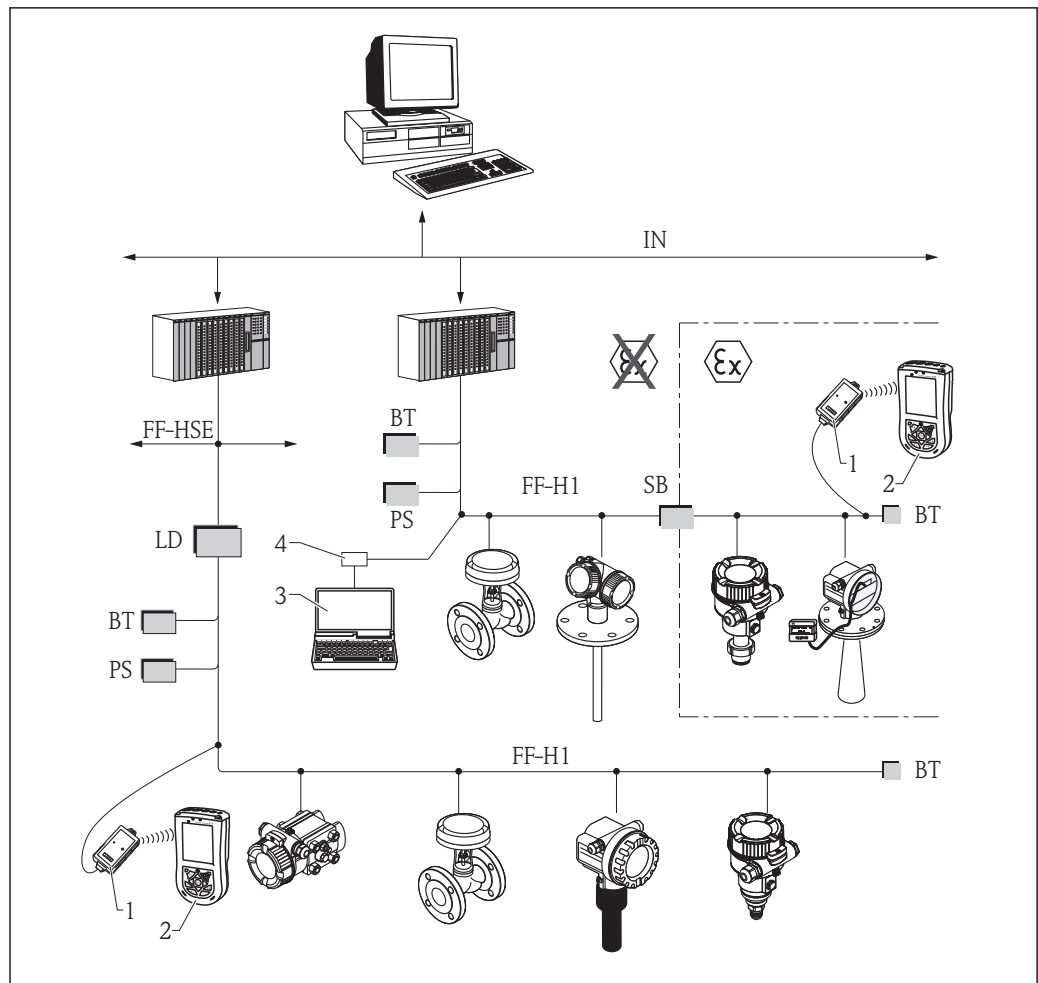
图 35 基金会现场总线(FF)系统架构及其相关部件
