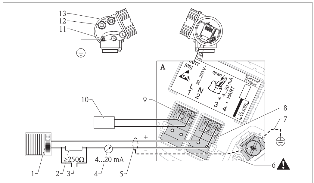
图 8 四线制连接的接线端子分配示意图; 4...20 mA HART (90...253 V AC )
