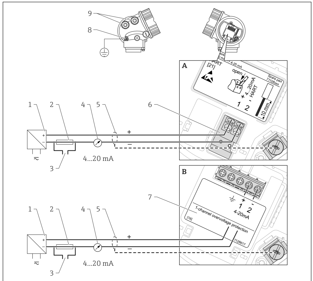
图 4 两线制连接的接线端子分配示意图; 4...20 mA HART
