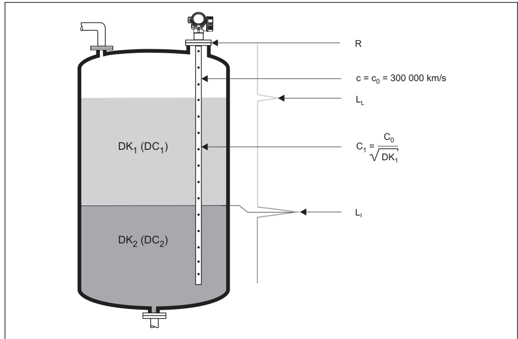
图 2 使用导波雷达进行界面测量
