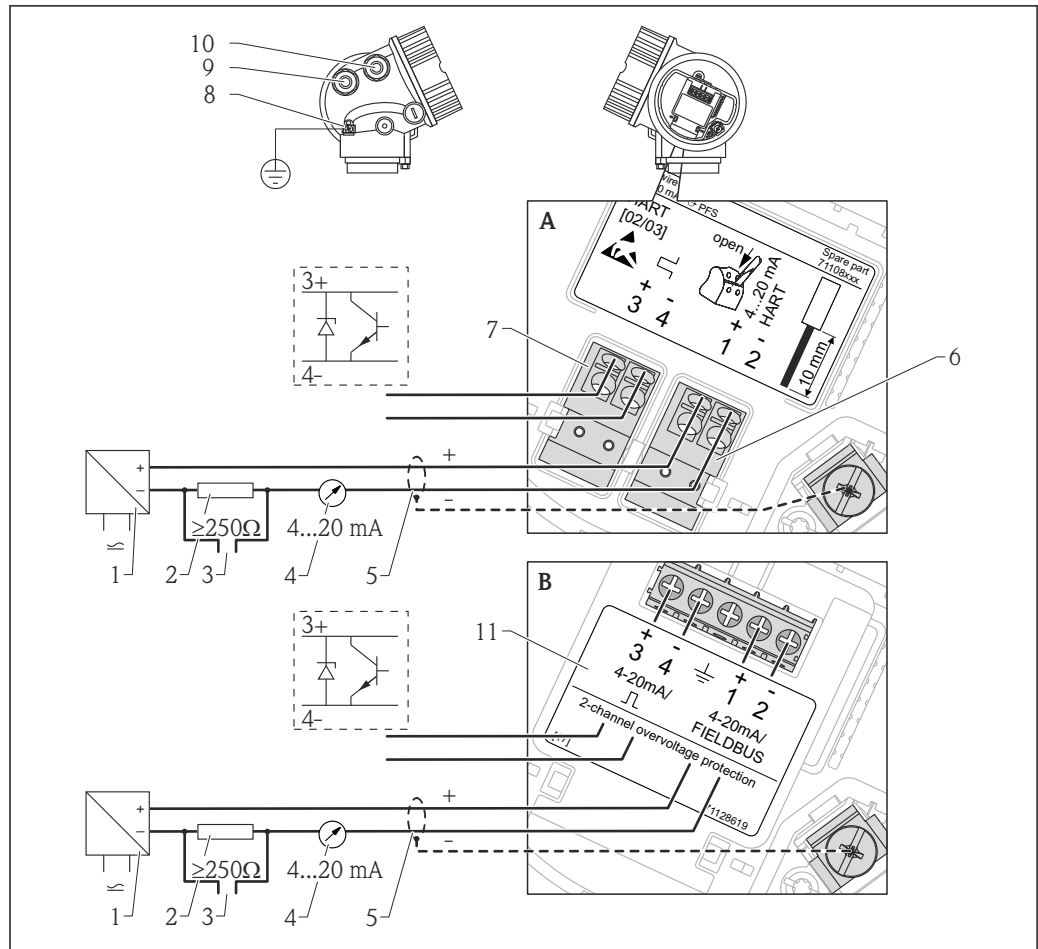
图 5 两线制连接的接线端子分配示意图; 4...20 mA HART, 开关量输出
