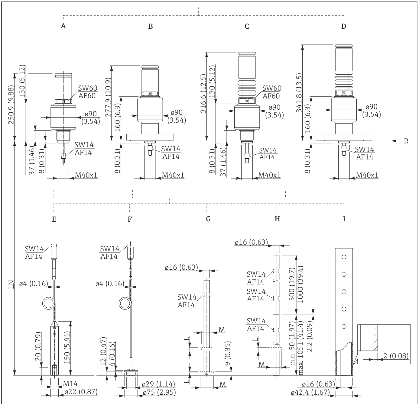
32 FMP54: 过程连接/探头; 单位: mm (in)。测量单位 mm (in)
