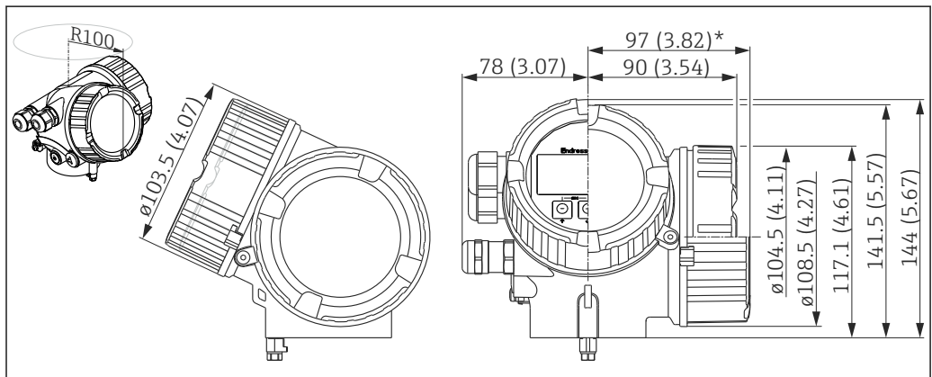
图 26 GT20 外壳(铝, 带涂层); 单位: mm (in)
