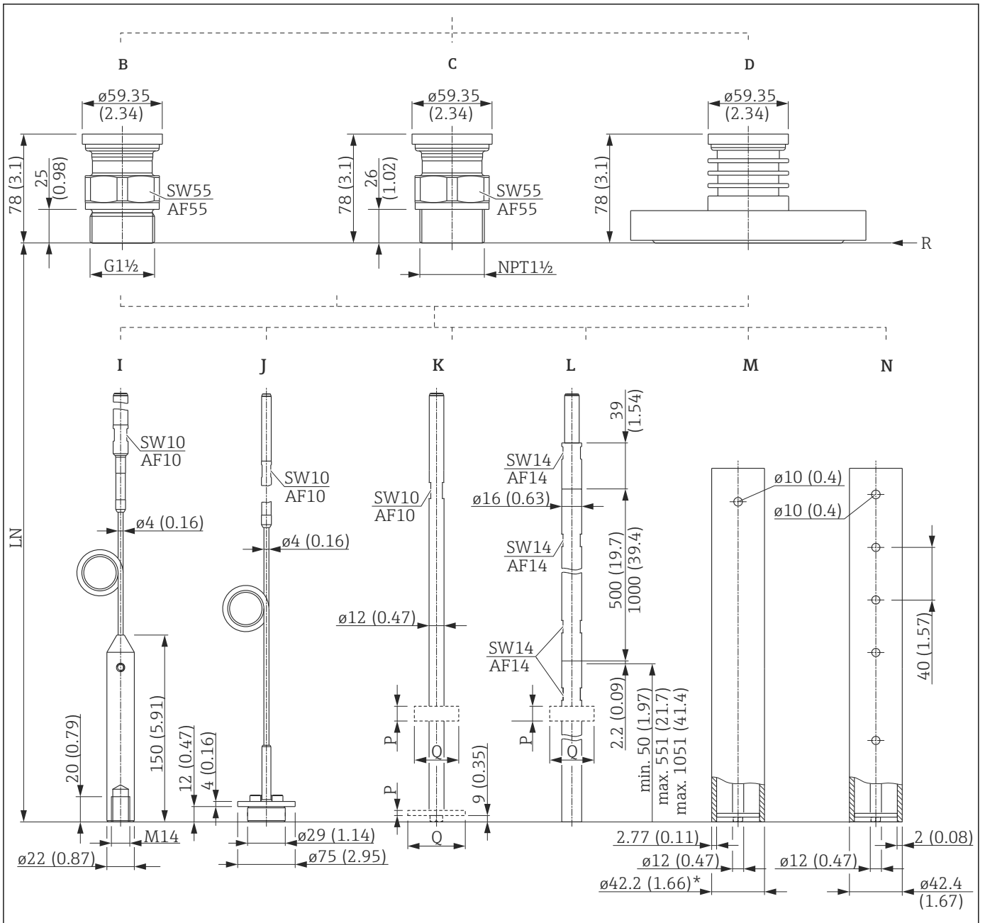
30 FMP51: 过程连接/探头; 单位: mm (in)。测量单位 mm (in)
