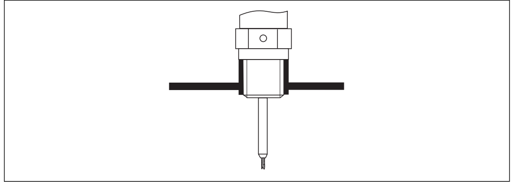
图 18 带螺纹连接的仪表安装示意图；与容器顶齐平安装
