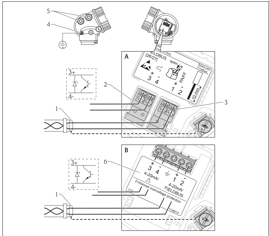
图 9 PROFIBUS PA / 基金会现场总线(FF)的接线端子分配示意图
