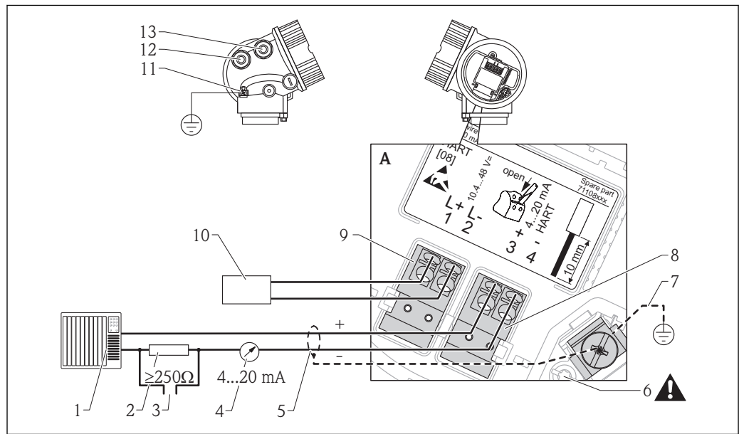
图 7 四线制连接的接线端子分配示意图; 4...20 mA HART (10.4...48 V DC)
