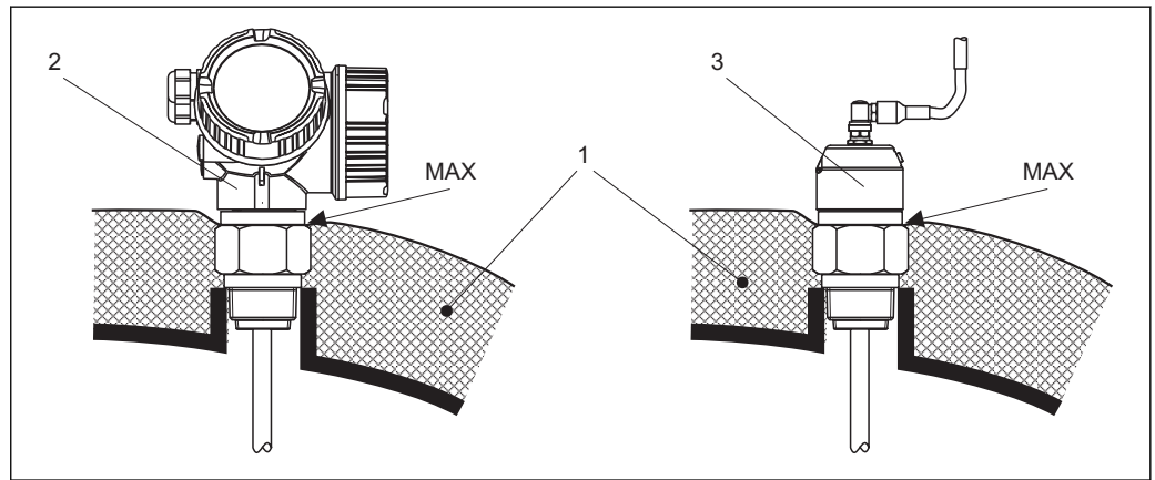
20 螺纹过程连接- FMP51
