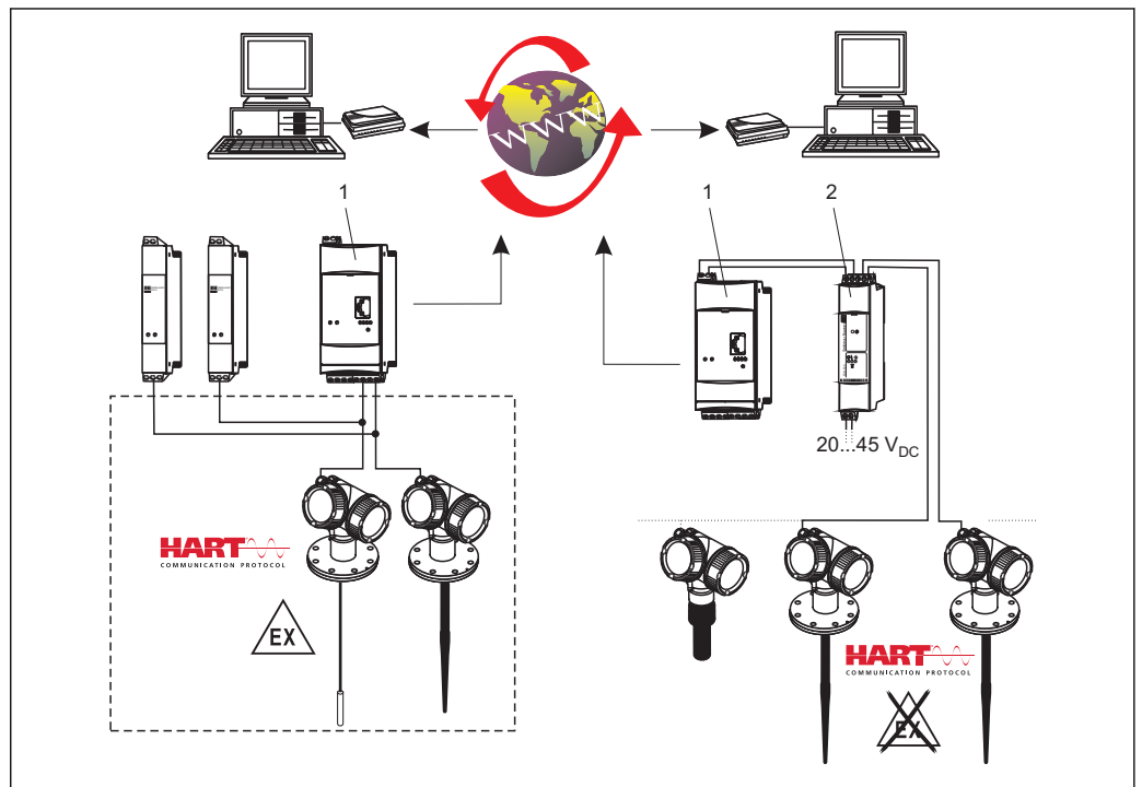
图 37 完整的测量系统包括：
