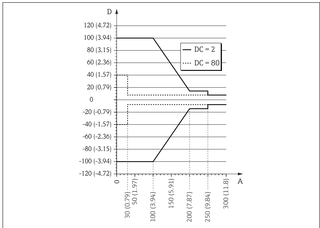
15 带金属对中盘的探头末端出现的测量误差(产品选型表的订购选项 610 “安装附件”, 选型代号 OA、OB 或 OC)
