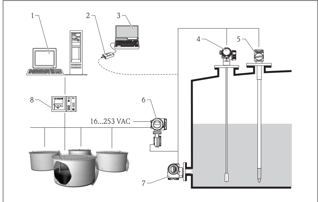
图 36 完整的测量系统包括：
