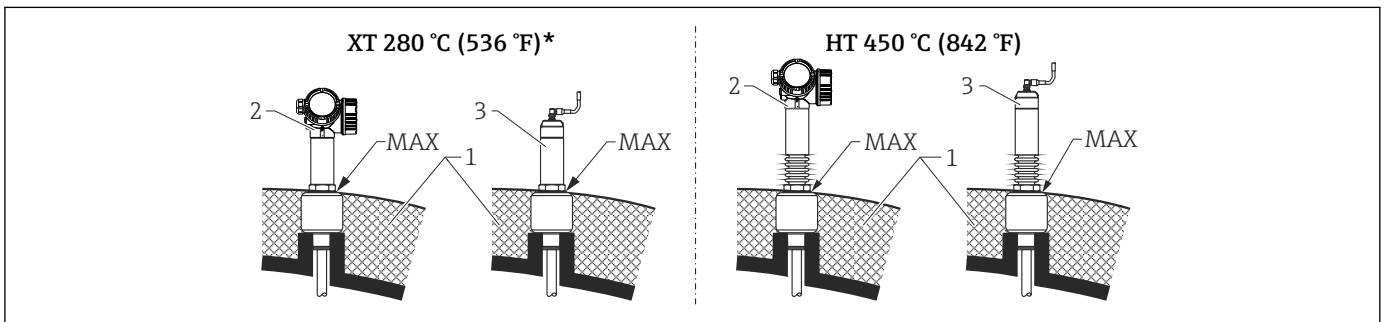
22 螺纹过程连接- FMP54, 增温型(XT)和高温型(HT)传感器
