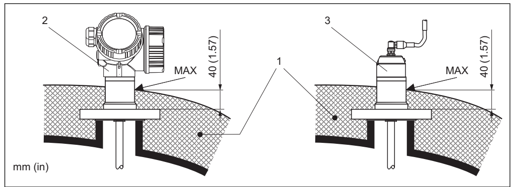
21 法兰过程连接- FMP51、FMP52
