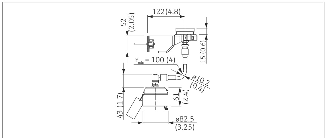
图 28 连接部分的外形尺寸，适用于分体式探头；单位：mm (in)；连接电缆的长度：订购
