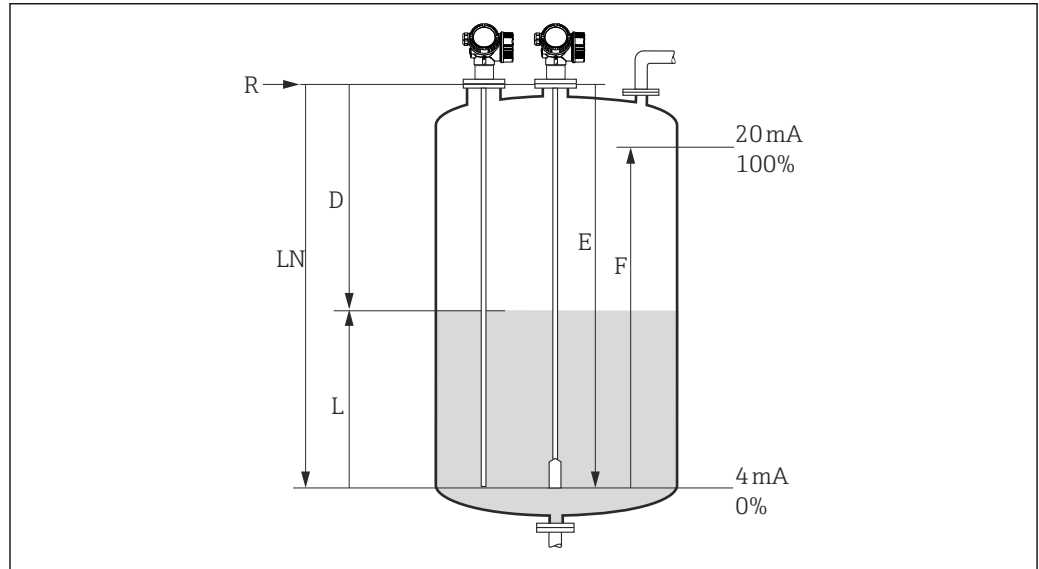
图 1 使用导波雷达进行液位测量的参数
