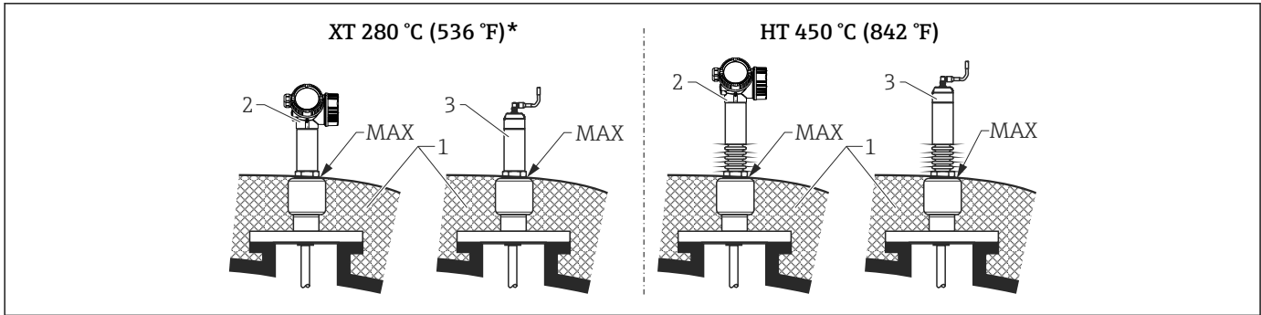
图 23 法兰过程连接- FMP54, 增温型(XT)和高温型(HT)传感器
