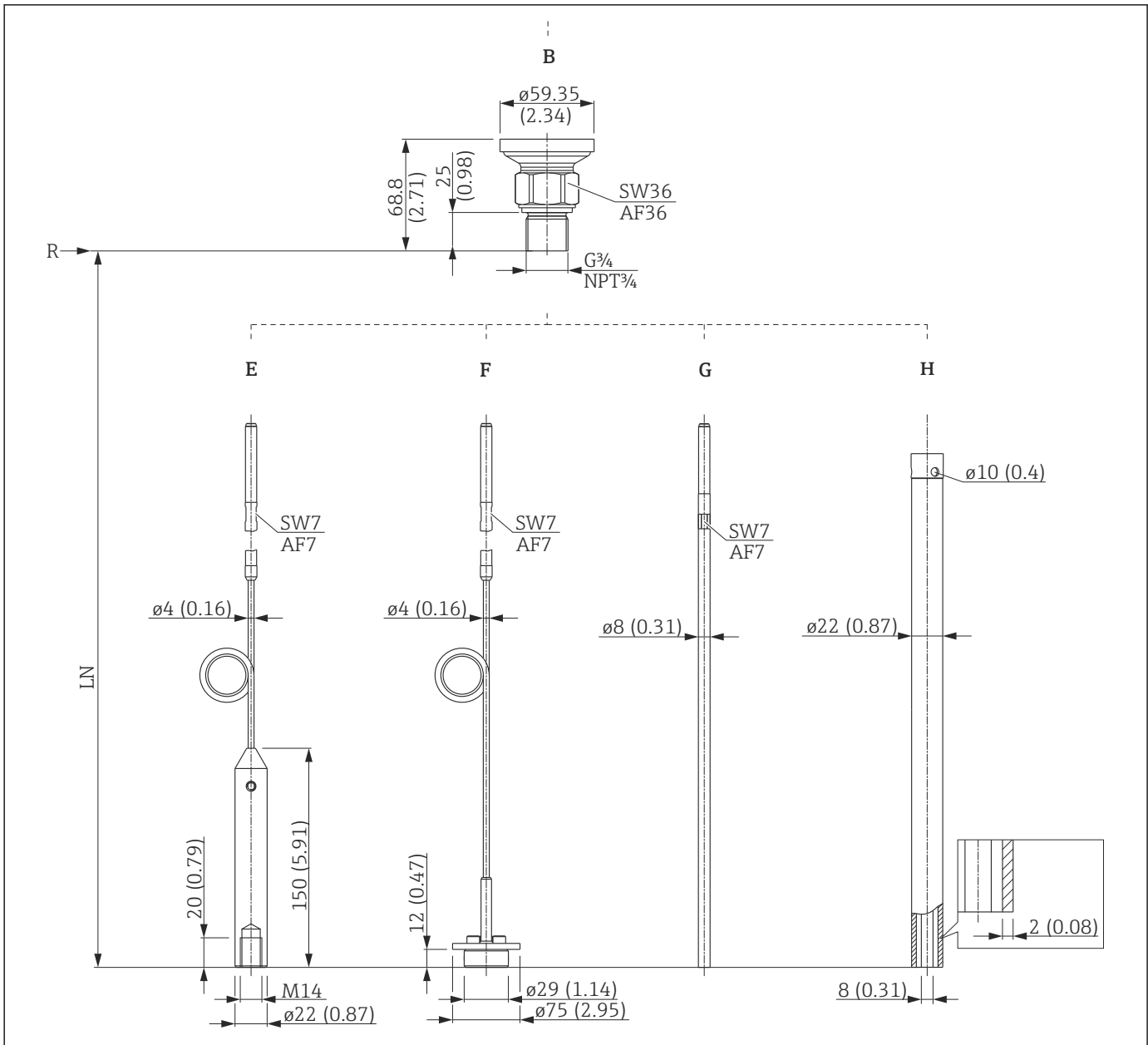
图 29 FMP51: 过程连接/探头; 单位: mm (in)。测量单位 mm (in)
