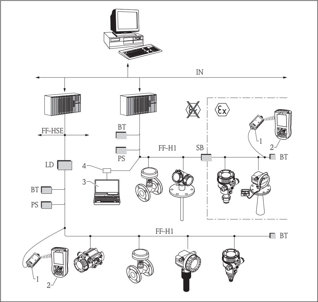
31 基金会现场总线(FF)系统架构及其相关部件
