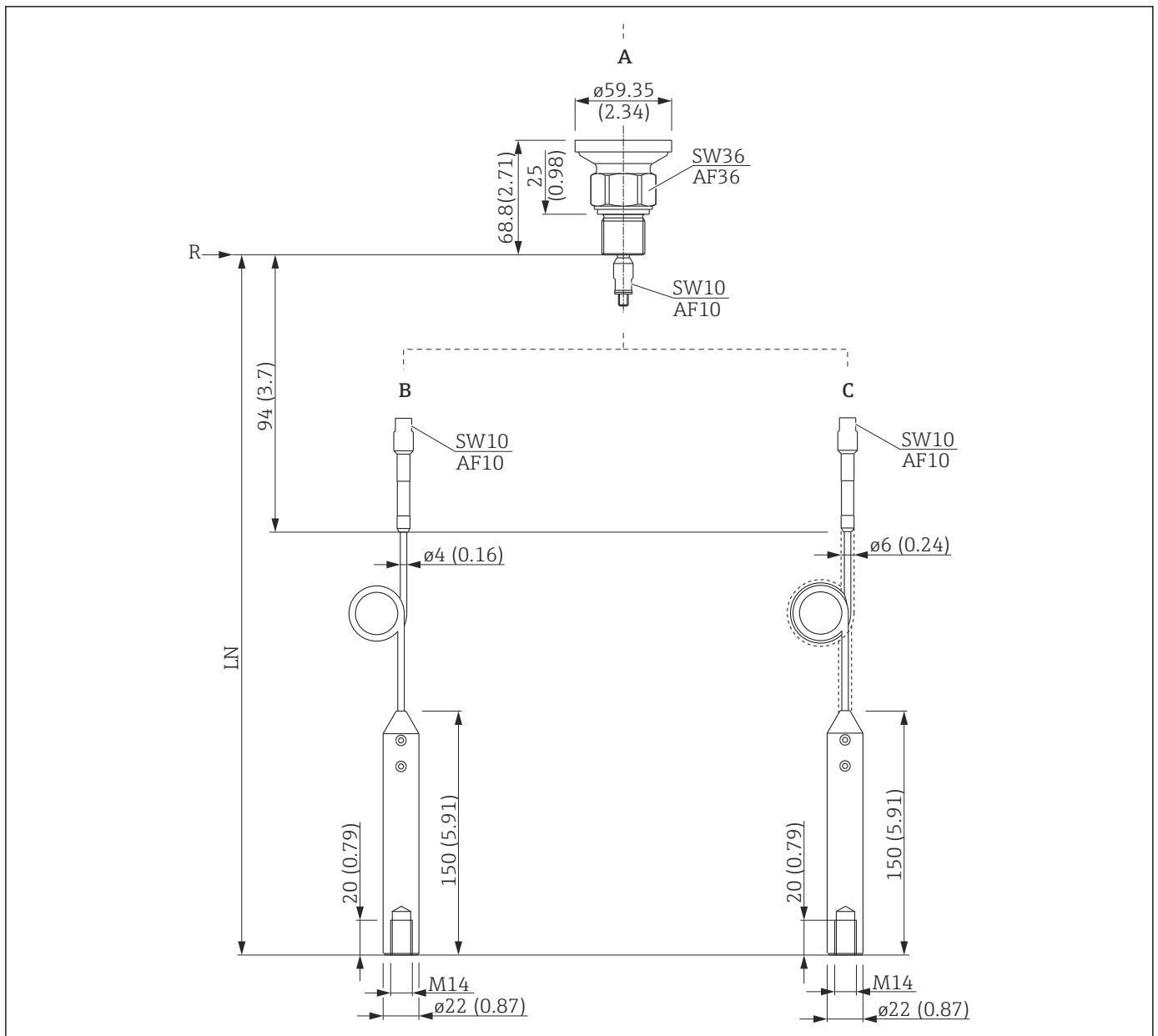
图 27 FMP56: 过程连接/探头。测量单位 mm (in)
