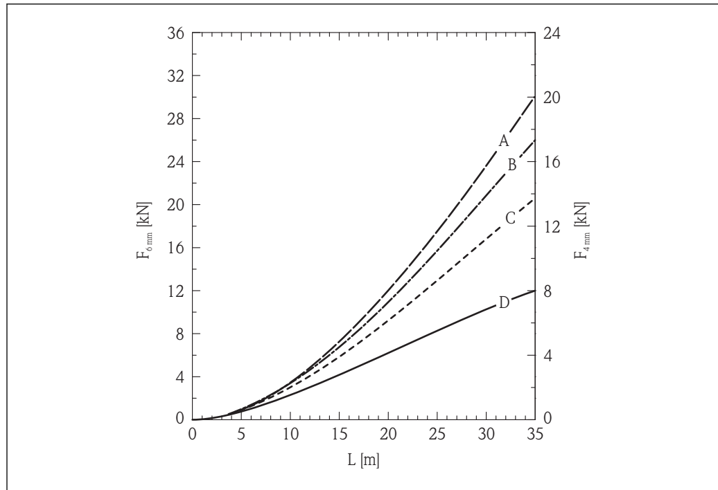
图 17 张力负载 - 物位(L)关系曲线图; 6 mm (0.24 in)和 4 mm (0.16 in)缆式探头, 小麦料仓; 光滑金属壁
