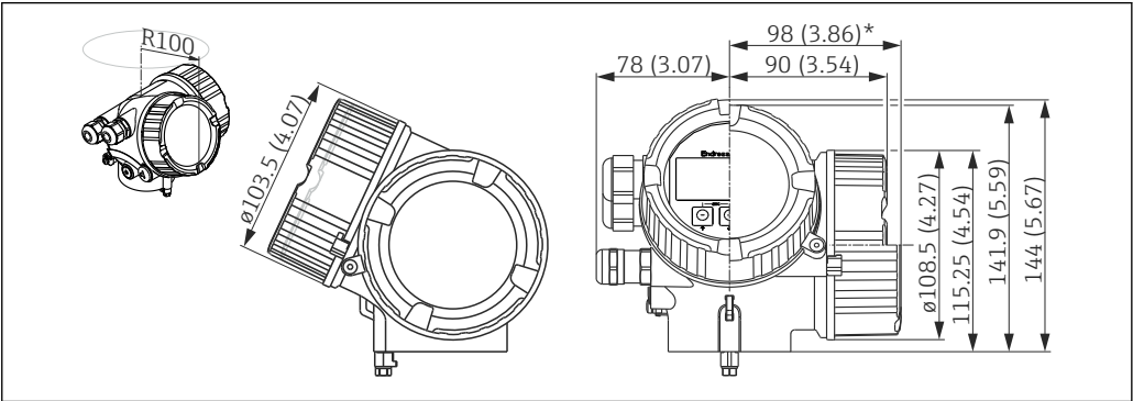
22 GT18 外壳(316L); 单位: mm (in)
