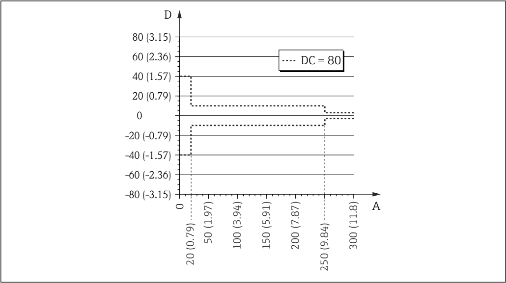
图 12 缆式探头末端出现的测量误差
