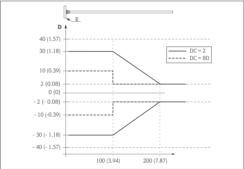
图 13 缆式探头末端出现的测量误差，单位：mm (in)
