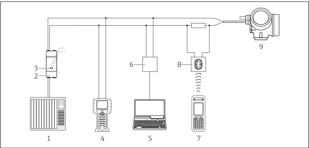
图 30 通过 HART 通信进行远程操作
