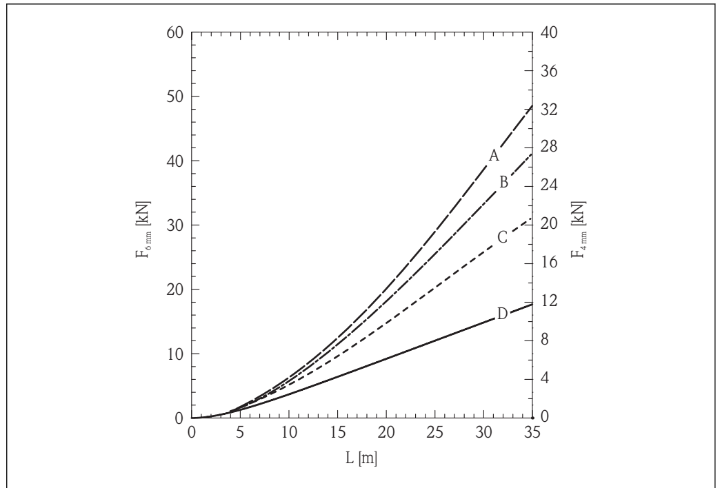
15 张力负载 - 物位(L)关系曲线图; 6 mm (0.24 in)和 4 mm (0.16 in)缆式探头, 石英砂料仓; 光滑金属壁
