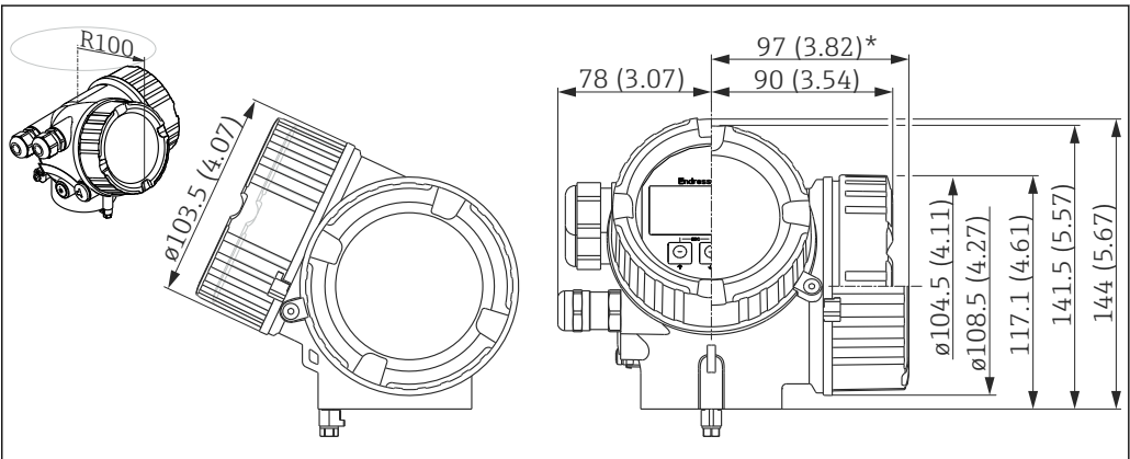
24 GT20 外壳(铝, 带涂层); 单位: mm (in)
