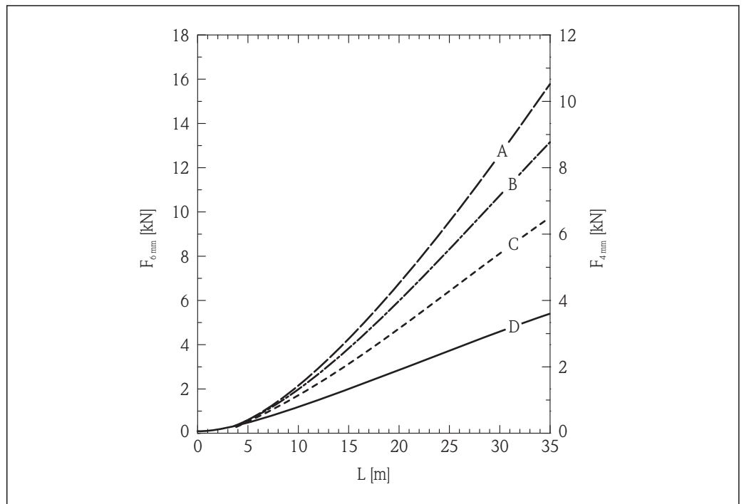
16 张力负载 - 物位(L)关系曲线图; 6 mm (0.24 in)和 4 mm (0.16 in)缆式探头, 聚乙烯粒子料仓; 光滑金属壁
