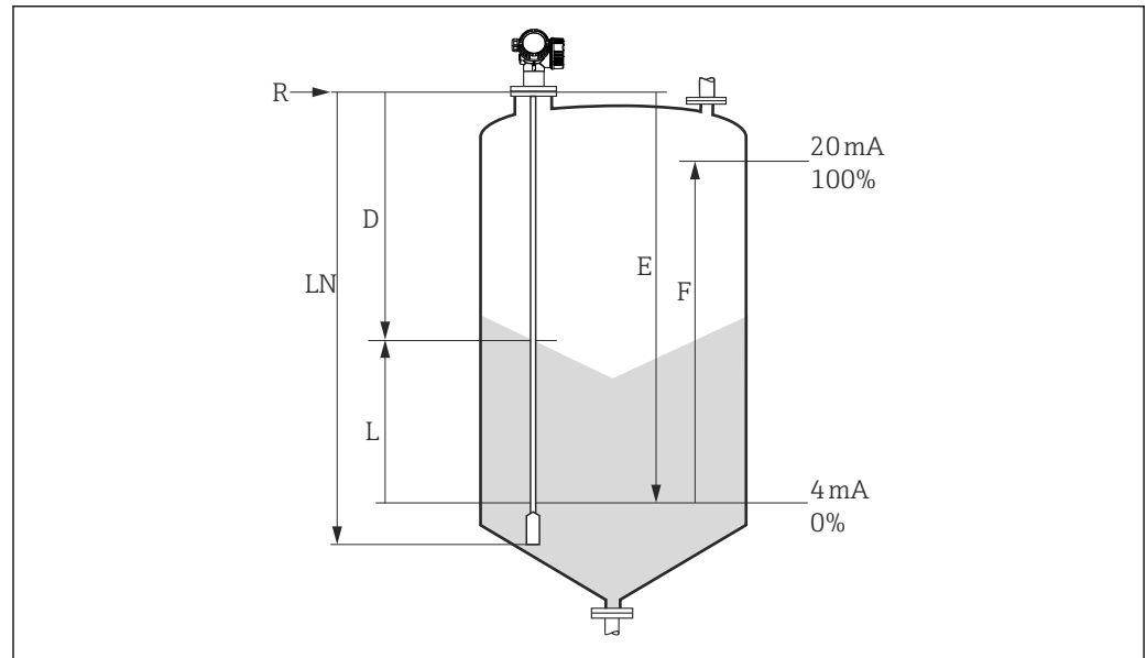
图 1 使用导波雷达进行液位测量的参数
