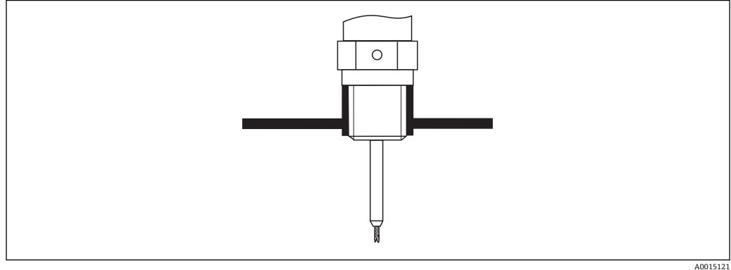
图 19 带螺纹连接的仪表安装示意图；与容器顶齐平安装
