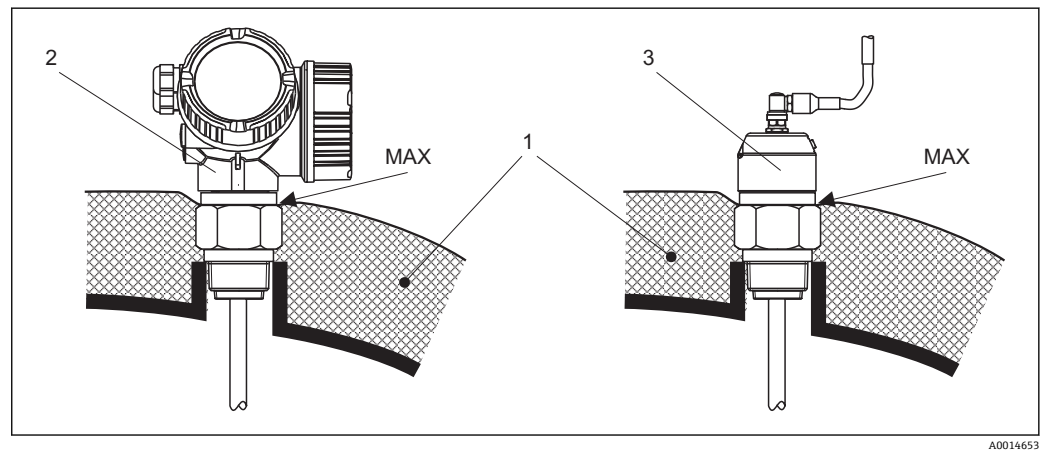
20 螺纹过程连接- FMP56、FMP57
