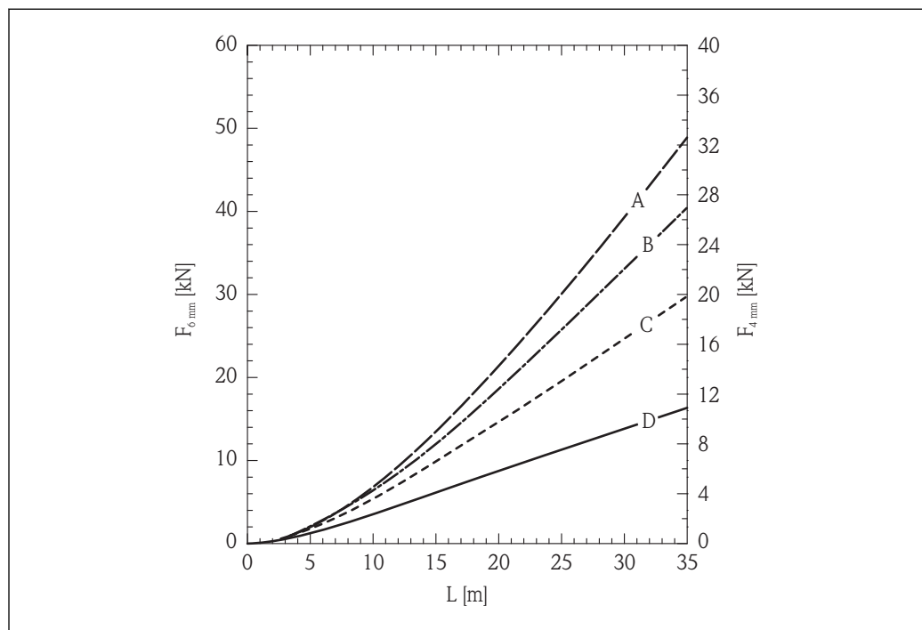
图 18 张力负载 - 物位(L)关系曲线图; 6 mm (0.24 in)和 4 mm (0.16 in)缆式探头, 水泥料仓; 光滑金属壁
