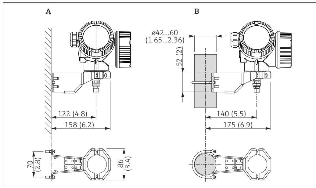
图 25 电子腔外壳的安装支架示意图，单位：mm (in)
