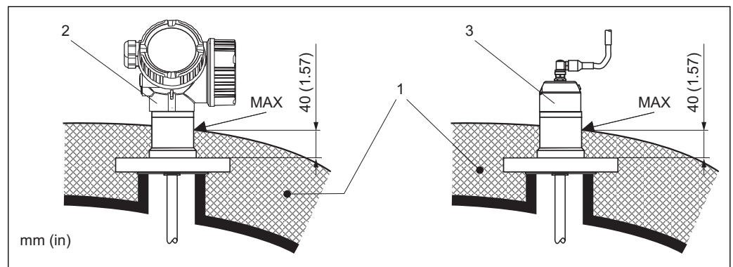
21 法兰过程连接- FMP57
