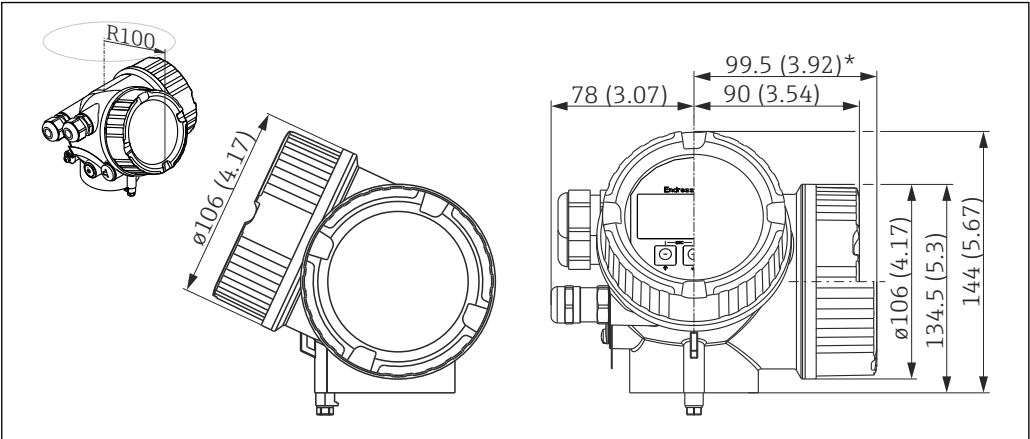
23 GT19 外壳(塑料 PBT); 单位: mm (in)
