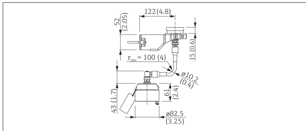
图 26 连接部分的外形尺寸，适用于分体式探头；单位：mm (in)；连接电缆的长度：订购
