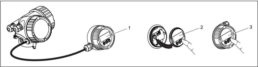
图 29 FHX50 的操作选项
