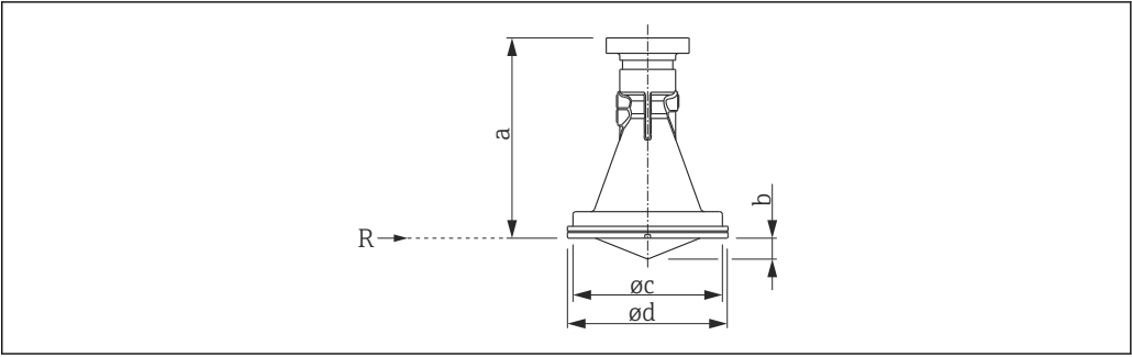
23 不带过程连接的 FMR56 的示意图；外形尺寸单位：mm (in)
