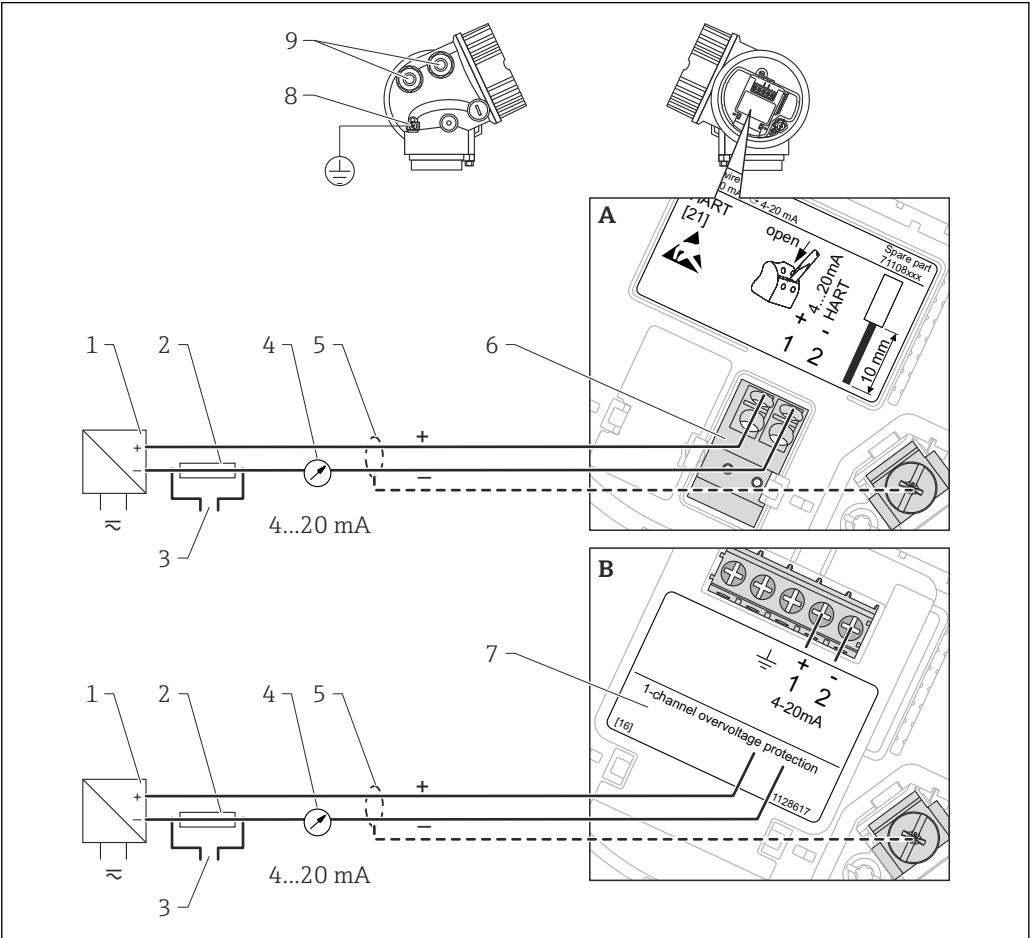
2 两线制连接的接线端子分配示意图; 4...20 mA HART
