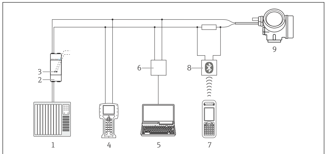
图 32 通过 HART 通信进行远程操作
