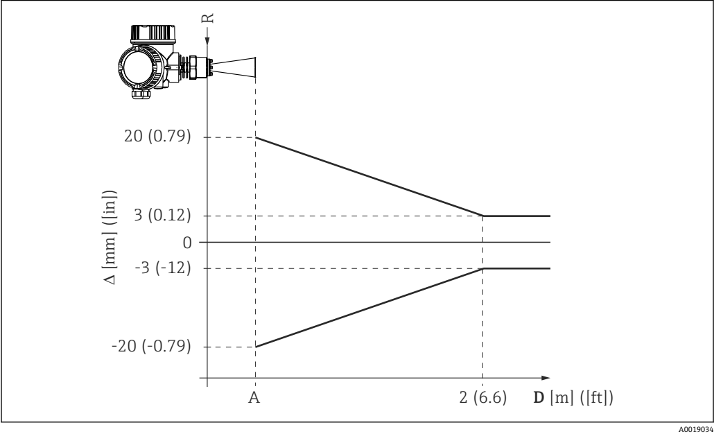
图 10 近距离测量时的最大测量误差示意图
