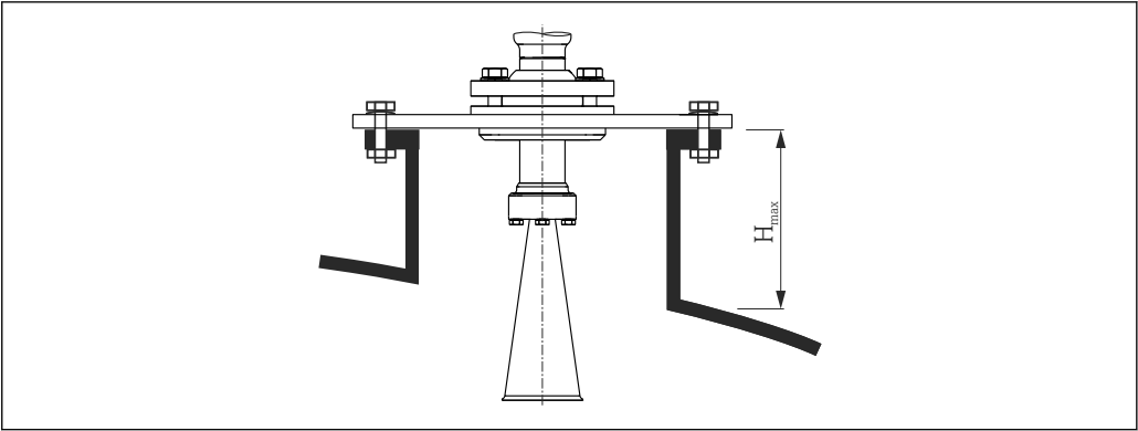
14 喇叭天线的安装短管高度(FMR57)
