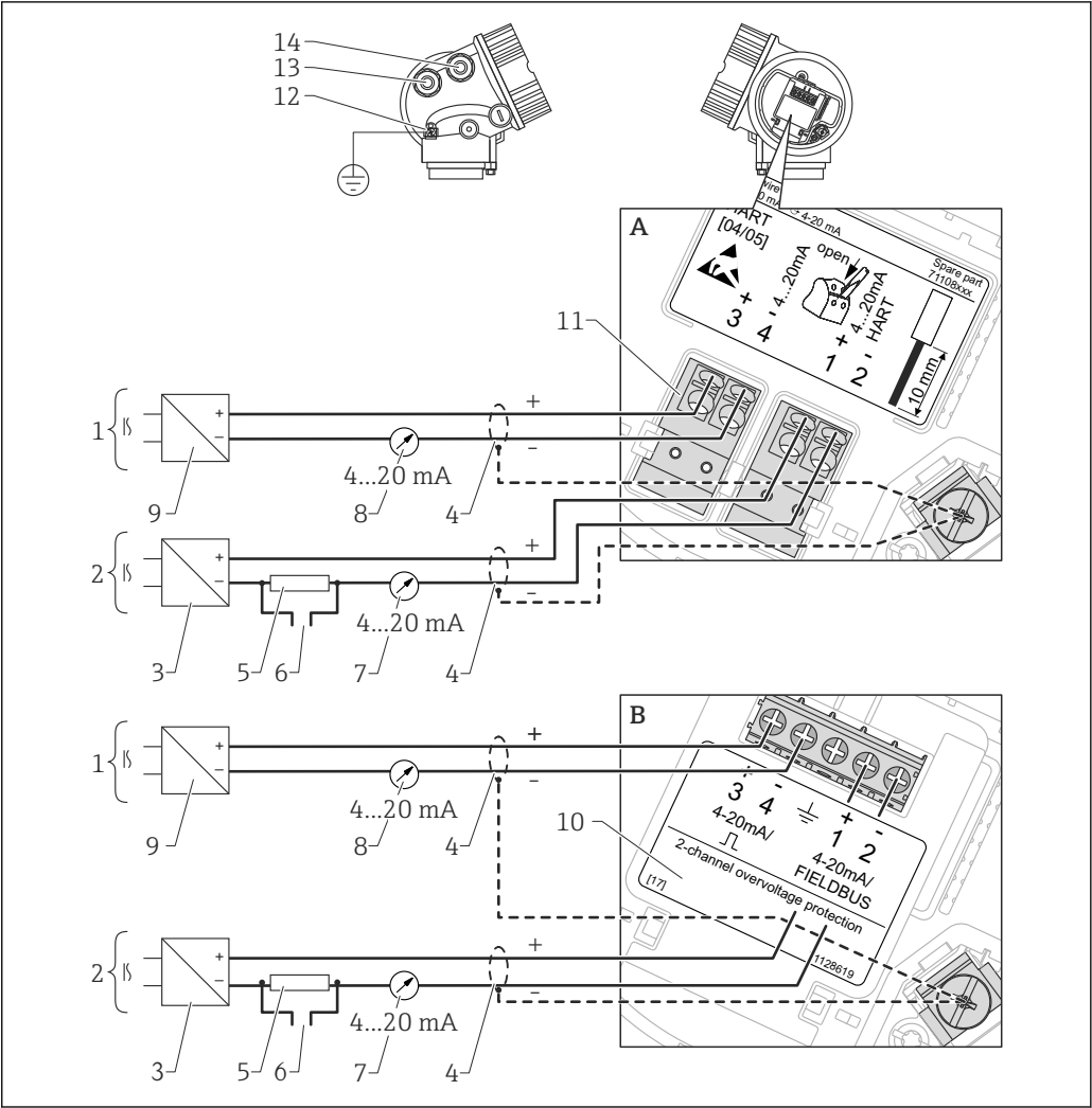
4 两线制连接的接线端子分配示意图; 4...20 mA HART, 4...20 mA
