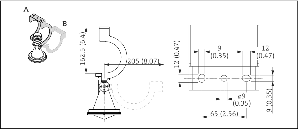
24 FMR50/FMR56 的安装支架外形尺寸示意图；单位：mm (in)
