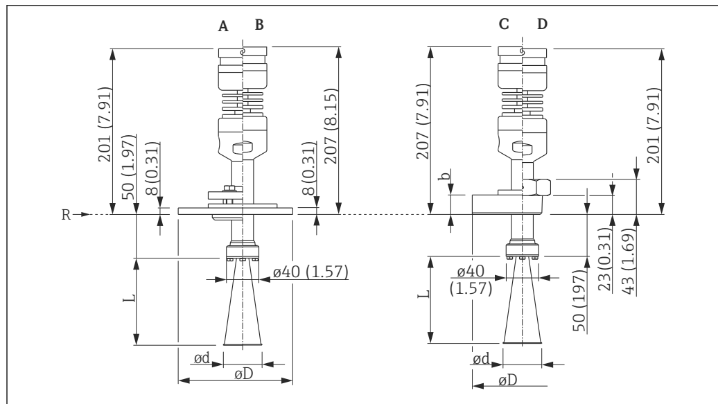
图 29 带喇叭天线的 FMR57 (高温型)的外形尺寸示意图; 外形尺寸单位: mm(in)
