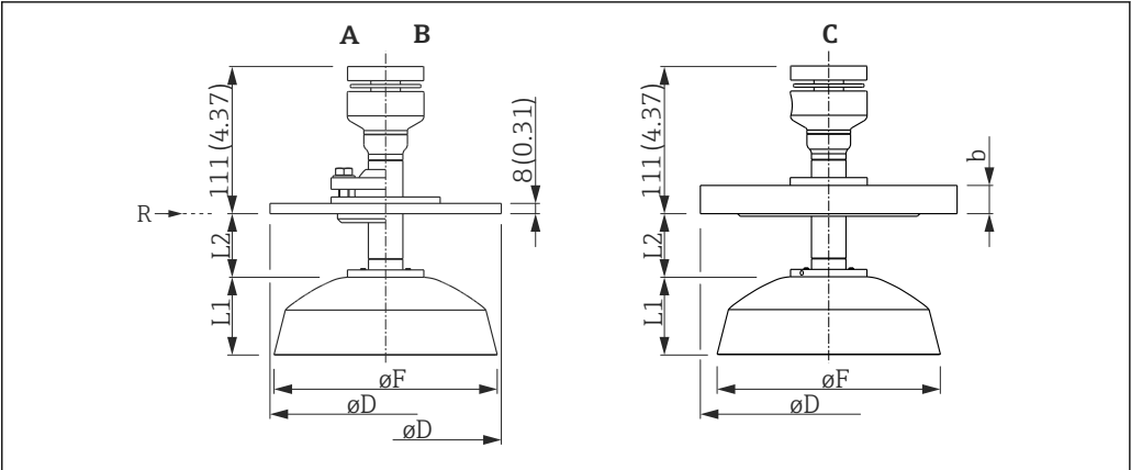
30 带抛物面天线的 FMR57 的外形尺寸示意图；外形尺寸单位：mm (in)
