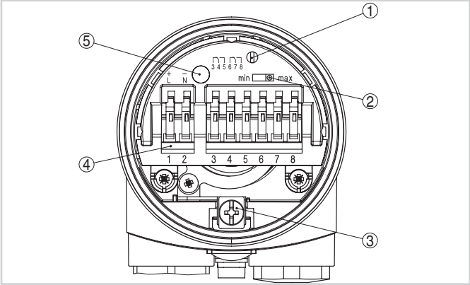
电子部件腔和接线腔 - 继电器输出口
