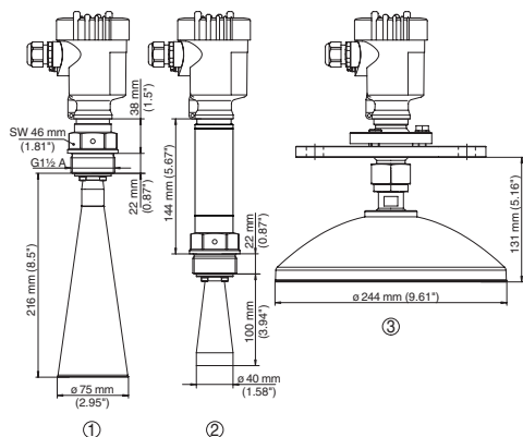
VEGAPULS 68 的尺寸
