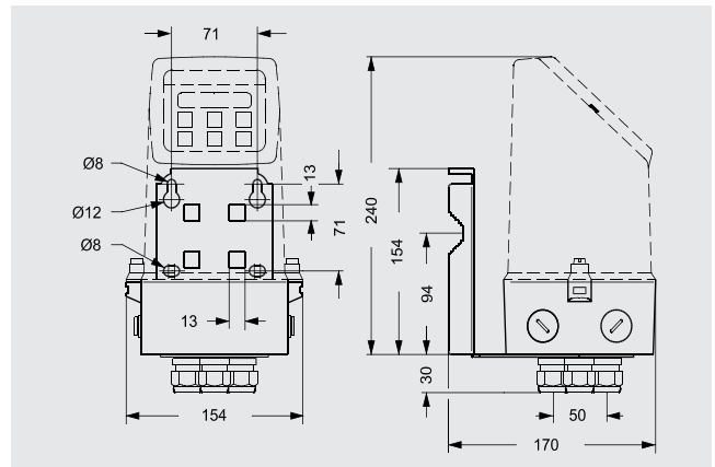
变送器墙装
