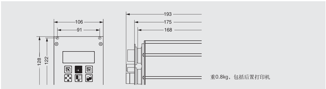
变送器墙装
