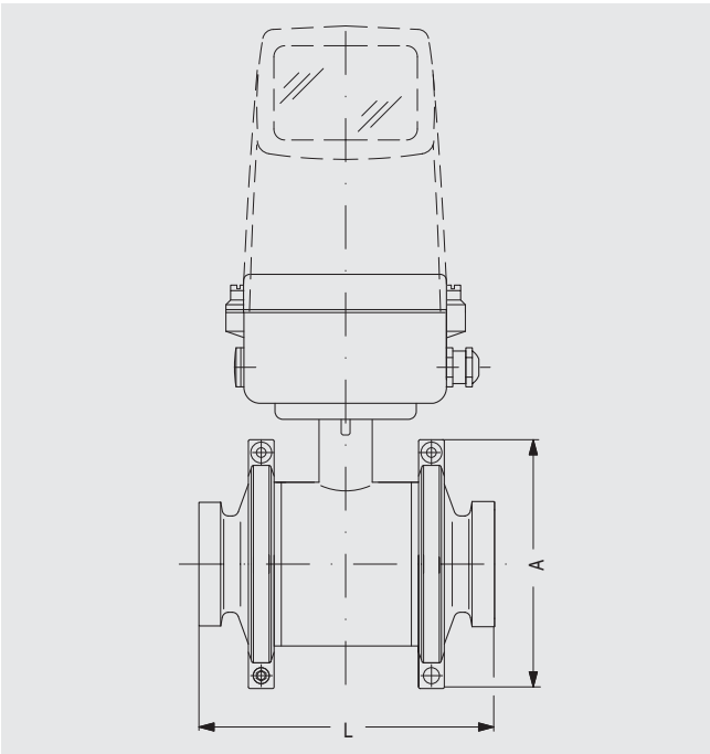
MAG 1100 Food 传感器一体式 / 分体式 - 嵌入长度
