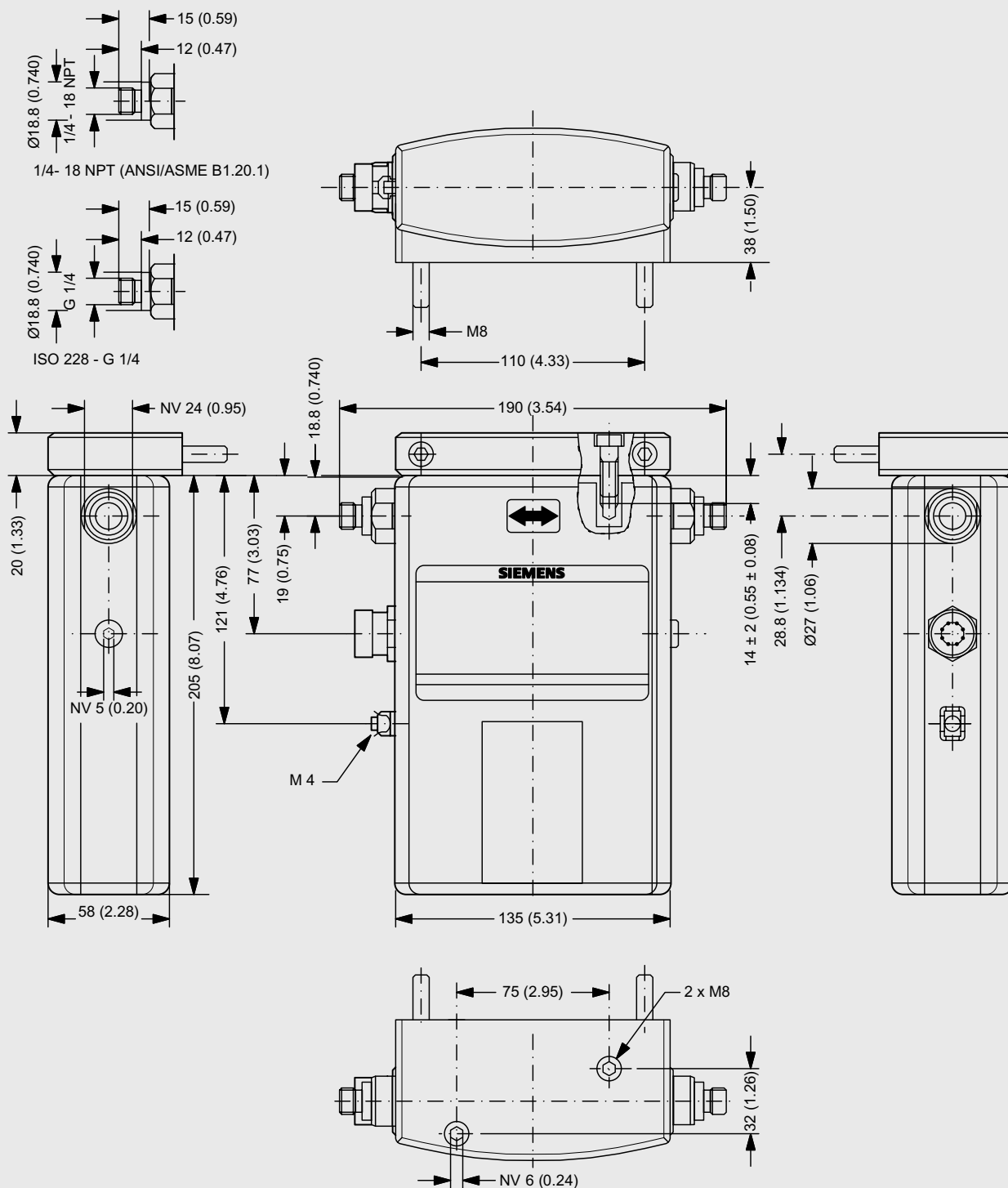
SITRANS FC300 尺寸图，单位 mm (inch)
