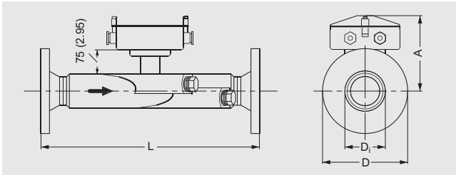
传感器 SONO 3300
